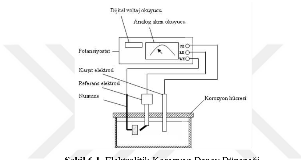
Şekil 6.1. Elektrolitik Korozyon Deney Düzenegi.
