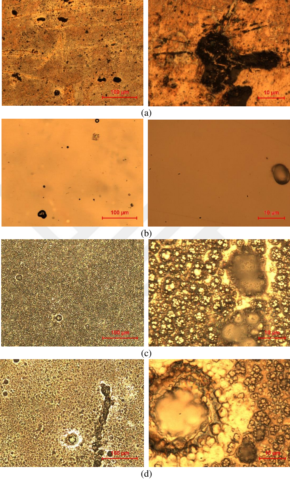
Şekil 7.6. Düşük (200X) ve Yüksek (1500X) Büyütmelerde (a) Be-Cu Alaşımı, (b) Ni-P, (c) Ni-B ve (d) Ni-P/Ni-B Kaplamaların Korozyon Deneyi Sonrası Yüzey Görüntüleri.
