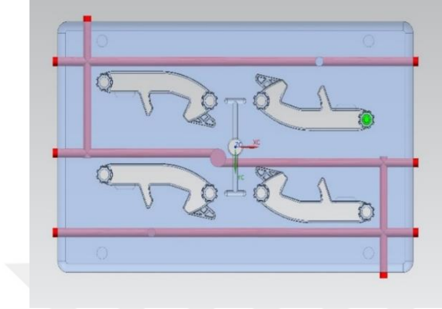
Şekil 3.12. PSR parçasına ait kalıpta soğutma kanalları
