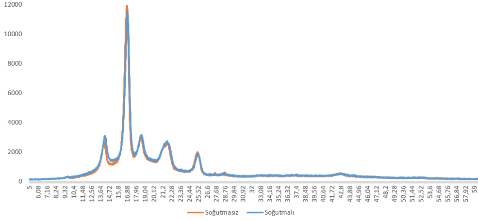
Şekil 5.2. PSR parçasının kulak kısmından alınan kesitlerin XRD analiz grafiği
