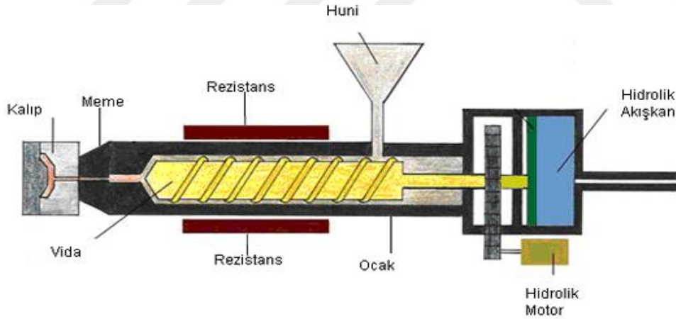
Şekil 3.2. Vida bölümleri
