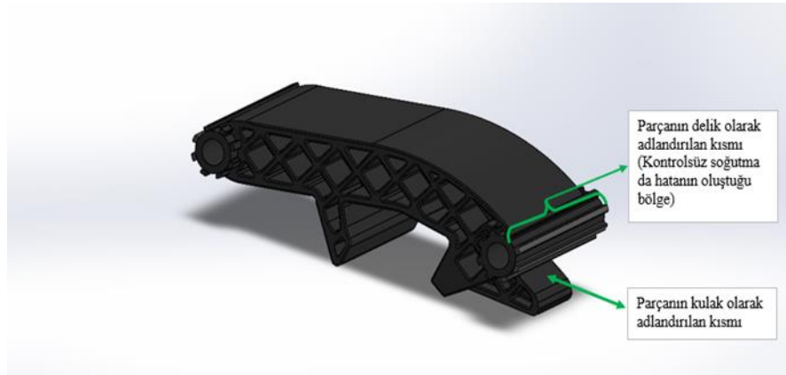
Şekil 5.1. PSR parçasında XRD analizi yapılan kısımların gösterimi
