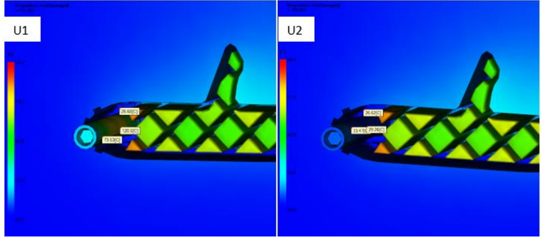
Şekil 5.6. Yavaş ve hızlı soğutmada parça yüzey sıcaklıkları
