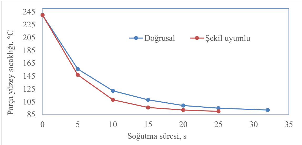
Şekil 5.10. Plastik parçaların çıkarma sıcaklığına erişim süreleri
