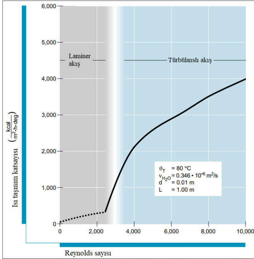
Şekil 3.27. Isı taşınım katsayısının Reynolds sayısına göre değişimi [109]
