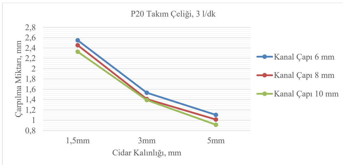
Şekil 5.21. Çarpılma miktarının cidar kalınlığına göre değişimi
