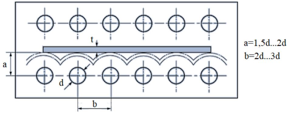
Şekil 3.19. Soğutma kanallarının konumları (a: kanal-kalıp arası mesafe, b: kanallar arası mesafe)
