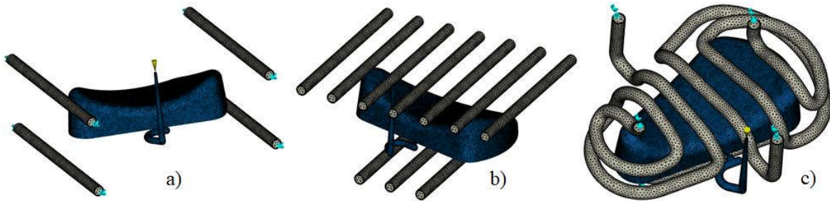
Şekil 4.21. a) Doğrusal, b) Eş hacimli doğrusal ve c) Şekil uyumlu soğutma kanalları
