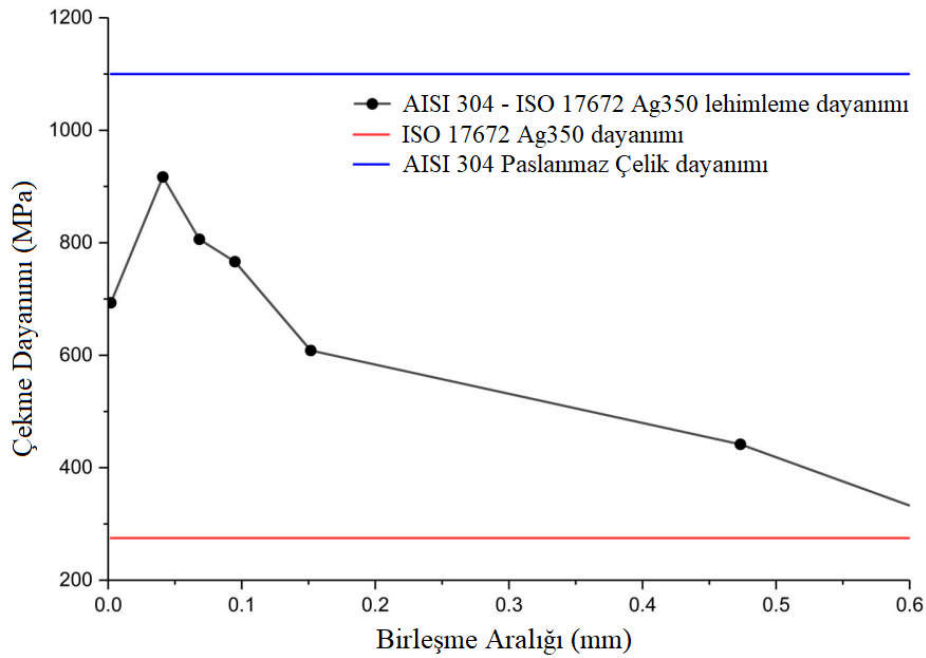
Şekil 3.29. Lehimleme aralığı-birleştirme dayanımı ilişkisi [117]
