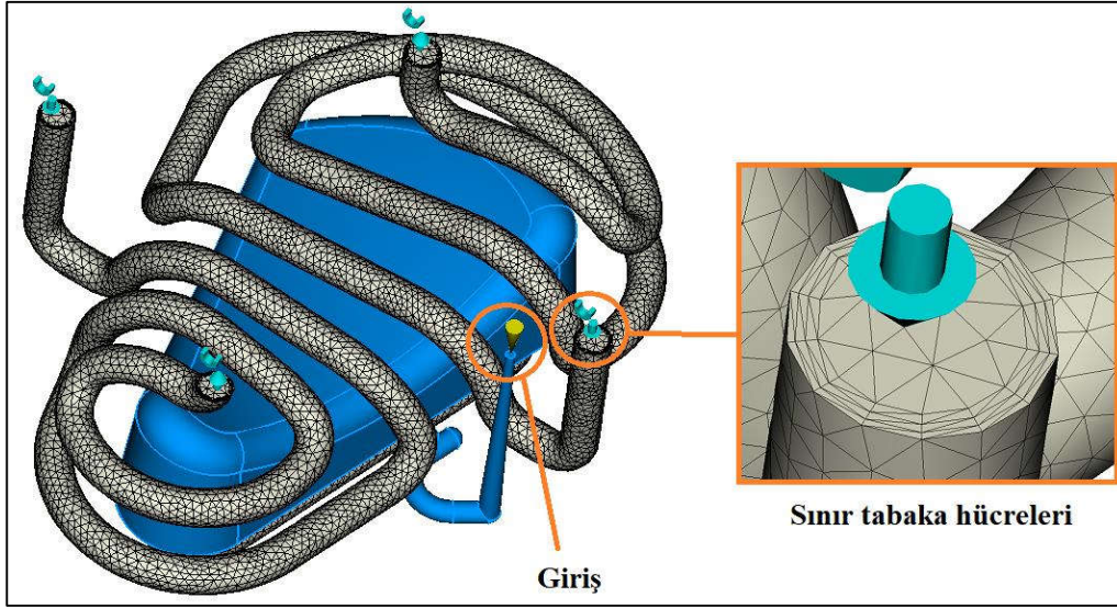
Şekil 4.23. Plastik parça üzerindeki giriş (gate) noktası
