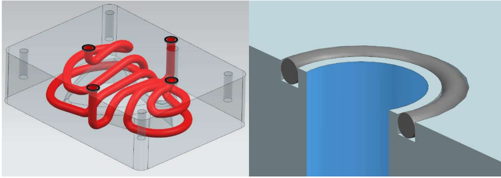
Şekil 4.18. Kanal girişlerine yerleştirilen conta
