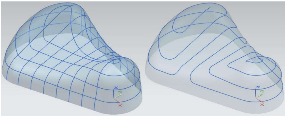
Şekil 4.9. Bağlantı eğrilerinin eklenmesi, kırpma ve yuvarlatma [69]
