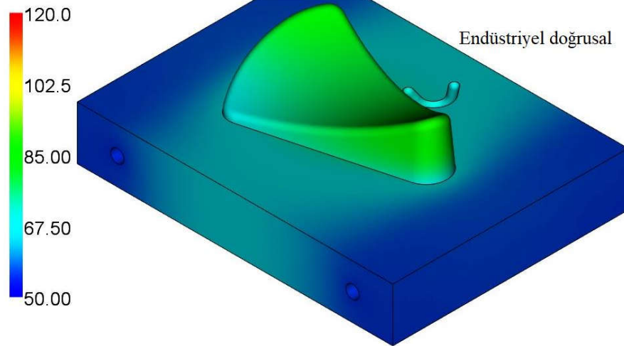
Şekil 2.1. Erkek kalıp çekirdeği üzerindeki sıcaklık dağılımları
