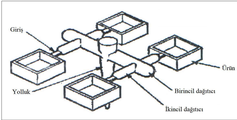
Şekil 3.6. Soğuk yolluk bileşenleri [93]
