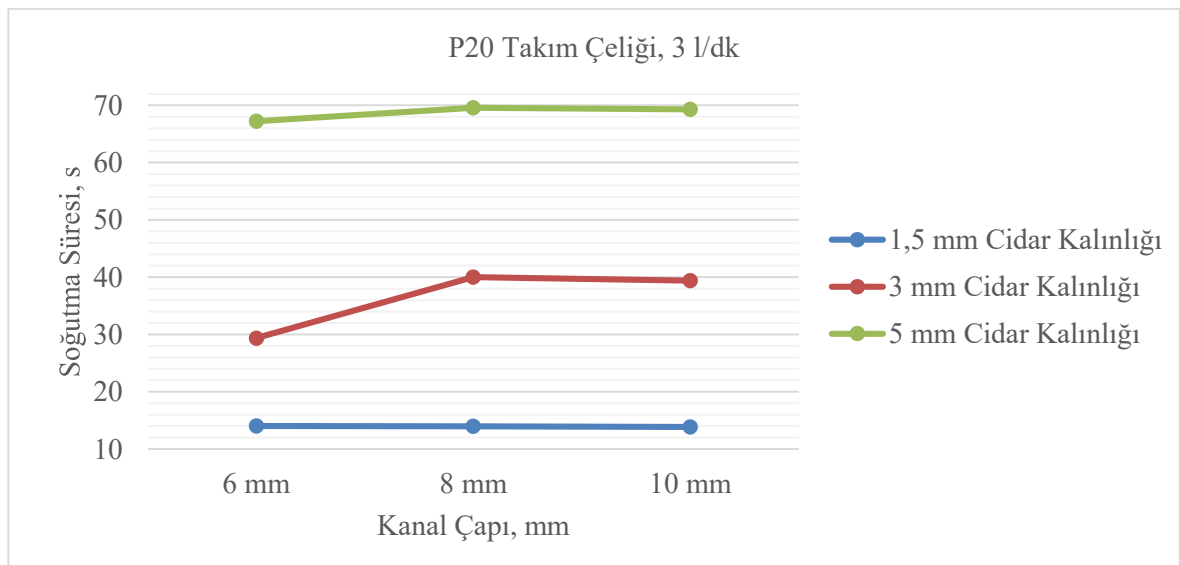
Şekil 5.18. Soğutma süresinin kanal çapına göre değişimi
