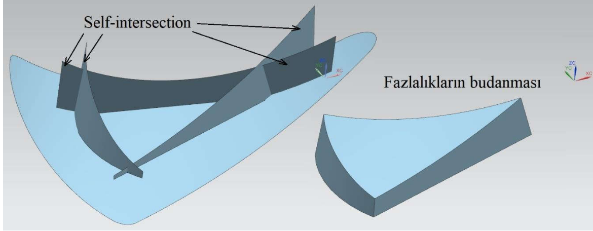
Şekil 4.4. İç yüzeyin ofsetlenmesiyle elde edilen referans yüzey
