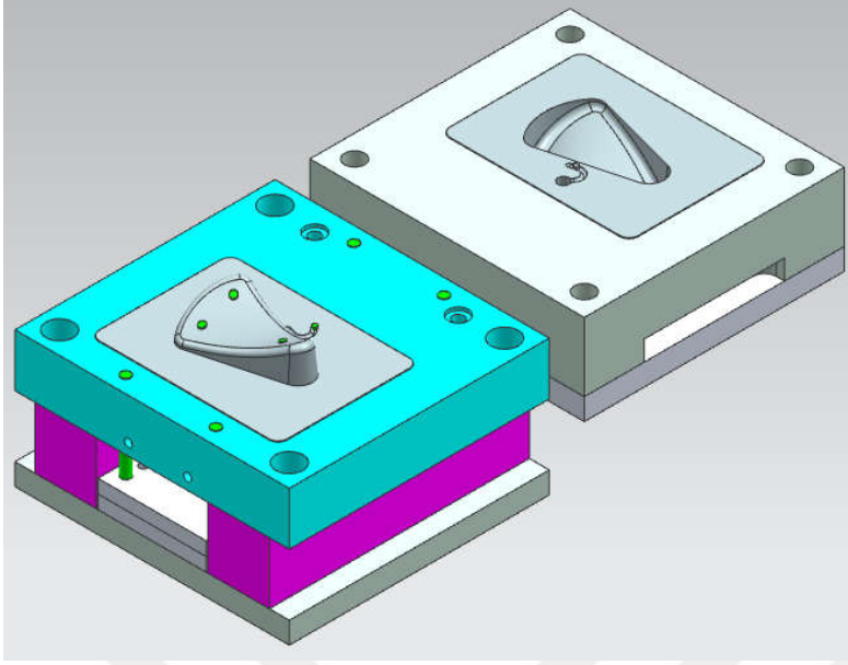
Şekil 4.17. Tek gözlü plastik enjeksiyon kalıbı tasarımı
