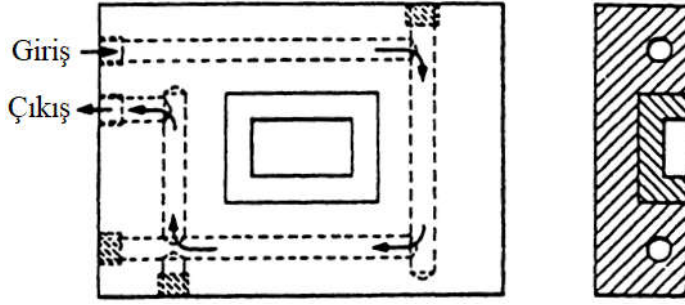
Şekil 3.21. Dişi kalıp plakasının soğutulması
