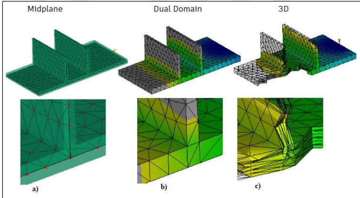
Şekil 4.22 Sayısal ağda kullanılan hücre tipleri a) Midplane, b) Dual Domain, c) 3D [125]
