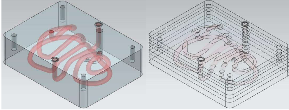
Şekil 4.19. Kalıp çekirdeğinin CAD modeli ve katmanlara ayrılması
