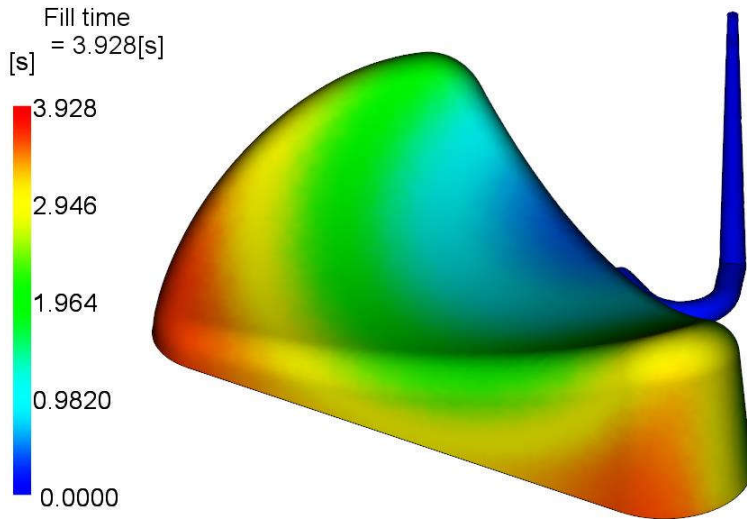
Şekil 5.3. Kalıp boşluğunun dolum süresi
