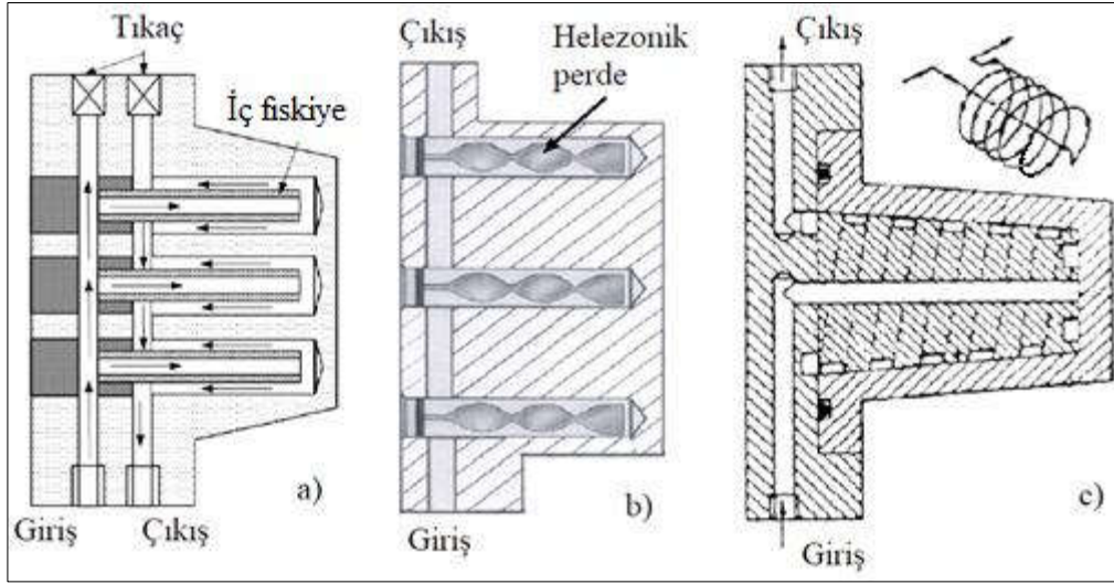
Şekil 3.24. a) İç fiskiyeli (bubbler) kanal, b) Helezonik bölmeli (baffle) kanal, c) Lokmalı helis kanal
