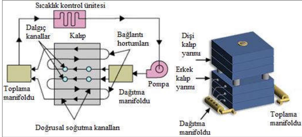
Şekil 3.18. Plastik enjeksiyon kalıplamada soğutma sistemi
