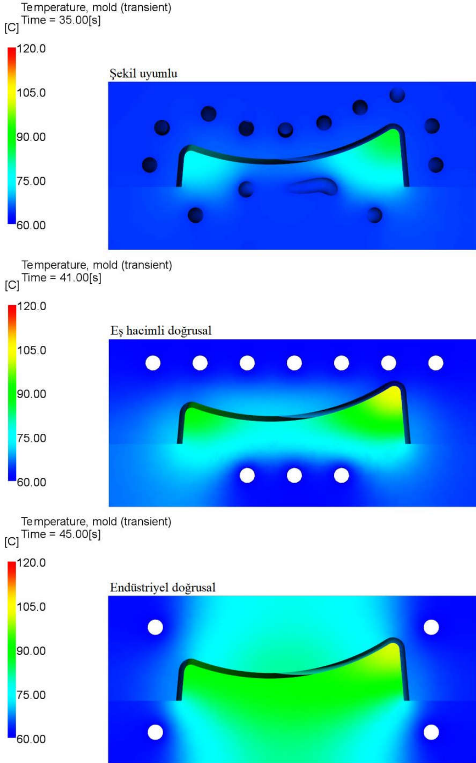
Şekil 5.5. Kalıp üzerindeki sıcaklık dağılımları
