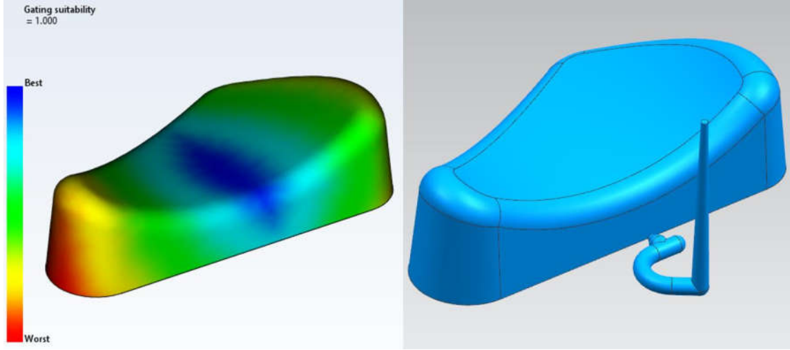
Şekil 4.15. Giriş yeri analizi ve yolluk tasarımı
