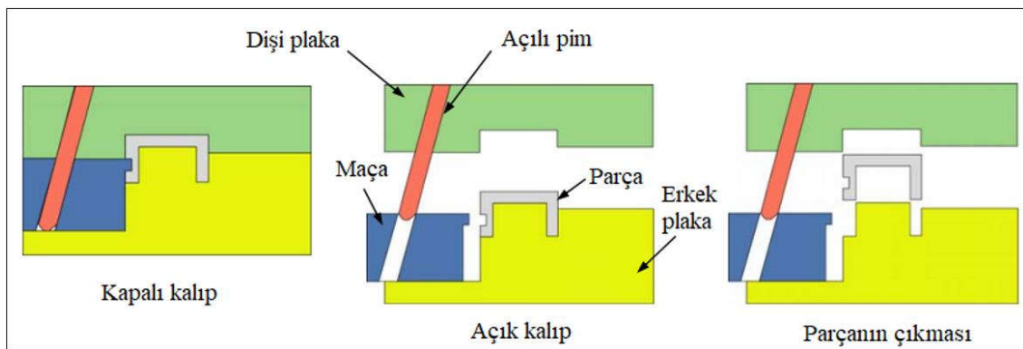
Şekil 3.12. Maça hareketi ile parçanın kalıptan çıkması [97]
