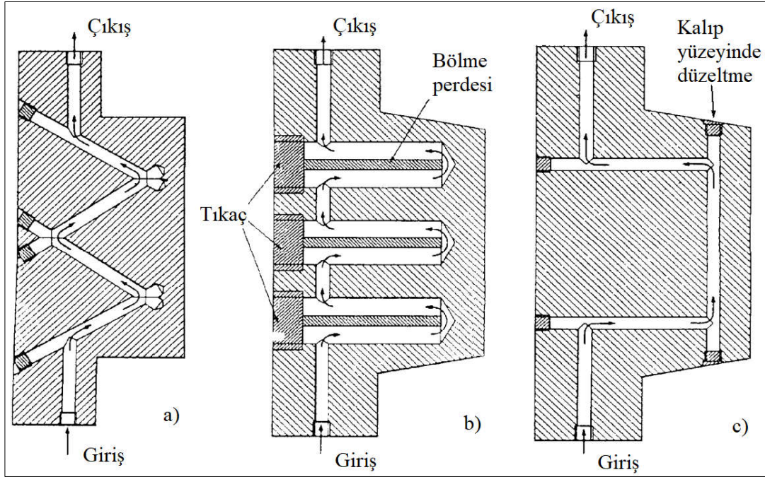
Şekil 3.23. a) Açılı delinmiş kanallar, b) Bölmeli (baffle) kanal, c) Kalıp yüzeyinden delinen kanal
