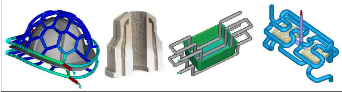
Şekil 3.26. Şekil uyumlu soğutma uygulamaları [35, 53, 61, 107]
