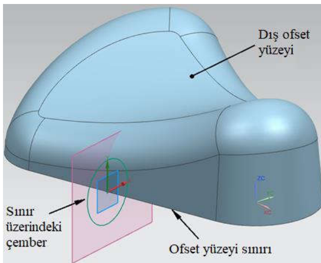
Şekil 4.5. Ofset kenarı üzerinde oluşturulan çember [69]
