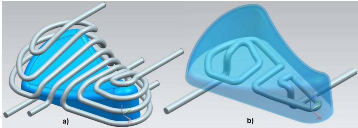
Şekil 4.11. a) Dişi ve b) Erkek kalıp yarımında soğutma kanallarının elde edilmesi [69]
