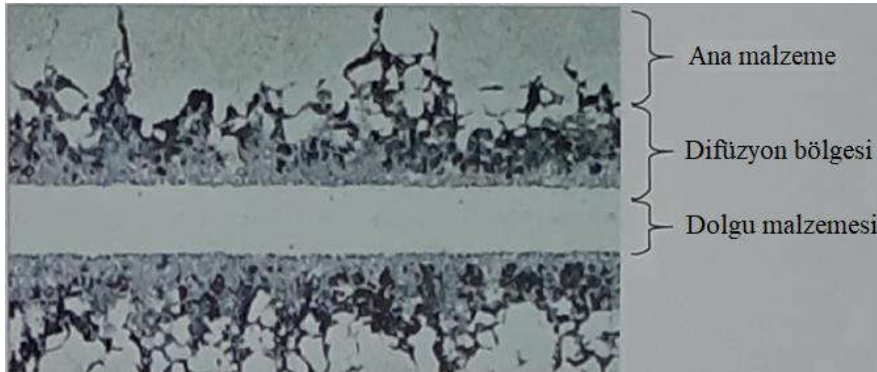
Resim 3.2. Sert lehimle birleştirme bölgesinde mikro yapı [119]
