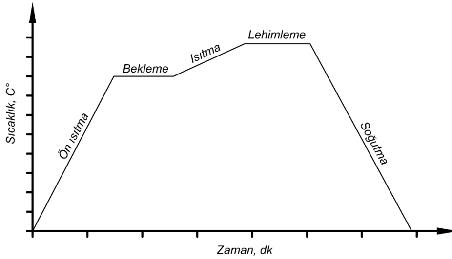
Şekil 3.31. Sert lehimlemede zaman-sıcaklık çevrimi [115, 118]
