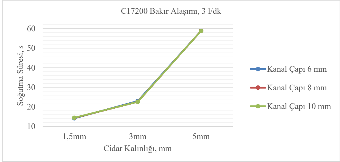
Şekil 5.17. Soğutma süresinin cidar kalınlığına göre değişimi
