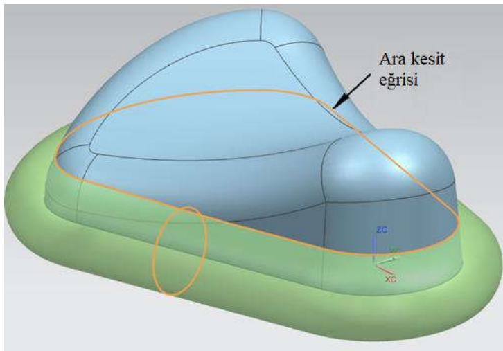
Şekil 4.7. Ara kesit eğrisinin elde edilmesi [69]
