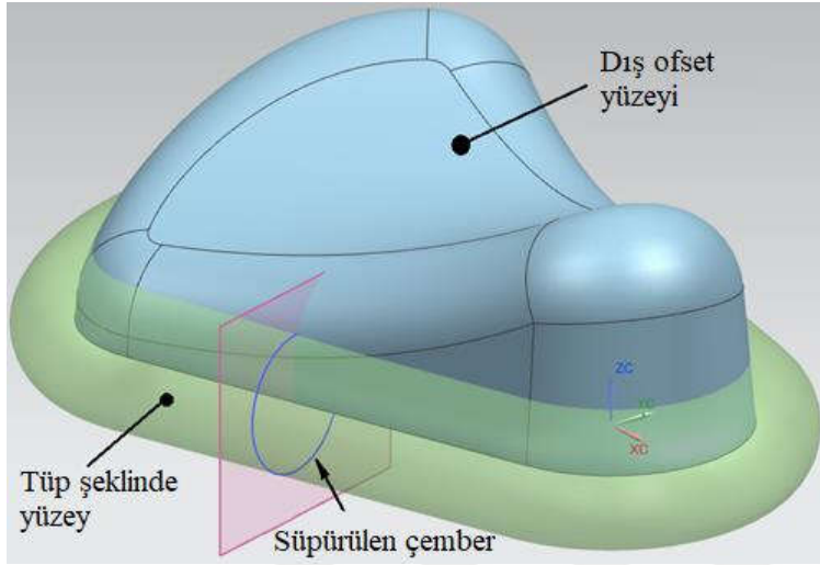
Şekil 4.6. Tüp şeklindeki yüzeyin oluşumu [69]
