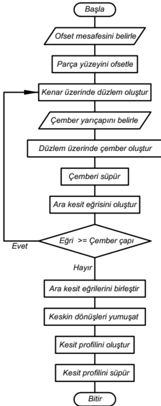
Şekil 4.2. Kanal tasarımı algoritmasının şematik gösterimi
