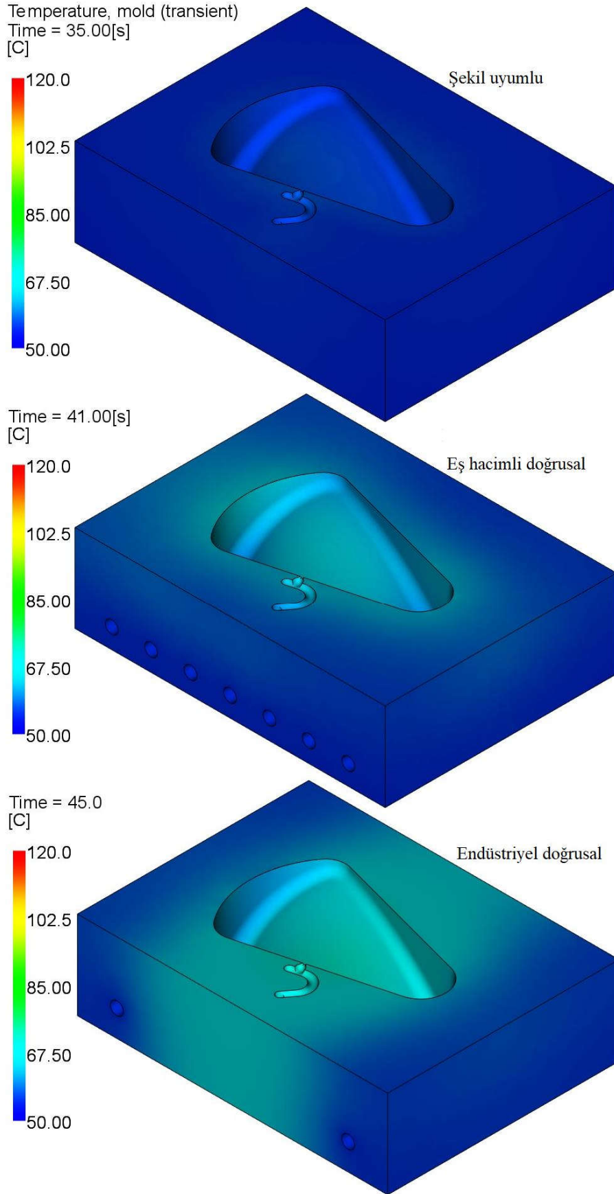
Şekil 2.2. Dişi kalıp çekirdeği üzerindeki sıcaklık dağılımları
