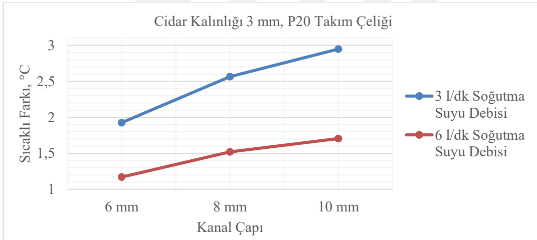
Şekil 5.26. Soğutma suyunun giriş çıkış sıcaklık farkının kanal çapına göre değişimi
