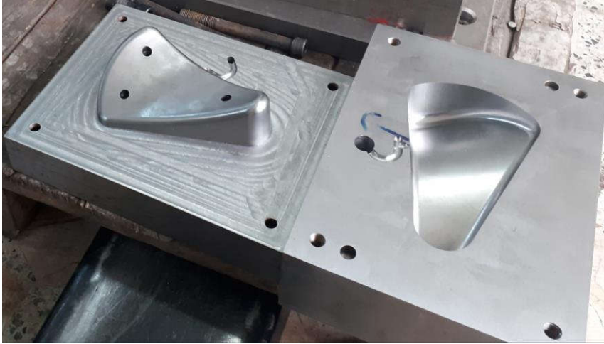
Resim 4.3. İşlenmiş kalıp çekirdekleri [84]
