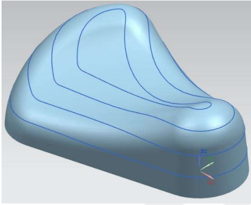
Şekil 4.8. Ara kesit tekrarı ile eğrilerin elde edilmesi [69]
