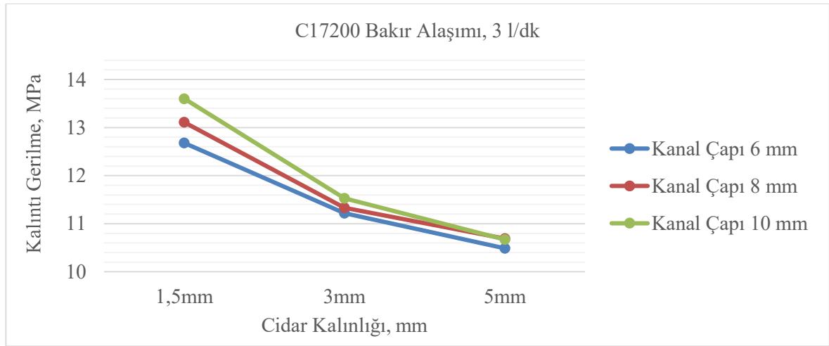
Şekil 5.25. Cidar kalınlığı ve kanal çapının kalın gerilmeye etkisi
