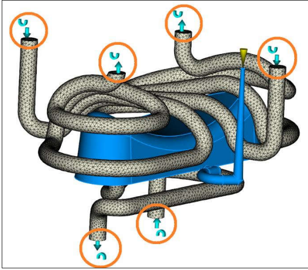
Şekil 4.24. Soğutma kanalları üzerindeki giriş ve çıkış noktaları
