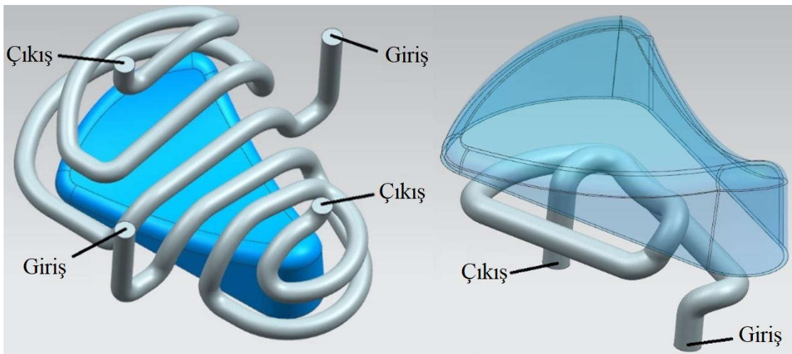
Şekil 4.13. Soğutma kanallarının su giriş ve çıkışları [84]
