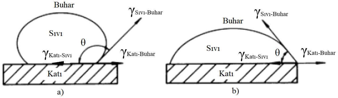
Şekil 3.30. Katı yüzey üzerindeki damlacığın temas açısı, a) \theta < 90^\circ , b) \theta > 90^\circ [117]
