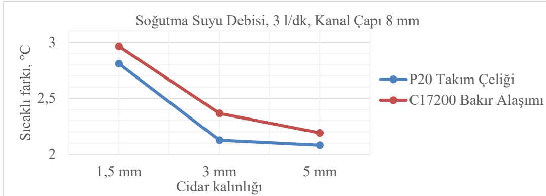
Şekil 5.27. Soğutma suyunun giriş çıkış sıcaklık farkının cidar kalınlığına göre değişimi
