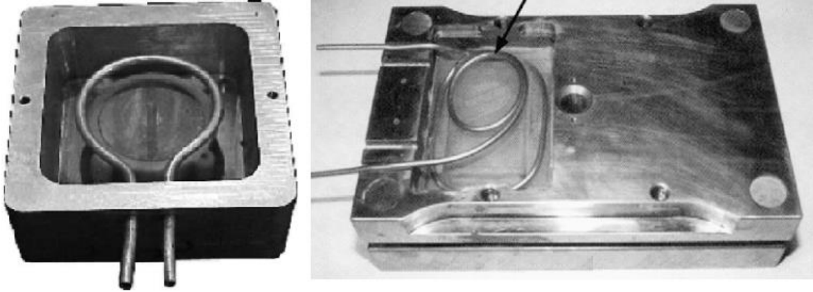
Resim 5.1. Metal boruların bükülerek kalıp içine yerleştirilmesi
