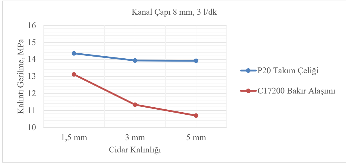
Şekil 5.24. Kalıntı gerilmenin cidar kalınlığına göre değişimi
