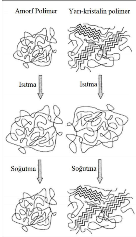
Şekil 3.2. Amorf ve Yarı-kristalin polimer malzemelerin ısı karşısındaki davranışı [87]
