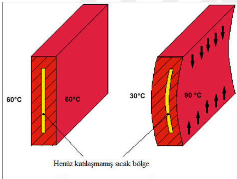
Şekil 3.15. Yüzey sıcaklık farkı nedeniyle çarpılmanın oluşumu [101]
