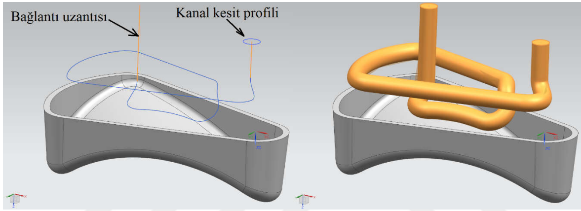
Şekil 4.10. Kanal kesit profilinin kanal hattı boyunca süpürülmesi
