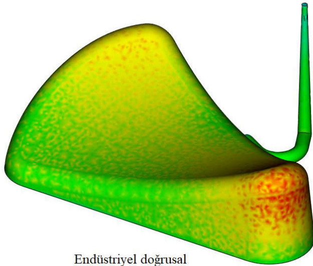
Şekil 5.8. Plastik parça üzerindeki kalıntı gerilmeler
