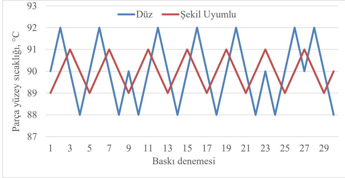
Şekil 5.11. Baskı demelerine göre kalıptan çıkan parçalarının yüzey sıcaklıkları
