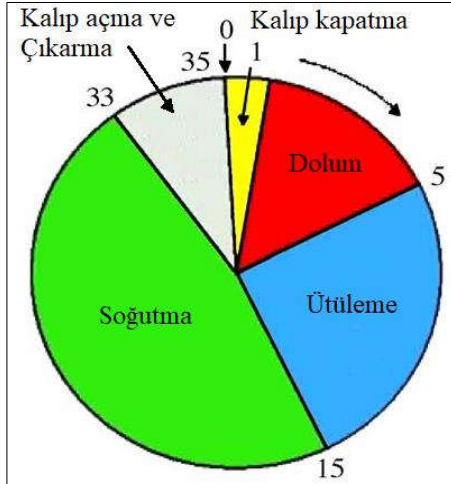
Şekil 3.14. Çevrim süresinde işlemlerin zaman aralıkları [3]
