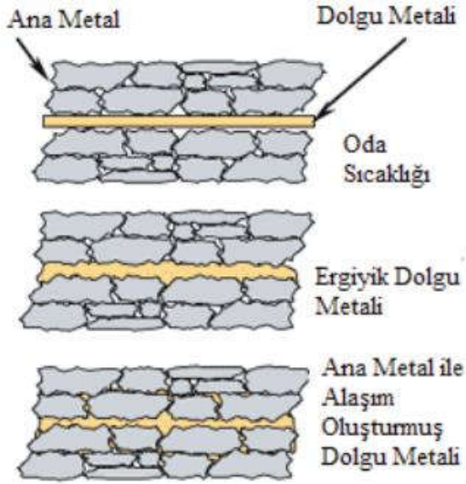
Şekil 3.28. Lehim oluşum mekanizması [114]
