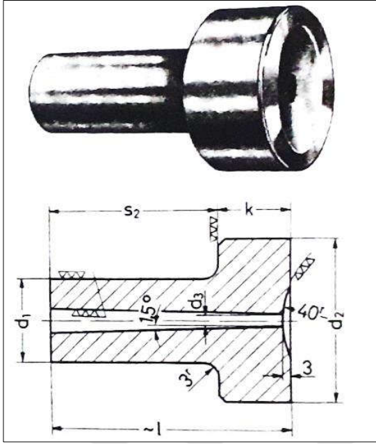
Şekil 3.7. Yolluk burcunun yapısı [94]
