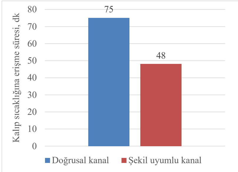
Şekil 5.12. Kalıp sıcaklığının dengeye gelme süreleri
