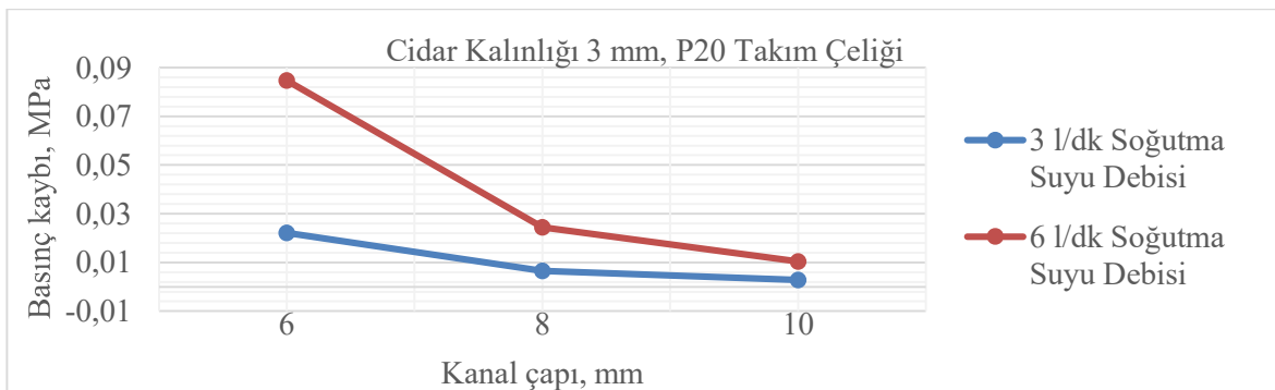
Şekil 5.28. Soğutma kanalındaki basınç kaybının kanal çapına göre değişimi
