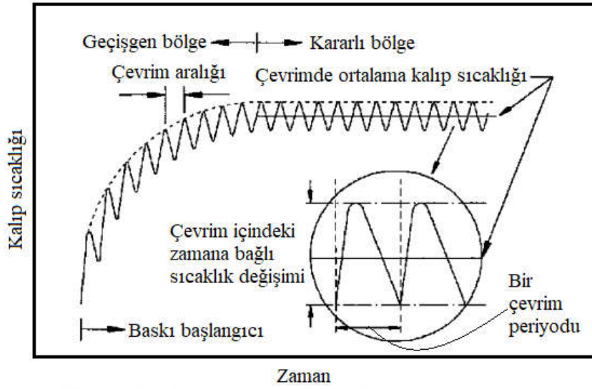
Şekil 3.16. Kalıp sıcaklığının zamanla değişimi [17]
