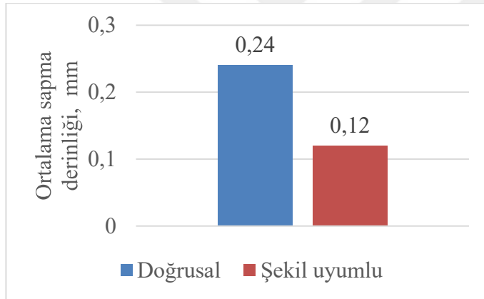
Şekil 5.14. Ortalama sapma derinlikleri
