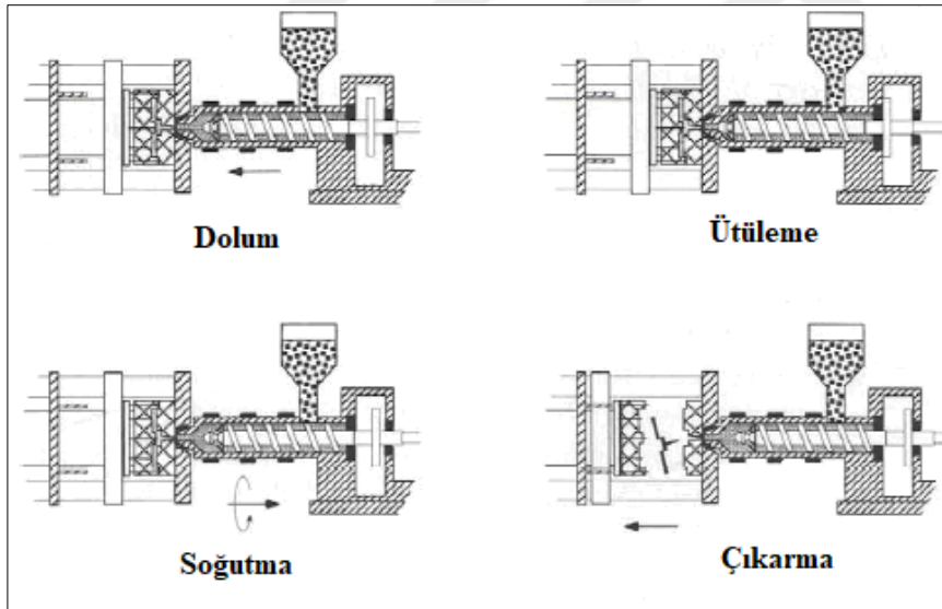
Şekil 3.4. Plastik enjeksiyon kalıplamada üretim safhaları [92]
