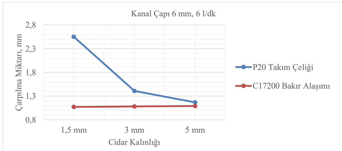
Şekil 5.22. Kalıp malzemesi ve cidar kalınlığının çarpılma miktarına etkisi
