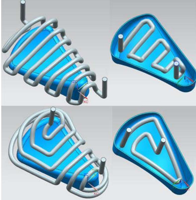
Şekil 4.12. Zikzak ve spiral şekil uyumlu soğutma kanalları
