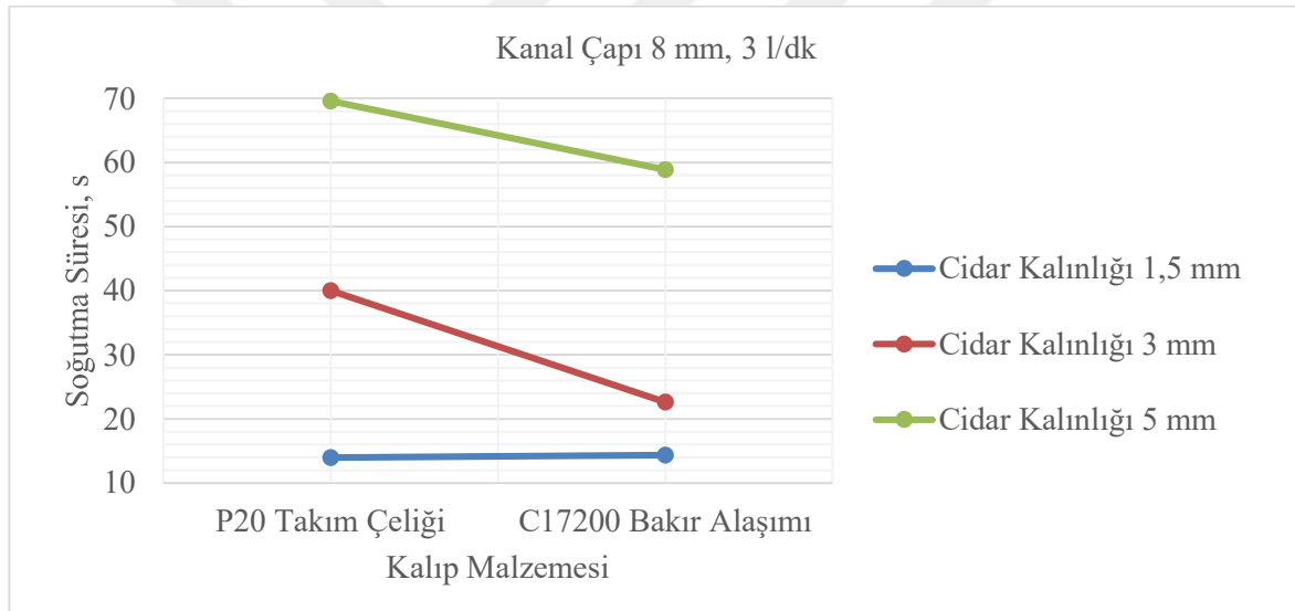
Şekil 5.19. Soğutma süresinin kalıp malzemesine göre değişimi
