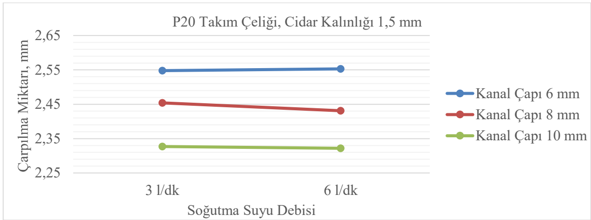
Şekil 5.23. Çarpılma miktarının soğutma suyu debisine göre değişimi
