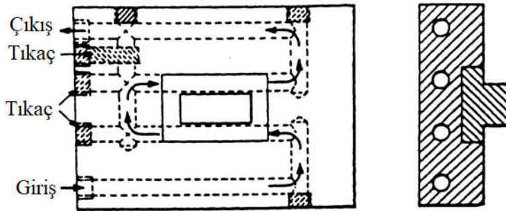
Şekil 3.20. Erkek kalıp plakasının soğutulması
