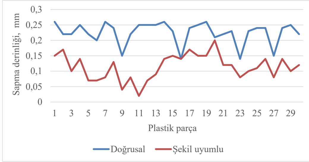
Şekil 5.13. Plastik parça üzerinde düzlemsel yüzeydeki sapma derinlikleri
