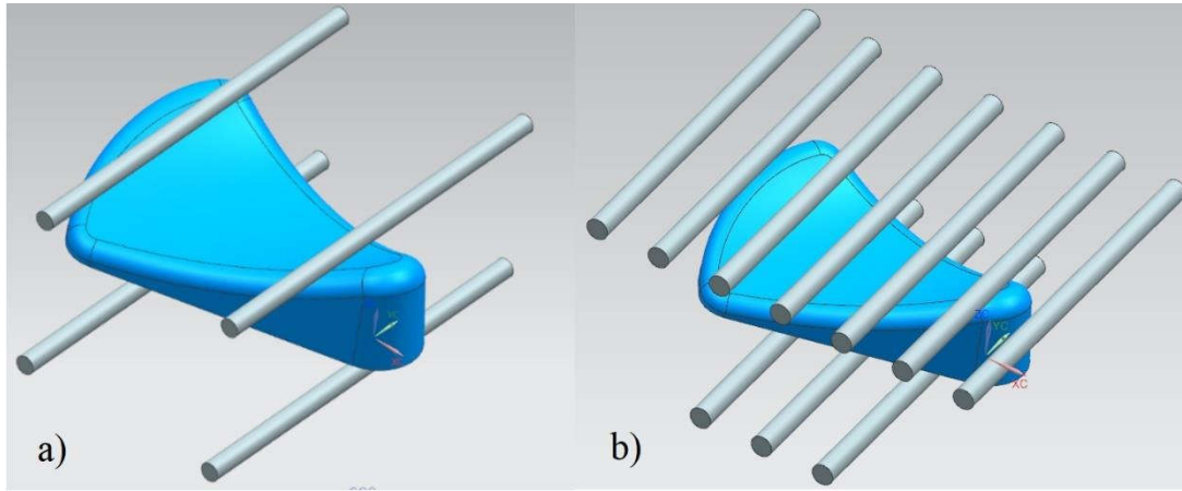
Şekil 4.14. Doğrusal soğutma kanalları, a) Endüstriyel, b) Eş hacimli
