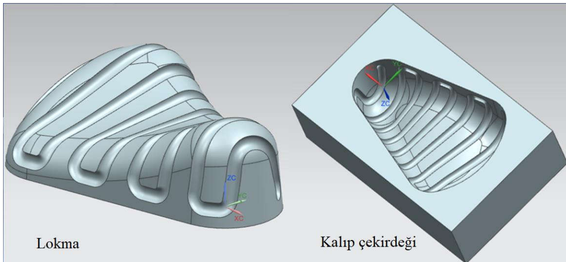
Şekil 5.1. Kalıp çekirdeğinin parçalı olarak üretimi
