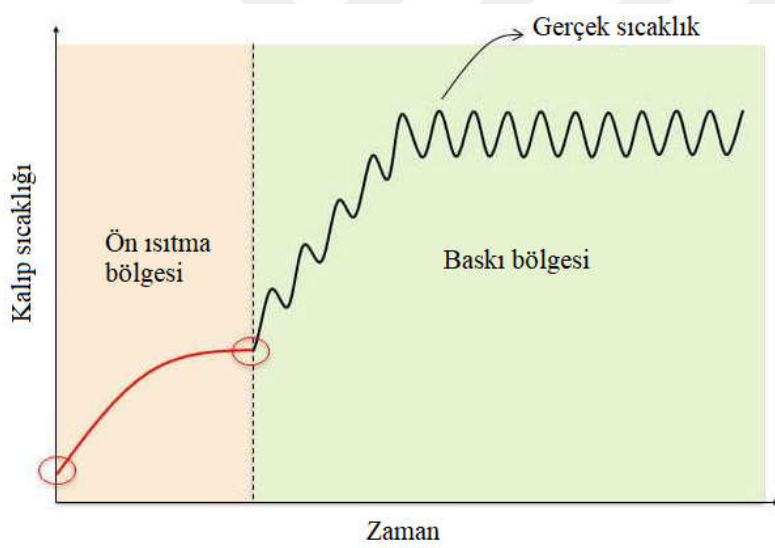
Şekil 3.17. Kalıp şartlandırıcı ile yapılan ön ısıtma [105]
