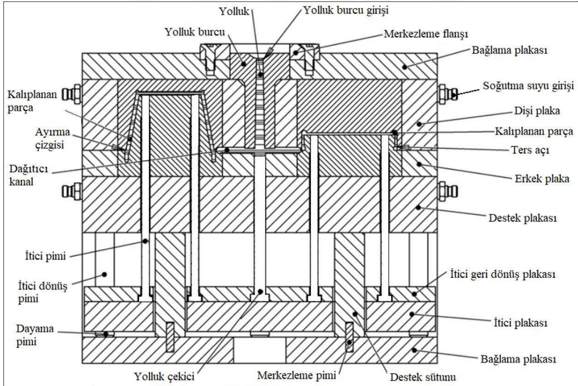
Şekil 3.5. Plastik enjeksiyon kalıbının genel yapısı [91]
