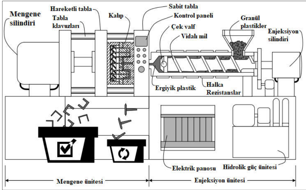
Şekil 3.3. Plastik enjeksiyon makinesinin bölümleri [91]
