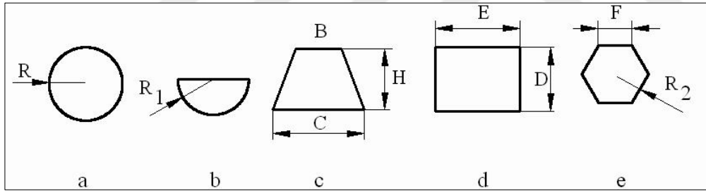
Şekil 3.9. Dağıtıcı kanal kesitleri, a. Daire, b. Yarım daire, c. Trapez, d. Dikdörtgen, e.
