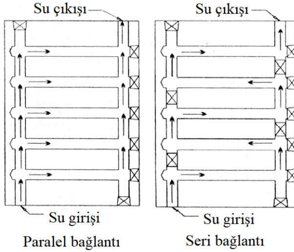
Şekil 3.22. Seri ve Paralel bağlantı tipleri
