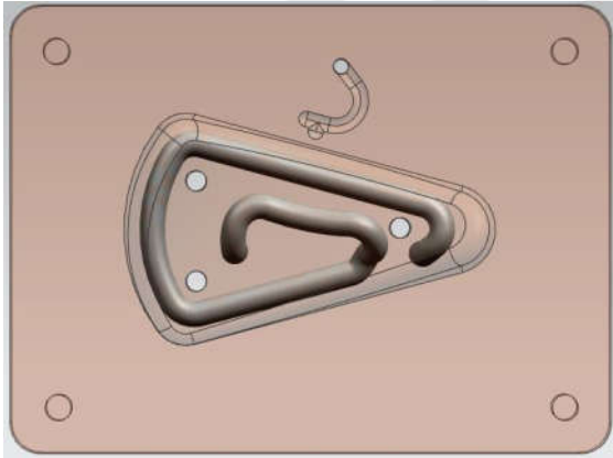
Şekil 4.20. İtici pim deliklerinin konumu
