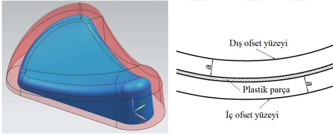
Şekil 4.3. Ofsetlenerek elde edilen referans yüzeyler [69].
