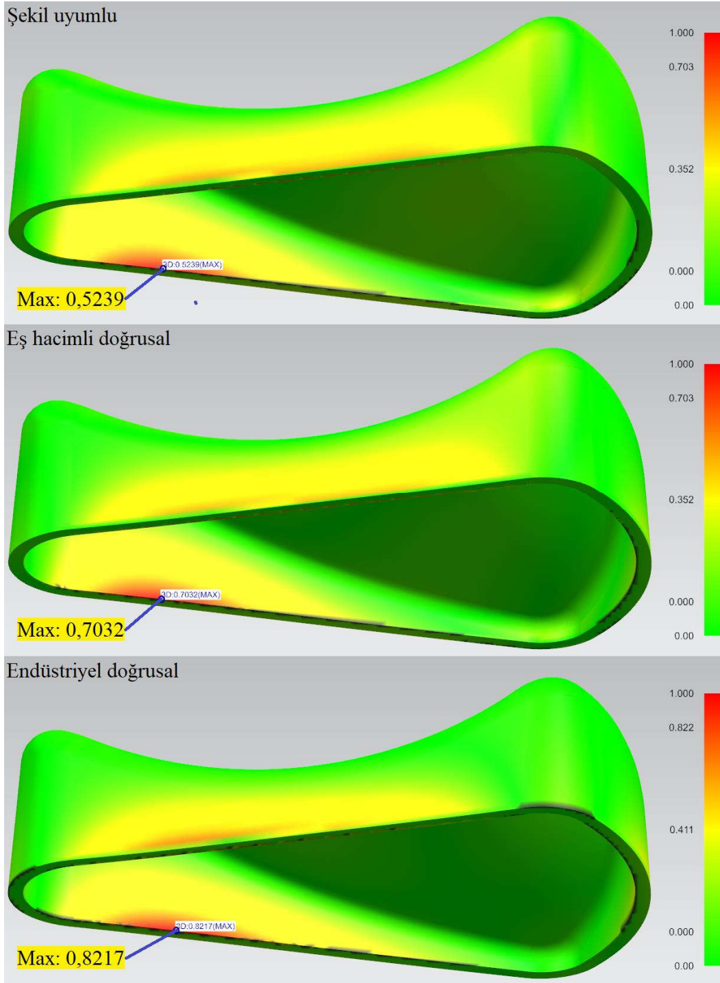
Şekil 5.7. Yüzeylerdeki mutlak sapma değerlerinin dağılımı
