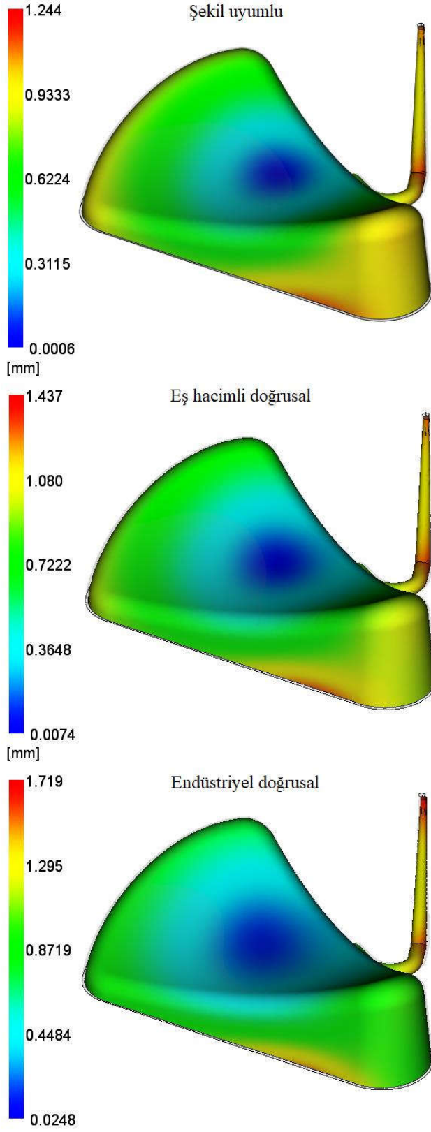
Şekil 5.6. Çarpılma değerlerinin dağılımı
