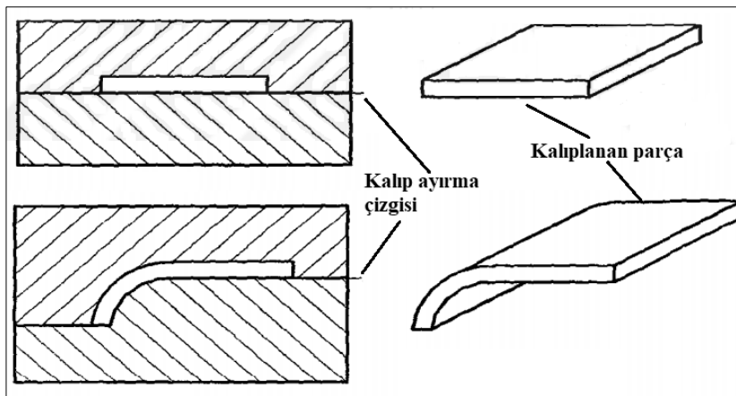
Şekil 3.11. Kalıp ayırma çizgisi [96]
