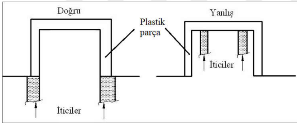
Şekil 3.13. Uygun itici konumları [95]
