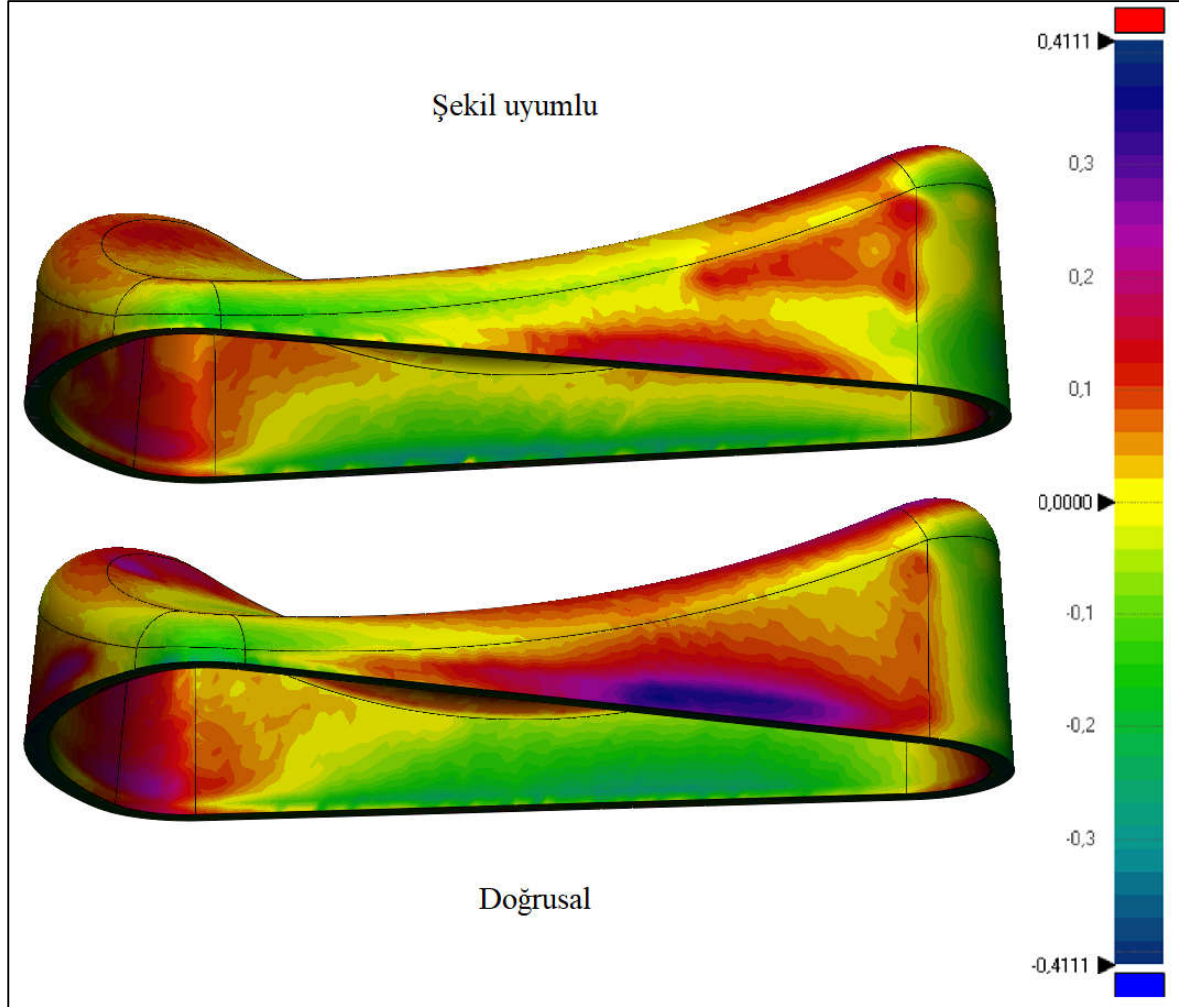
Şekil 5.15. Deney parçalarının yüzeyindeki çarpılma miktarı dağılımı
