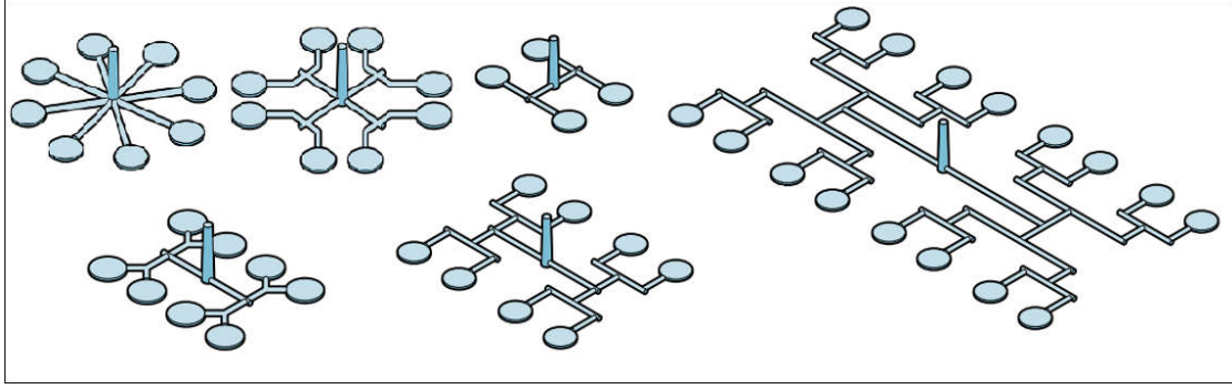
Şekil 3.8. Geometrik olarak dengelenmiş dağıtıcı kanal tasarımları
