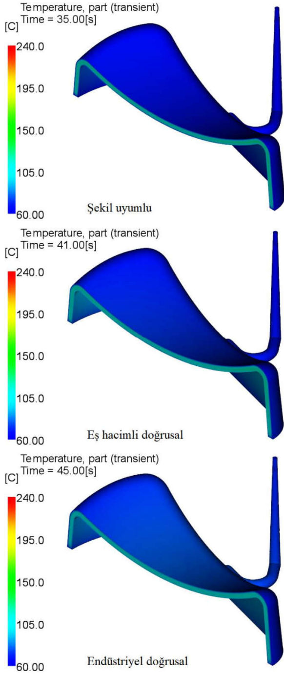
Şekil 5.4. Çıkarma sıcaklığına erişim sürelerindeki sıcaklık dağılımları
