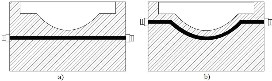
Şekil 3.25. a) Doğrusal soğutma kanalı, b) Şekil uyumlu soğutma kanalı
