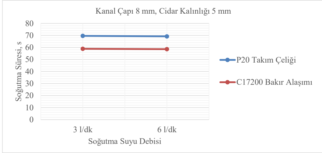
Şekil 5.20. Soğutma süresinin soğutma suyu debisine göre değişimi
