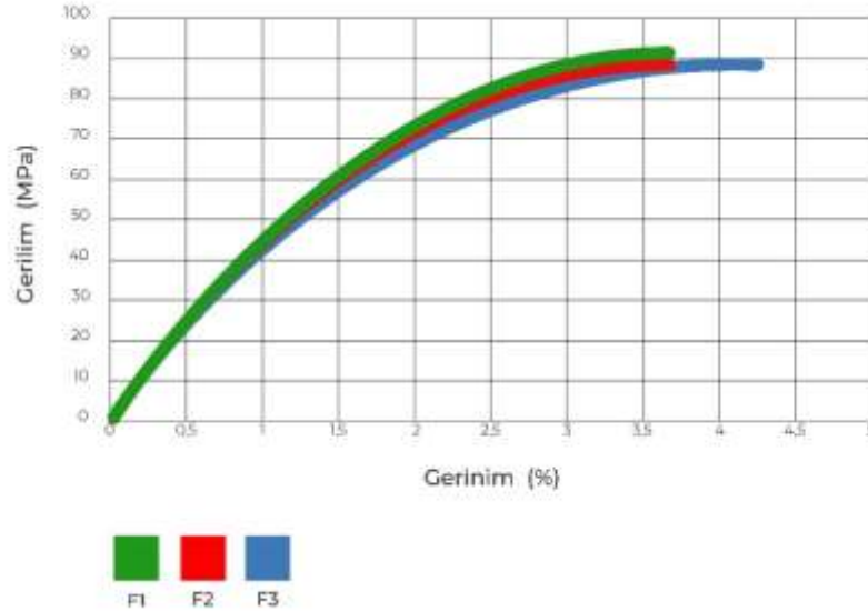
Şekil 5.11 F numunesine ait gerilim – gerinim grafiği
