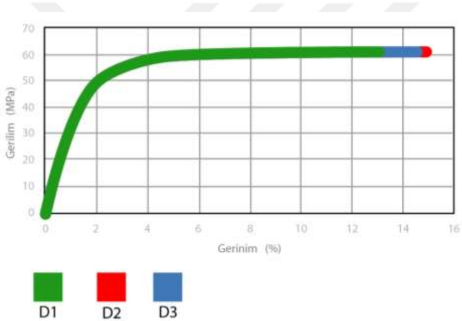
Şekil 5.7 D numunesine ait gerilim – gerinim grafiği
