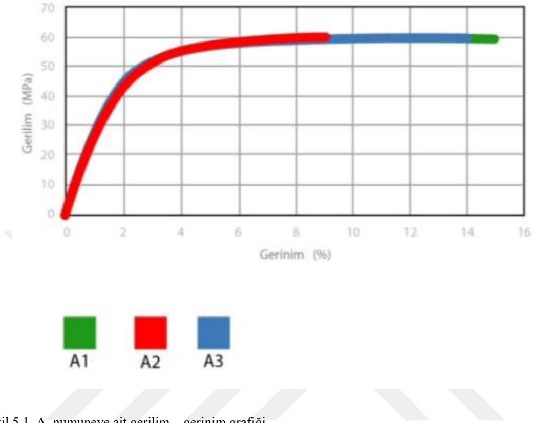
Şekil 5.1 A. numuneye ait gerilim – gerinim grafiği
