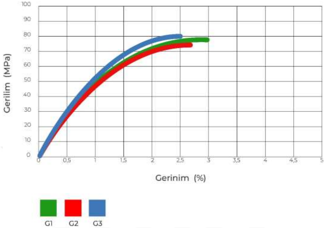
Şekil 5.13 G numuneye ait gerilim – gerinim grafiği
