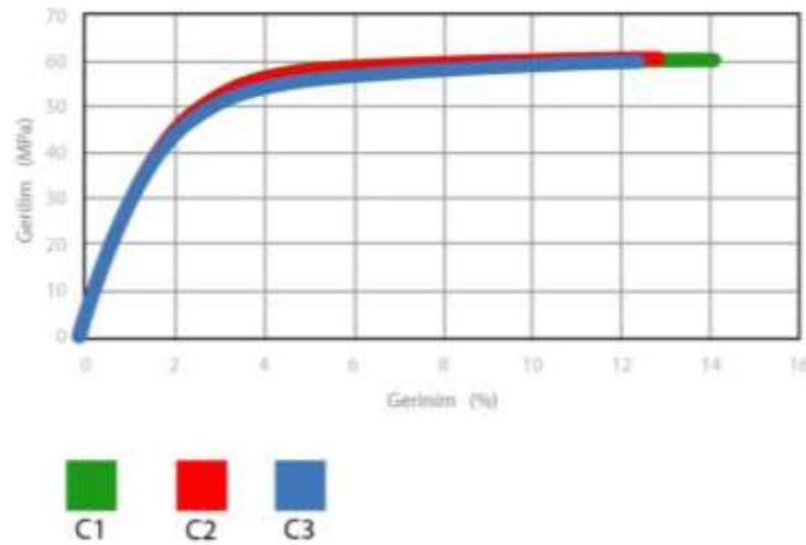
Şekil 5.5 C numunesine ait gerilim – gerinim grafiği
