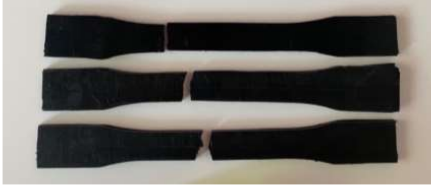
Şekil 5.2 Çekme Testi Sonrası Numune A
