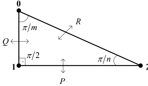
Şekil 6.1. Üçgenin kenarındaki yansımalar
