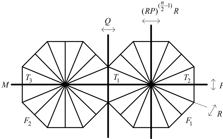
Şekil 6.2. Dönel otomorfizma
