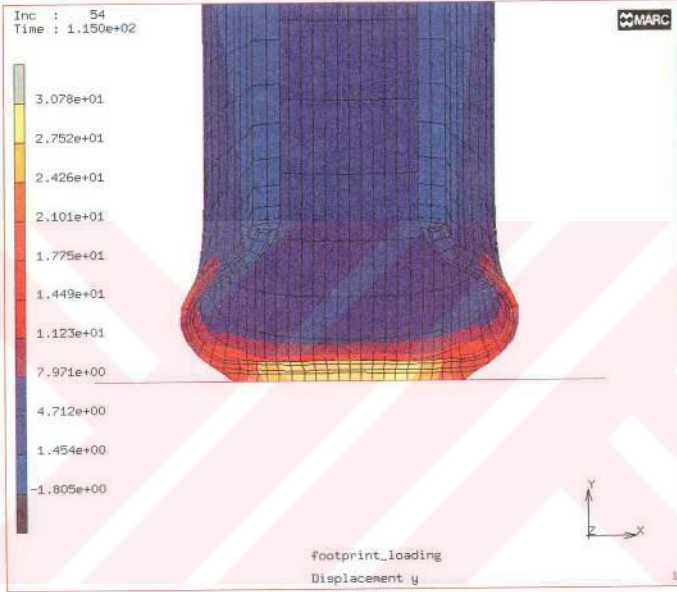
Şekil 52. 25 mm'lik temas yüzey deplasmanında oluşan radyal yer değiştirmenin dağılımı (Model 2)
