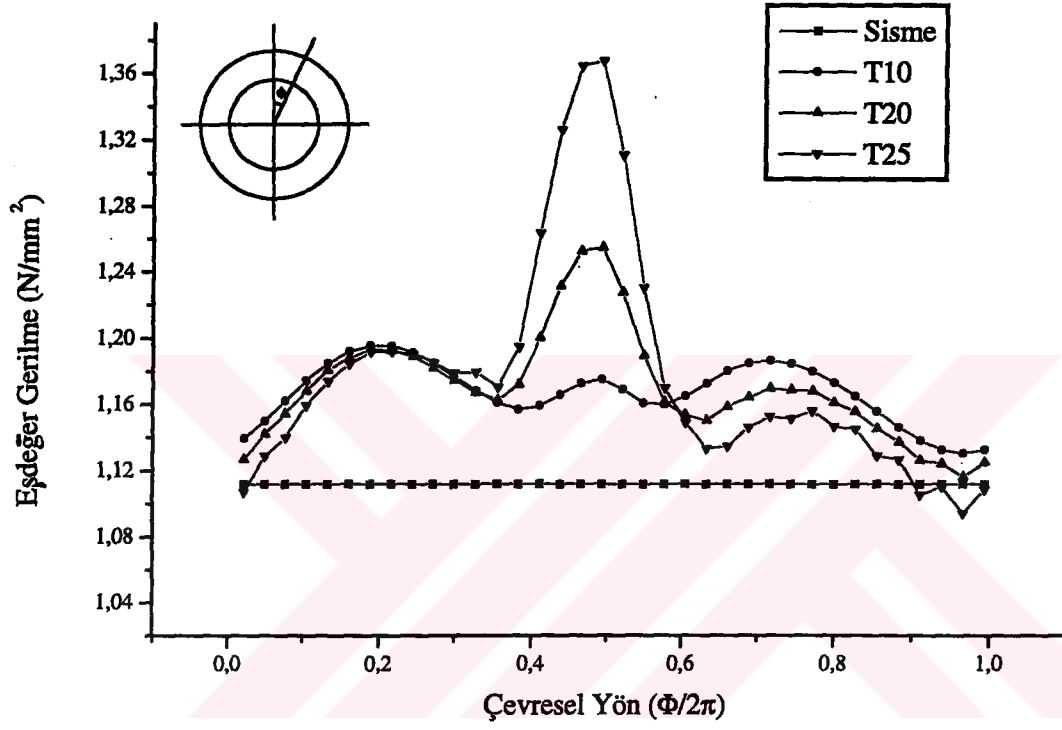
Şekil 78. Eleman 317'nin çevresel yöndeki eşdeğer gerilme değişimi.
