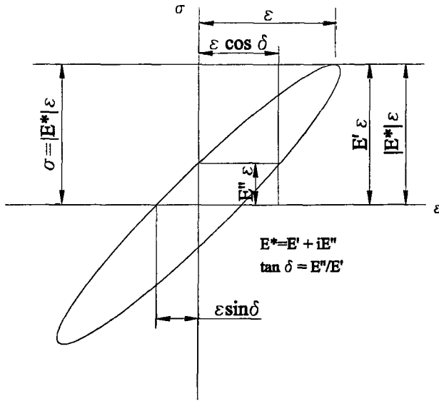
Şekil 14: Kayıp modülü ve faz açısı arasındaki ilişkiyi göstren histeresis çevrimi
