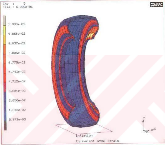
Şekil 30. Şişirme basıncı (2 Bar) etkisinde tekerde oluşan eşdeğer şekil değiştirmenin dağılımı (Model 1)
