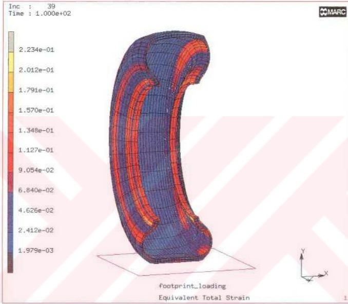
Şekil 48. Şişirme basıncı, santrifüj kuvvet ve araç yükü (20 mm'lik temas yüzey deplasmanında) etkisinde tekerde oluşan eşdeğer şekil değiştirmenin dağılımı (Model 2)
