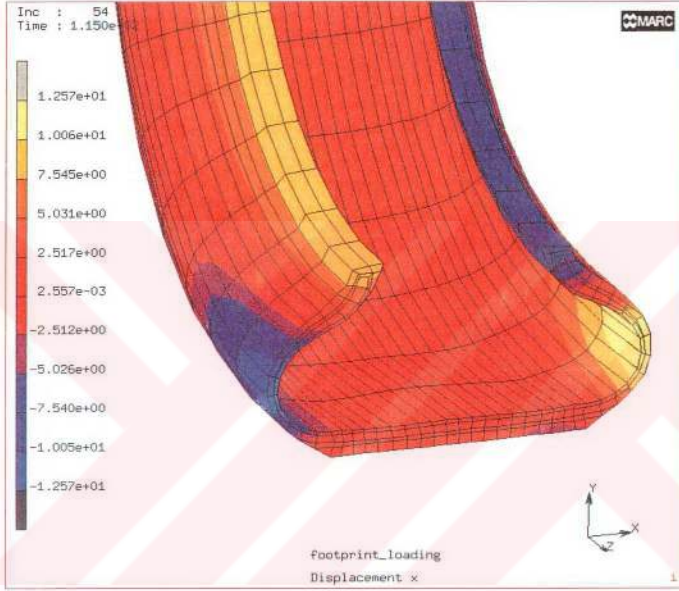
Şekil 77. 25mm'lik temas yüzeyi deplasmanında termal yüklemekten sonra oluşan maksimum yanak deplasmanı (Model 2)
