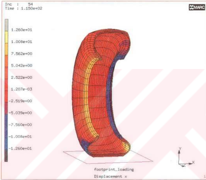
Şekil 53. 25 mm'lik temas yüzey deplasmanında oluşan aksenal yer değıştirmenin dağılımı (Model 2)
