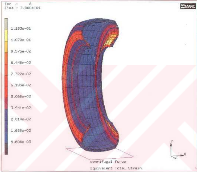
Şekil 47. Şişirme basıncı (2 Bar) + santrifuj kuvvet (80 km/h) etkisinde tekerde oluşan eşdeğer şekil değiştirmenin dağılımı (Model 2)
