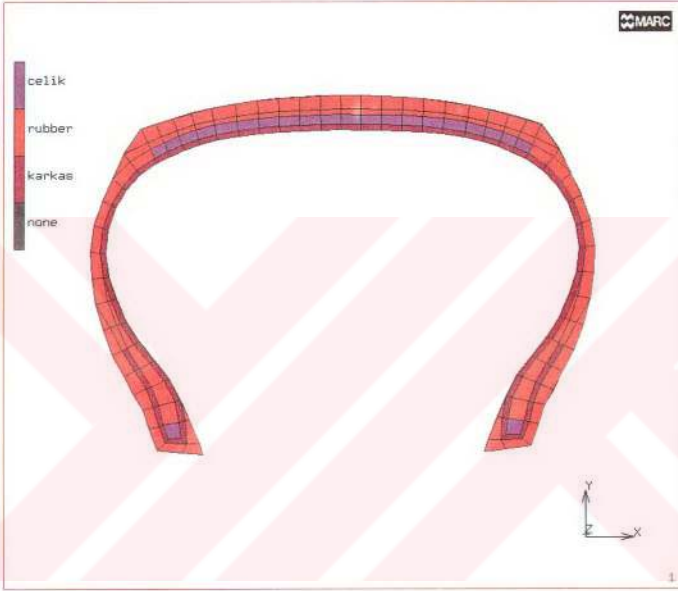
Şekil 58. Termal analizde kullanılan malzeme bölgeleri (Model 2)
