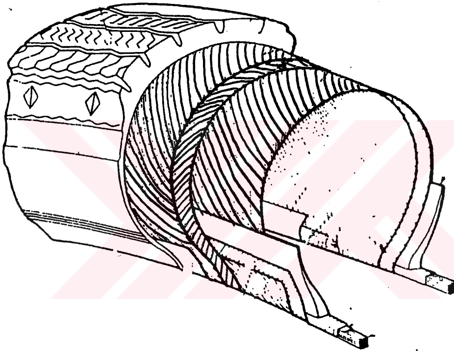
Şekil 2. Çapraz gövde katmanlı teker
