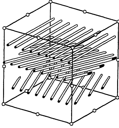
Şekil 11: Rebar elemandaki kordların yönlenmesi.
