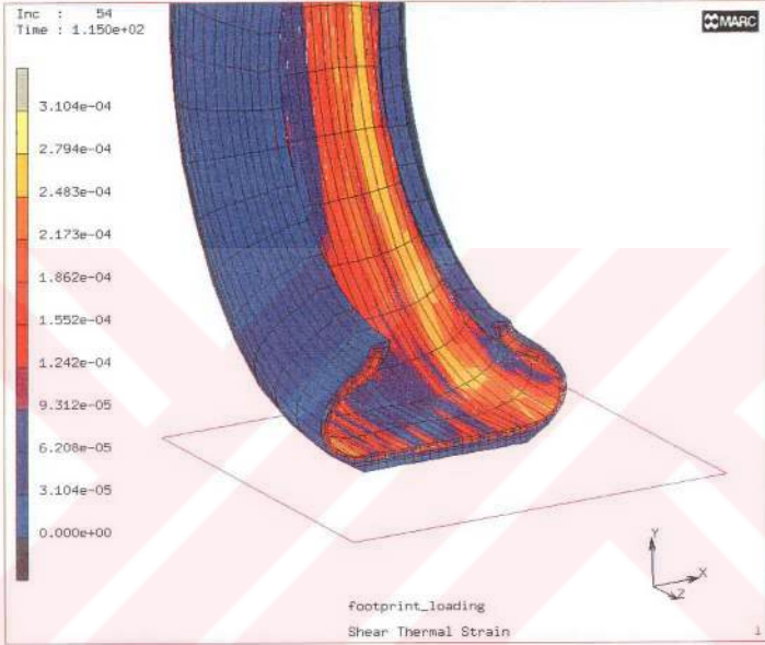
Şekil 74. 25mm'lik temas yüzeyi deplasmanında termal yüklemekten sonra oluşan kayma gerilmeleri (Model 2)
