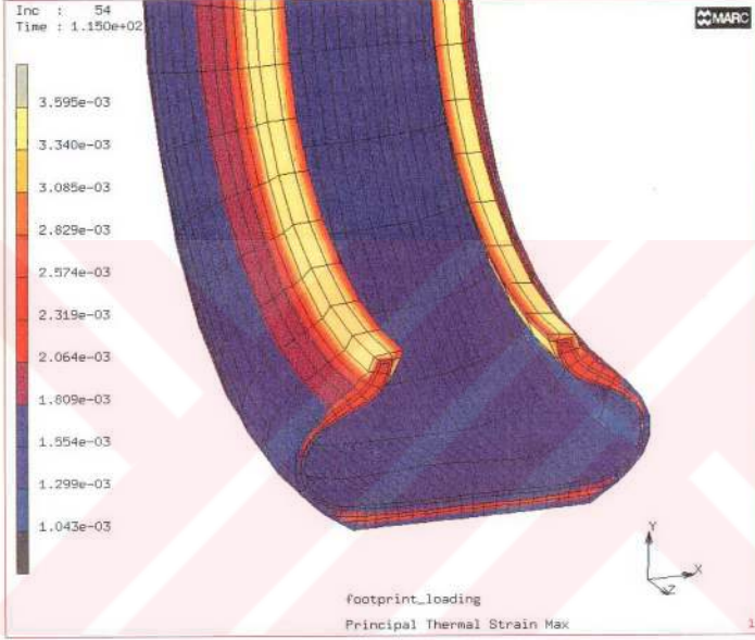
Şekil 76. 25mm'lik temas yüzeyi deplasmanında termal yüklemekten sonra oluşan maksimum şekil değişimi (Model 2)
