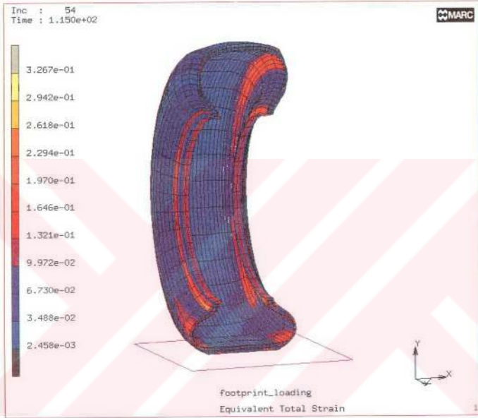
Şekil 49. Şişirme basıncı, santrifüj kuvvet ve araç yükü (25 mm'lik temas yüzey deplasmanında) etkisinde tekerde oluşan eşdeğer şekil değiştirmenin dağılımı (Model 2)
