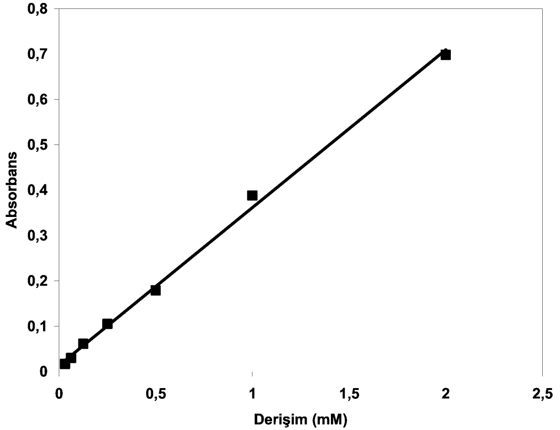
Şekil 3.1. p-Nitrofenil \beta -D-galaktosid kalibrasyon grafiđi
