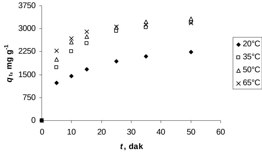
Şekil 3.24. p-VIm-C14 üzerine OII adsorpsiyonunun zamana bağlılığı. Deney koşulları: Bkz. Şekil 3.17.
