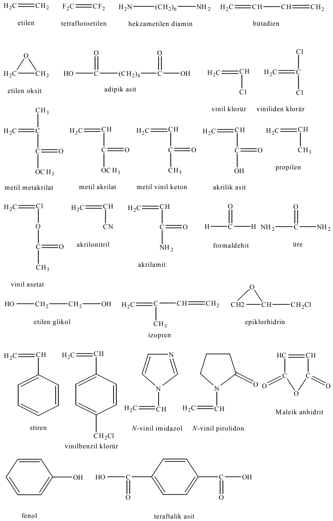
Şekil 1.2. Bazı monomerlerin kimyasal yapıları
