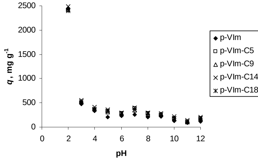
Şekil 3.12. Adsorbanlar üzerine OII adsorpsiyonunun pH ile değişimi. Deney koşulları: [Hidrojel]=0,2 mg mL -1 , [OII]= 500 mg L -1 , V_{\text{toplam}} = 100 mL, pH= 2,0-12,0.
