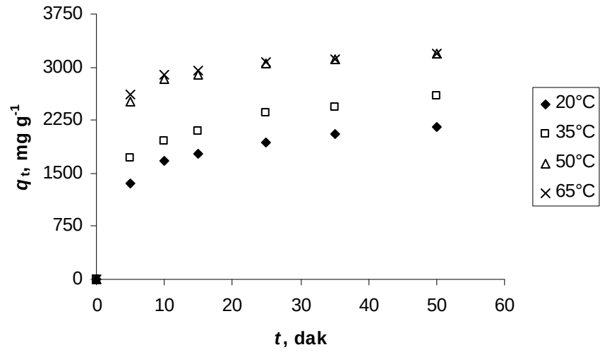
Şekil 3.25. p-VIm-C18 üzerine OII adsorpsiyonunun zamana bağlılığı. Deney koşulları: Bkz. Şekil 3.17.
