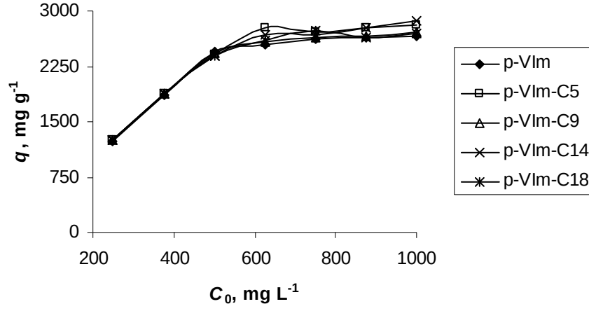
Şekil 3.14. OII başlangıç derişiminin hidrojelilerin adsorpsiyon kapasiteleri üzerine etkisi. Deney koşulları: [Hidrojel]= 0,2 mg mL -1 , [OII]= 250 mg L -1 -1000 mg L -1 , V_{\text{toplam}} = 100 mL, pH= 2,0.
