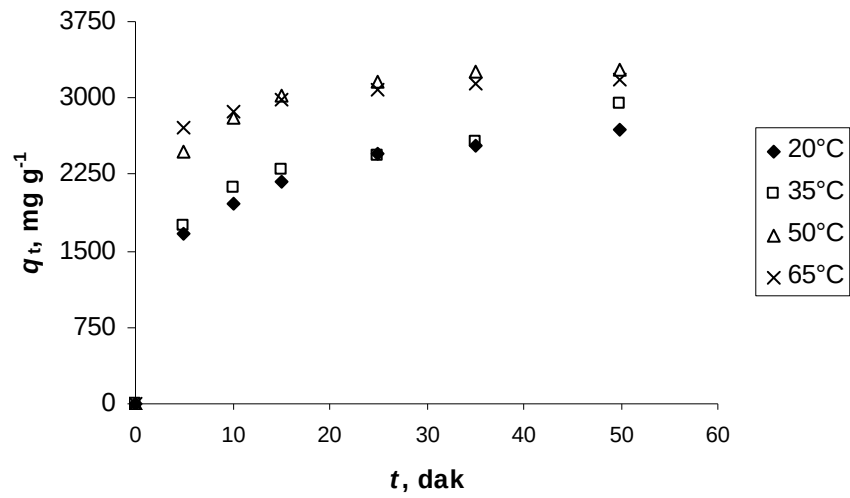
Şekil 3.17. p-VIm üzerine OII adsorpsiyonun zamana bağlılığı. Deney koşulları: [Hidrojel]= 0,2 mg mL -1 , [OII]= 700 mg L -1 , V_{\text{toplam}} = 100 mL, pH= 2,0, T= 293,15K–338,15 K.
