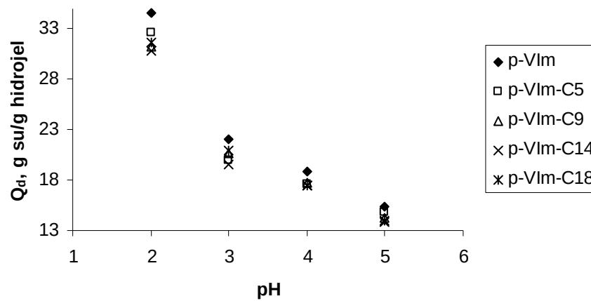
Şekil 3.4. Hidrojellerin denge şişme oranlarının pH’ a bağlılığı
