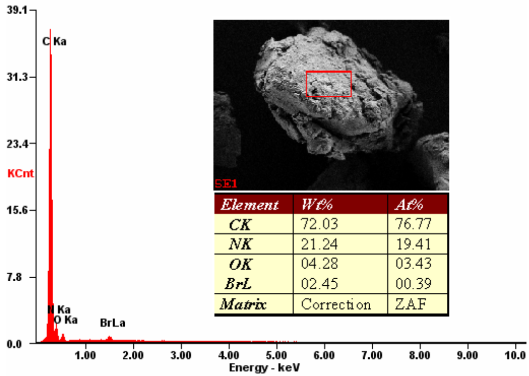
Şekil 3.8. p-VIm-C5 hidrojeline ait X-ışını spektrumu
