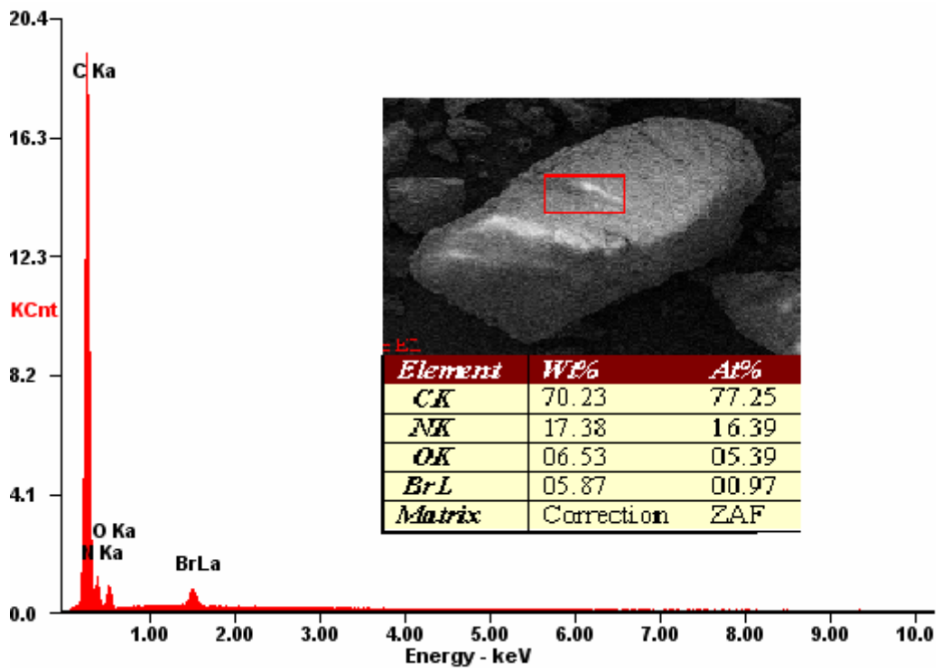
Şekil 3.9. p-VIm-C9 hidrojeline ait X-ışını spektrumu
