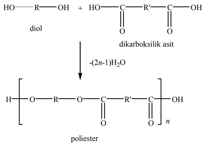
Şekil 1.7. Poliester oluşumu
