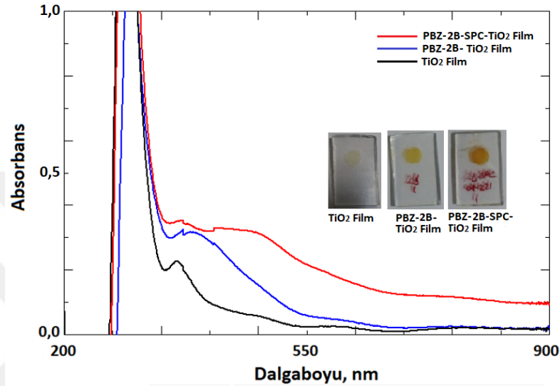
Şekil 8.4. \text{TiO}_2 , PBZ-2B- \text{TiO}_2 ve PBZ-2B-SPC- \text{TiO}_2 katı filmleri için UV-Vis Spektrumu.
