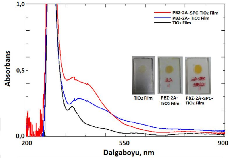
Şekil 8.2. \text{TiO}_2 , PBZ-2A- \text{TiO}_2 ve PBZ-2A-SPC- \text{TiO}_2 katı filmleri için UV-Vis Spektrumu.
