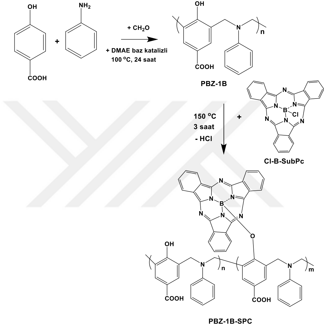
Şekil 7.17. PBZ-1B-SPC sentez reaksiyonu.
