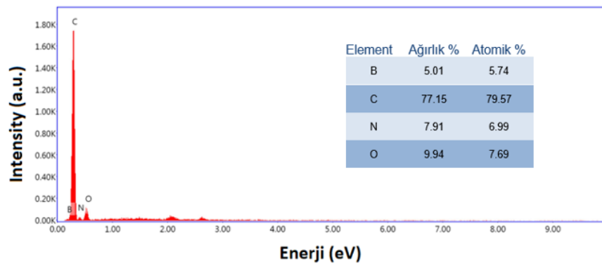
Şekil 7.48. PBZ-2A-SPC-MW için EDX spektrumu elementel analiz sonuçları.
