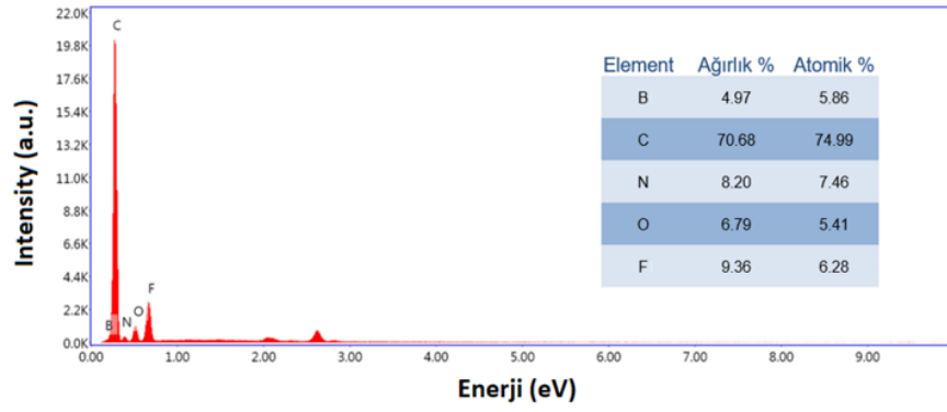
Şekil 7.8. PBZ-1A-SPC için EDX spektrumu elementel analiz sonuçları.
