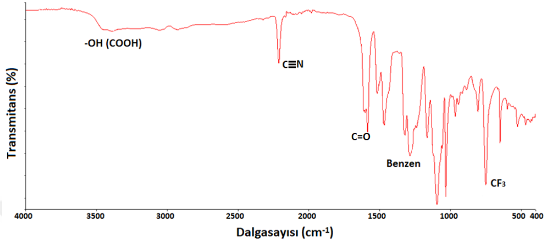
Şekil 6.10. PBZ-2A polimerinin FT-IR yapı tayini.
