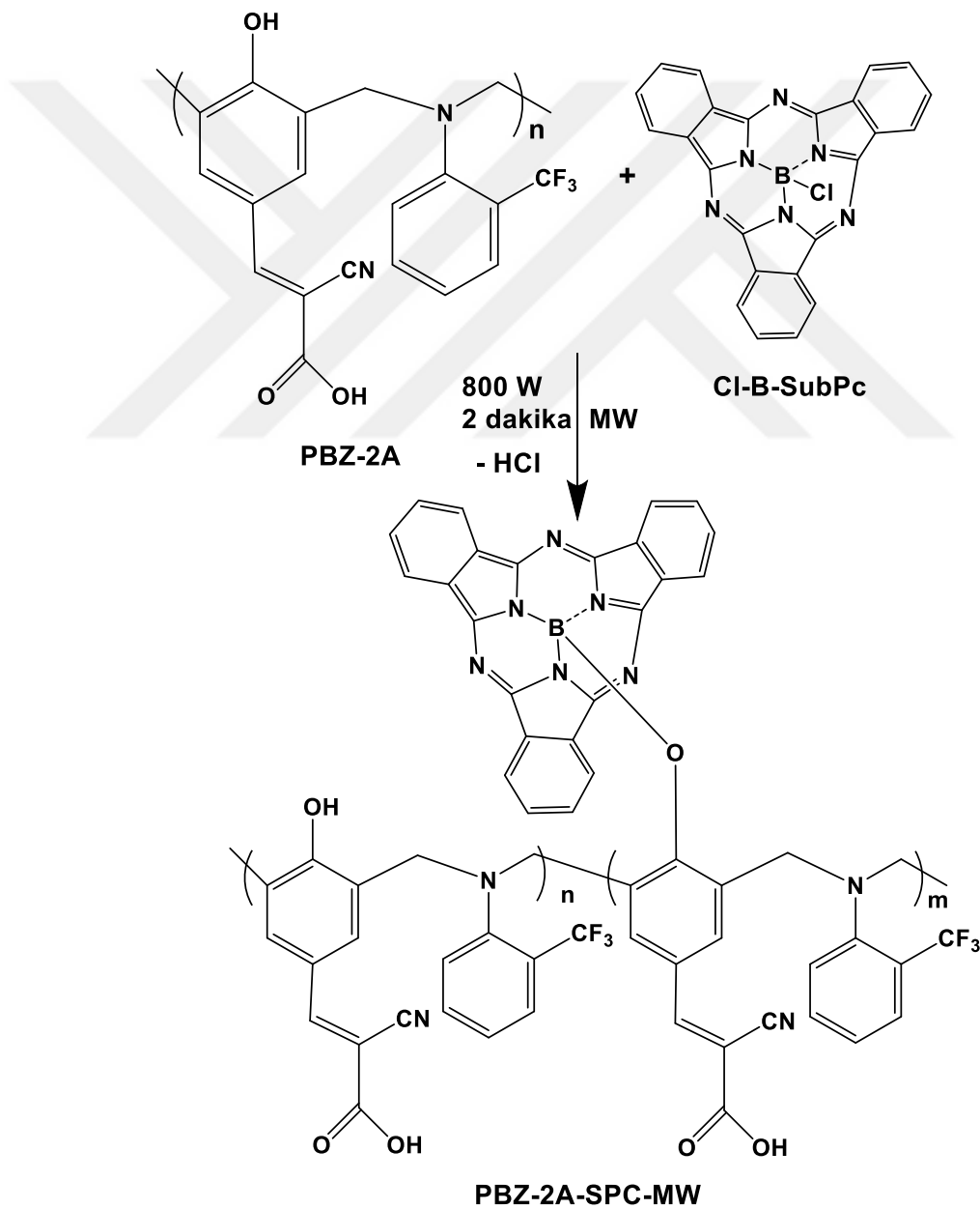
Şekil 7.37. PBZ-2A-SPC-MW mikrodalga sentez reaksiyonu.
