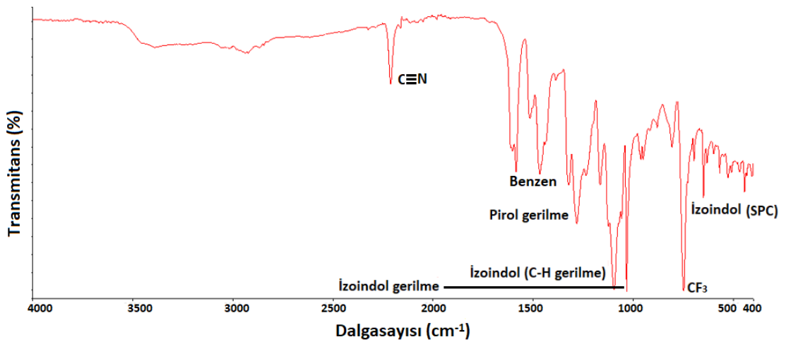
Şekil 7.11. PBZ-2A-SPC polimerinin FT-IR sepektrumu yapı tayini.
