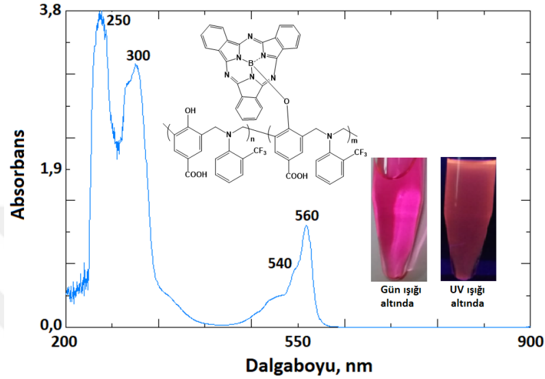
Şekil 7.33. PBZ-1A-SPC-MW polimerinin THF çözeltisinin UV-Vis spektrumu.
