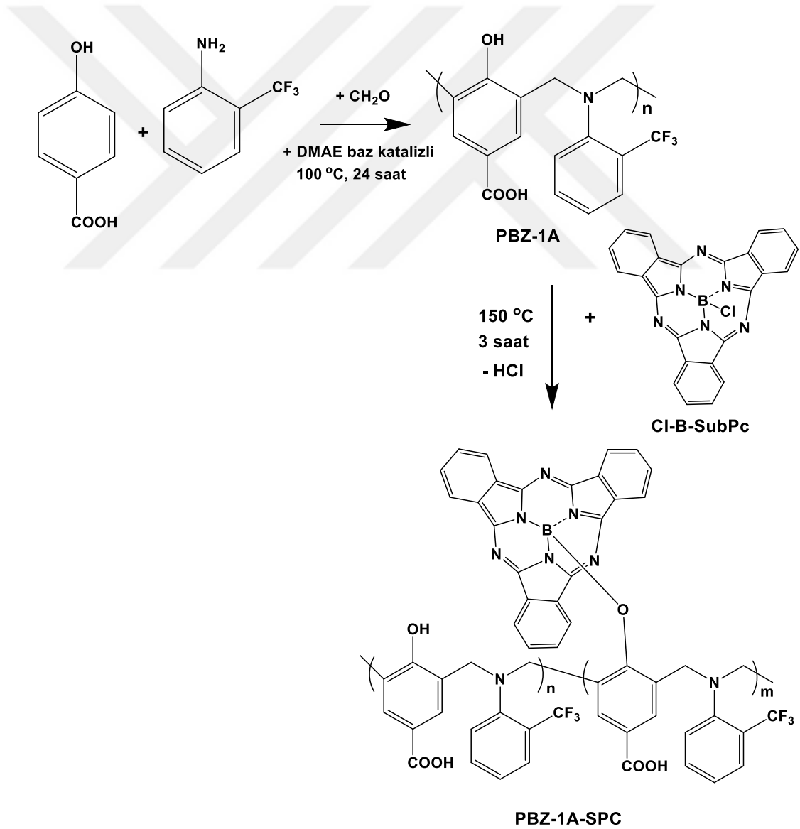
Şekil 7.3. PBZ-1A-SPC sentez reaksiyonu.
