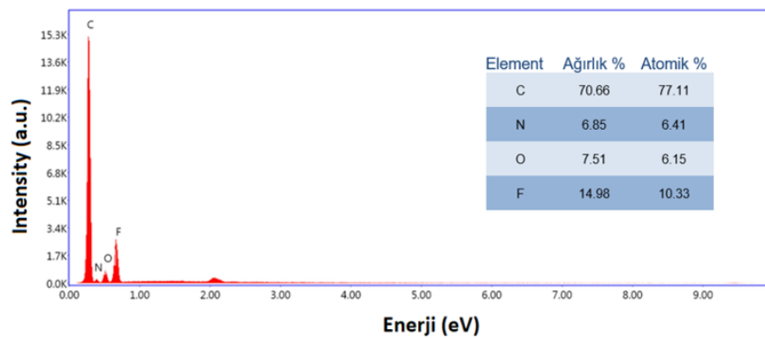
Şekil 6.6. PBZ-1A için EDX spektrumu elementel analiz sonuçları.
