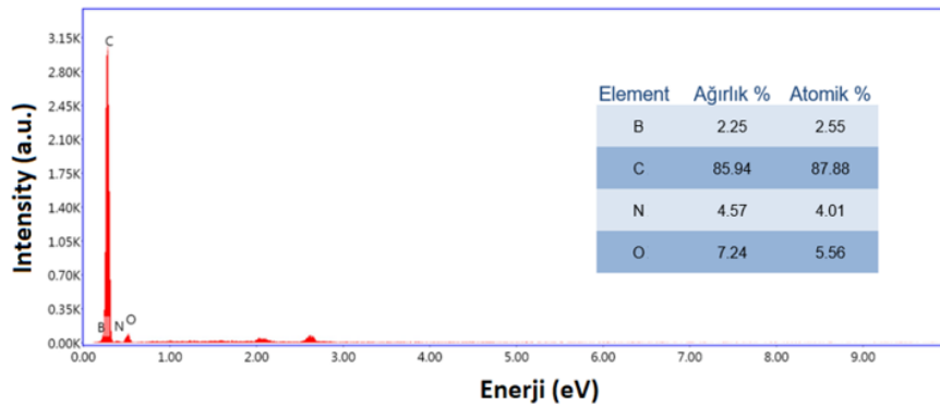
Şekil 7.22. PBZ-1B-SPC için EDX spektrumu elementel analiz sonuçları.
