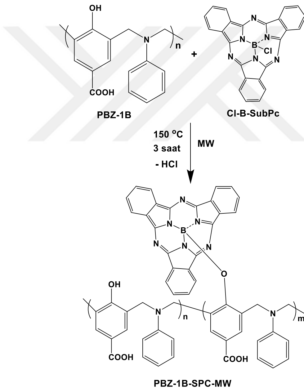
Şekil 7.43. PBZ-1B-SPC-MW mikrodalga sentez reaksiyonu.
