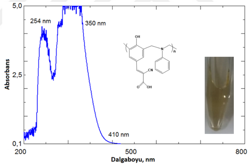
Şekil 6.27. PBZ-2B polimerinin THF çözeltisinin UV-Vis spektrumu.
