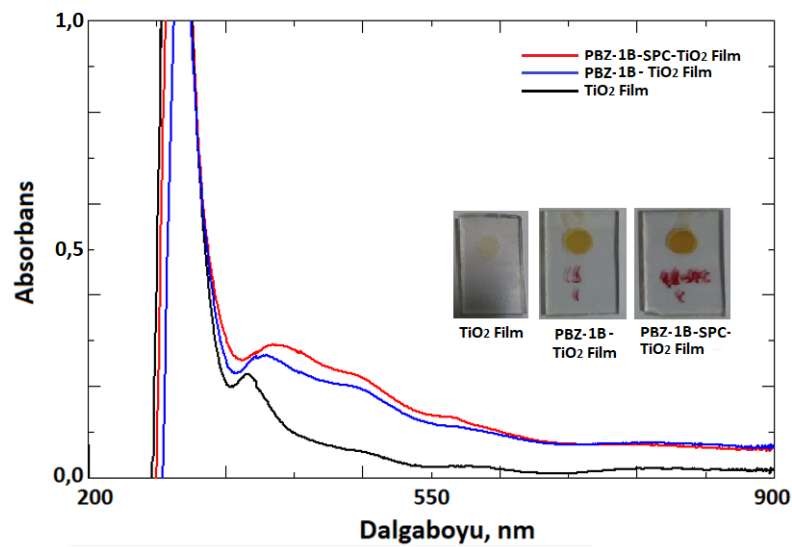
Şekil 8.3. \text{TiO}_2 , PBZ-1B- \text{TiO}_2 ve PBZ-1B-SPC- \text{TiO}_2 katı filmleri için UV-Vis Spektrumu.
