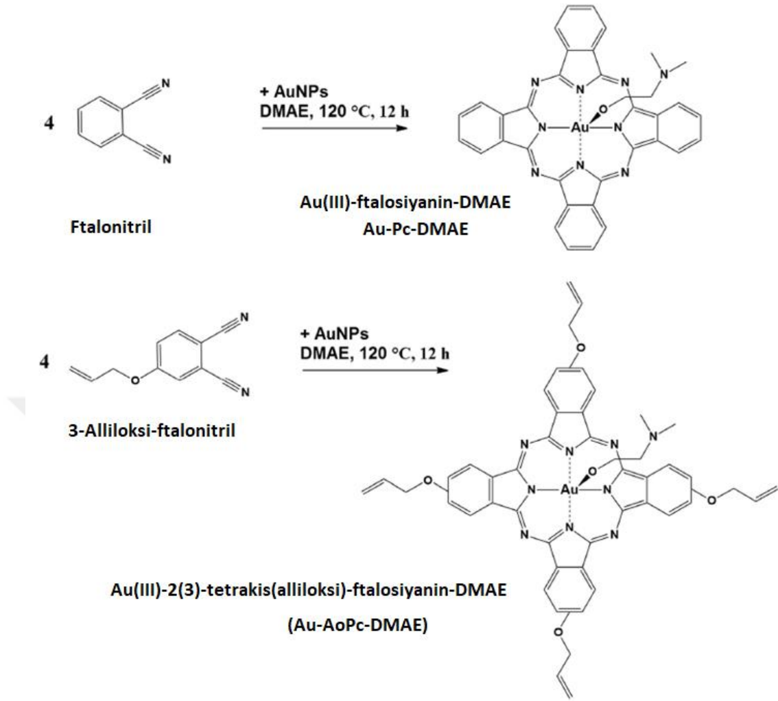
Şekil 2.9. Au-PC ve Au-AoPC kompleksleri sentez reaksiyonu [73].
