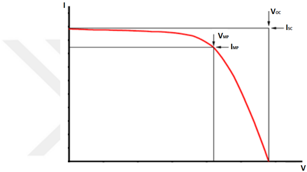
Şekil 3.5. Akım yoğunluğu-potansiyel eğrisi [129].
