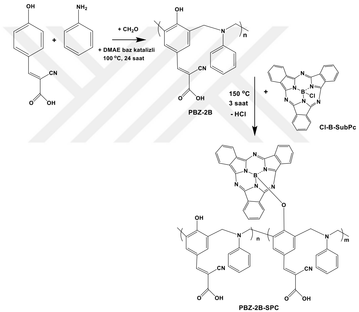
Şekil 7.24. PBZ-2B-SPC sentez reaksiyonu.
