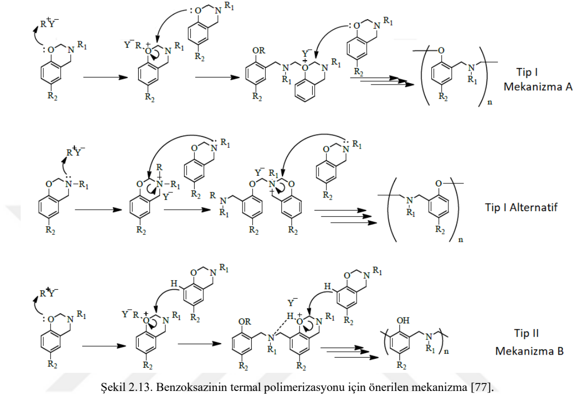
Şekil 2.13. Benzoksazinin termal polimerizasyonu için önerilen mekanizma [77].
