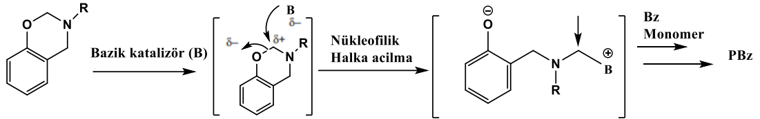
Şekil 2.11. Baz katalizörü ile halka açılma reaksiyon mekanizması [74].
