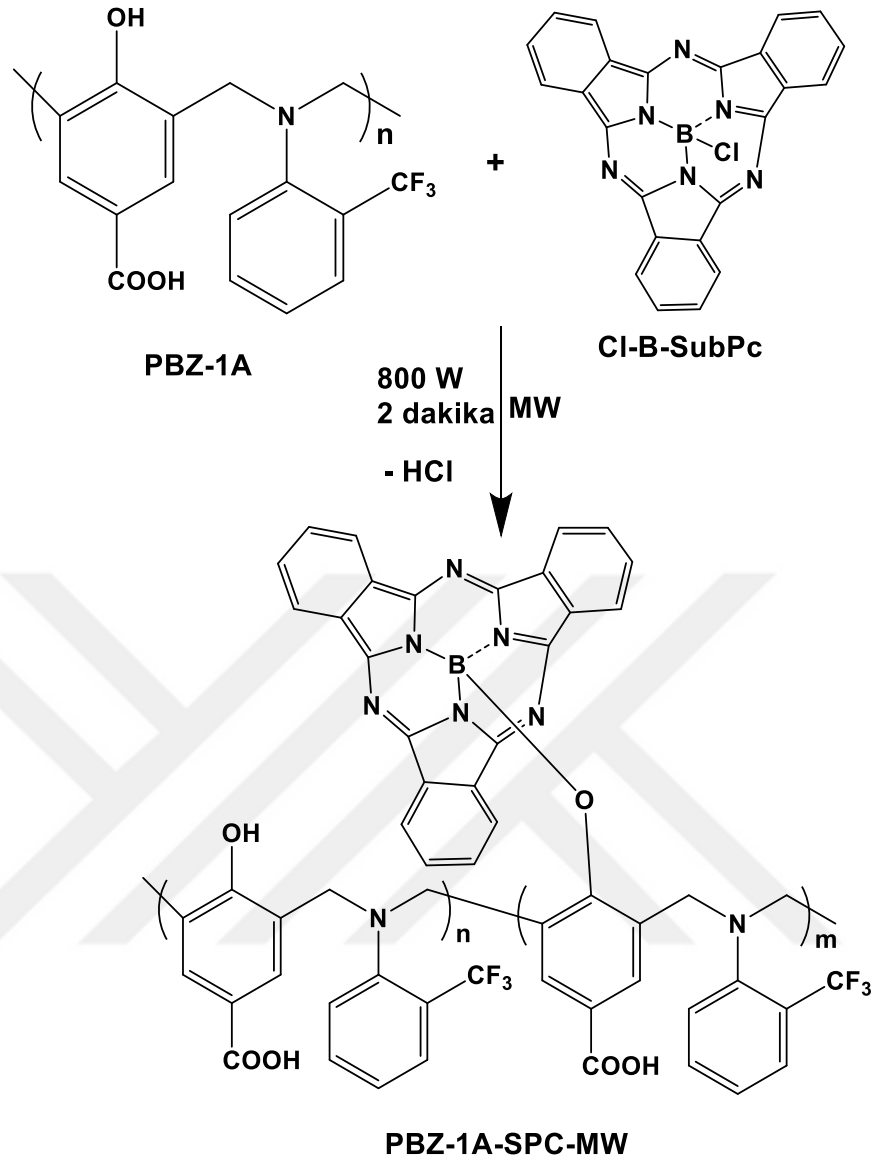
Şekil 7.31. PBZ-1A-SPC-MW mikrodalgalı sentez reaksiyonu.
