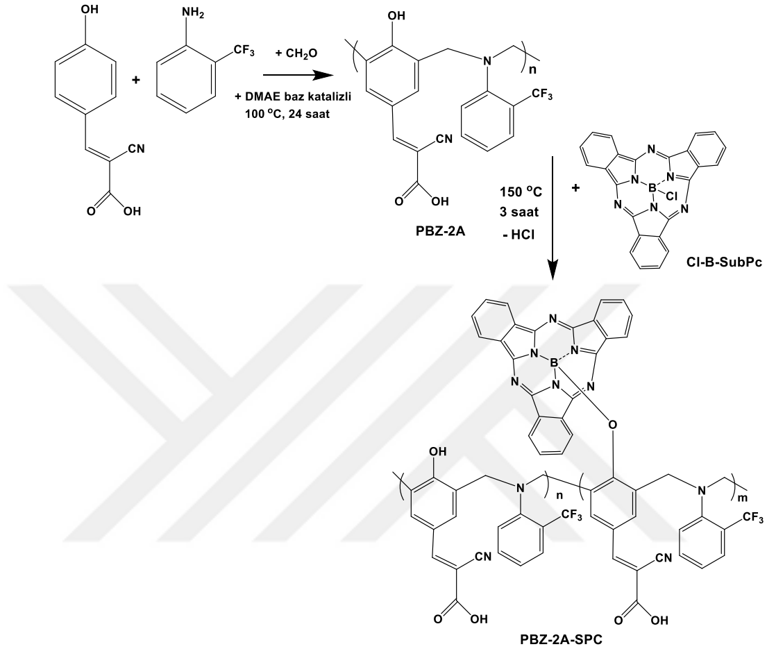
Şekil 7.10. PBZ-2A-SPC sentez reaksiyonu.
