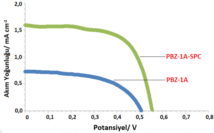
Şekil 8.8. PBZ-1A ve PBZ-1A-SPC polimerik boyalarına ait potansiyel-akım yoğunluğu grafiği.
