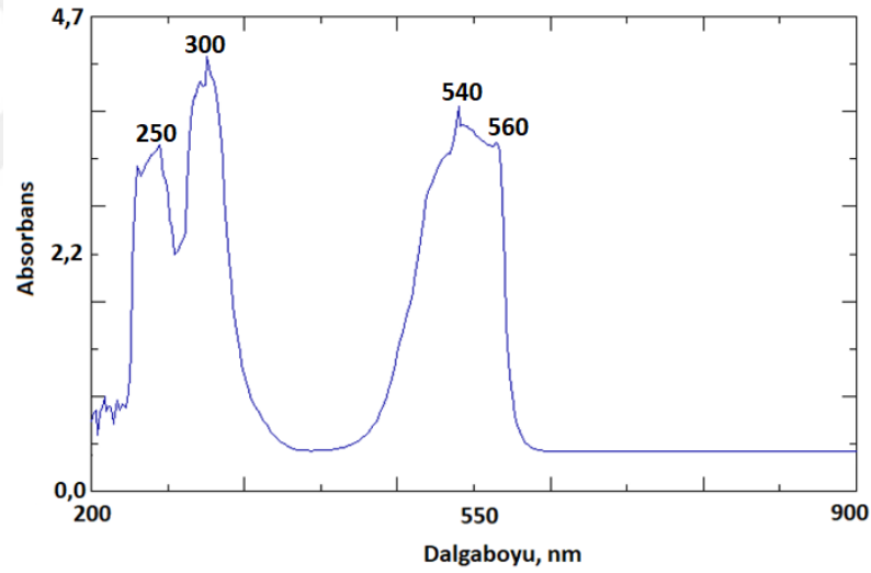
Şekil 7.1. SPC için THF çözeltisinin UV-Vis spektrumu.
