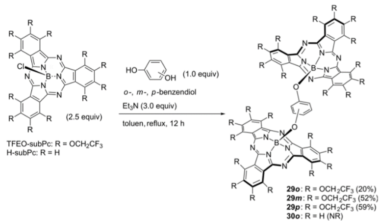
Şekil 2.15. Trifloroetoksi-subftalosiyanin benzendiol ile reaksiyonu [97].
