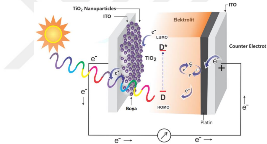
Şekil 3.6. BDGP enerji-seviye diyagramı [5].
