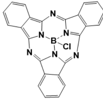
Şekil 2.14. Bor subftalosiyanin klorür molekülü.
