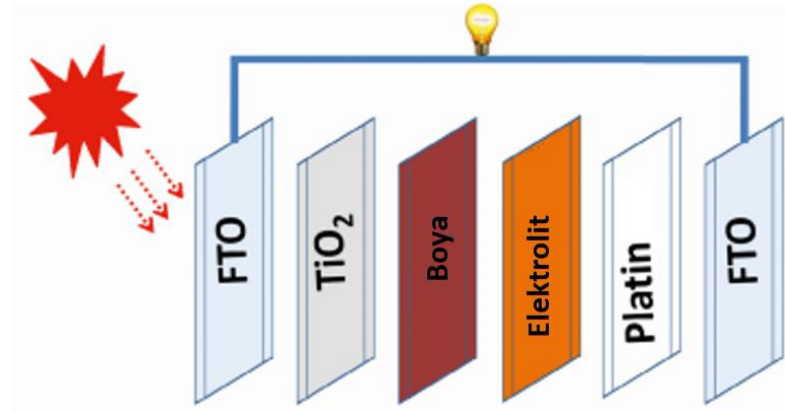
Şekil 3.4. BGDP şekilsel gösterimi [31].
