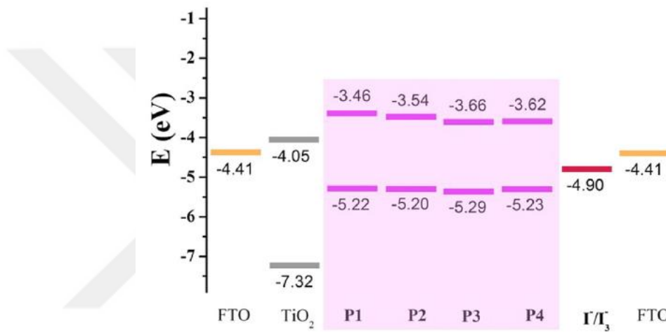
Şekil 3.9. Elektrokimyasal ve optiksel çalışmalardan elde edilen HOMO ve LUMO enerji diyagramları [132].
