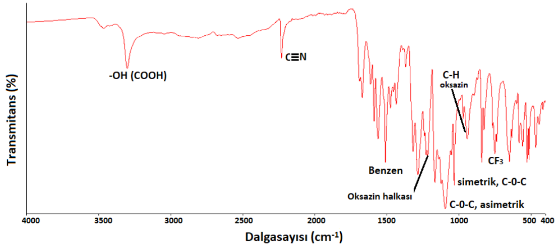
Şekil 5.5. BZ-2A monomerinin FT-IR yapı tayini.
