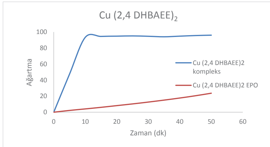
Şekil 4.7. Cu (2,4 DHBAEE) 2 kompleks ve epoksi polimerine ait %Ağartma-Zaman grafiği
