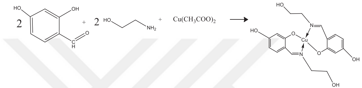
Şekil 3.5. \text{Cu}(2,4 \text{ DHBAE})_2 kompleksinin molekül yapısı
