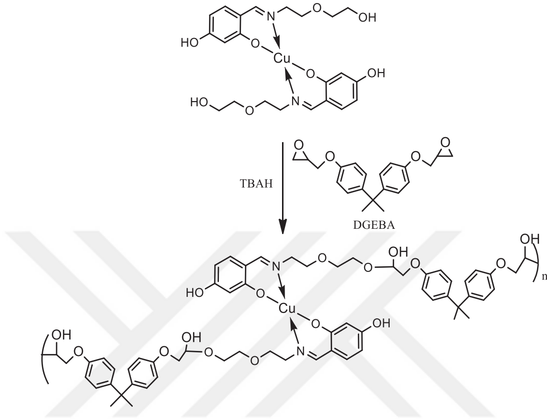
Şekil 3.9. Cu(2,4 DHBAEE) 2 epoksi polimeri sentezi
