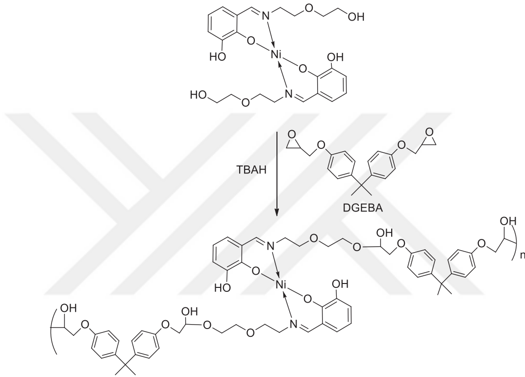
Şekil 3.8. Ni(2,3 DHBAEE) 2 epoksi polimeri sentezi
