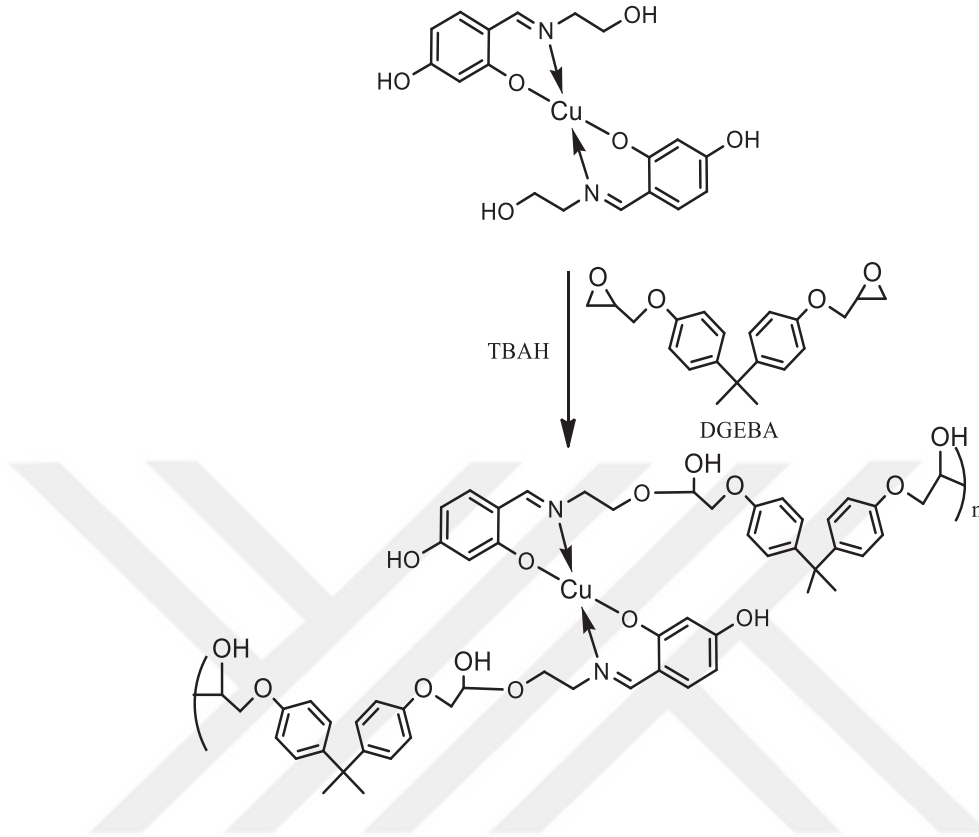
Şekil 3.11. Cu(2,4 DHBAE) 2 epoksi polimeri sentezi
