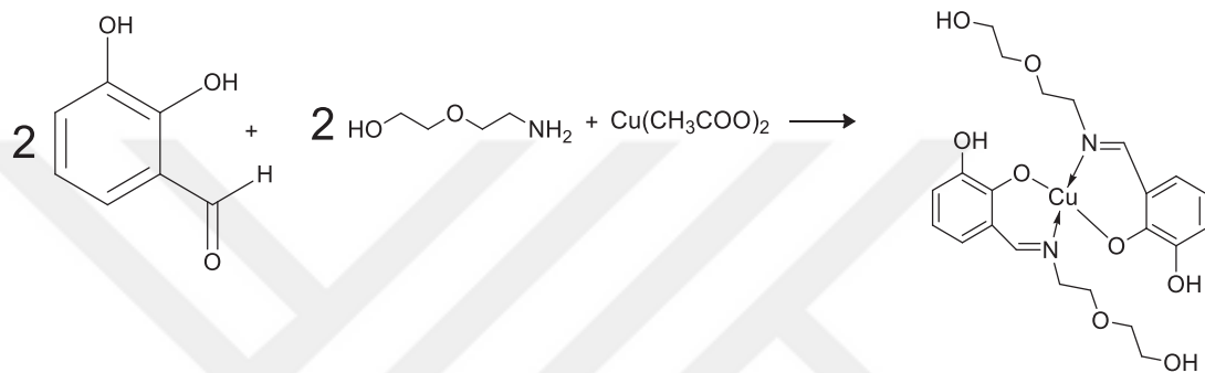
Şekil 3.1. \text{Cu}(2,3\text{DHBAEE})_2 kompleksinin molekül yapısı
