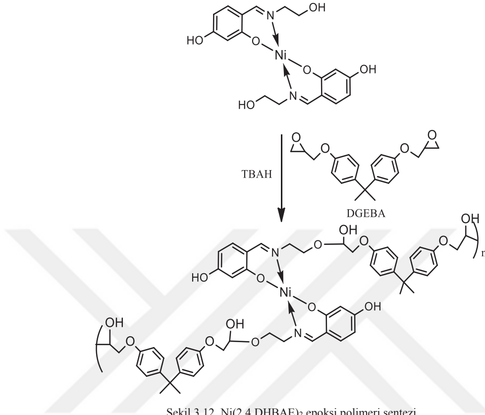
Şekil 3.12. Ni(2,4 DHBAE) 2 epoksi polimeri sentezi
