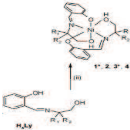
Şekil 2.12. Di-nükleer kompleksleri
