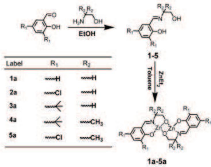
Şekil 2.14. Çinko-Salen kompleksi
