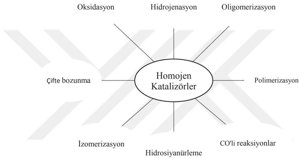
Şekil 2.4. Homojen geçiş metalli katalitik endüstriyel reaksiyonlar
