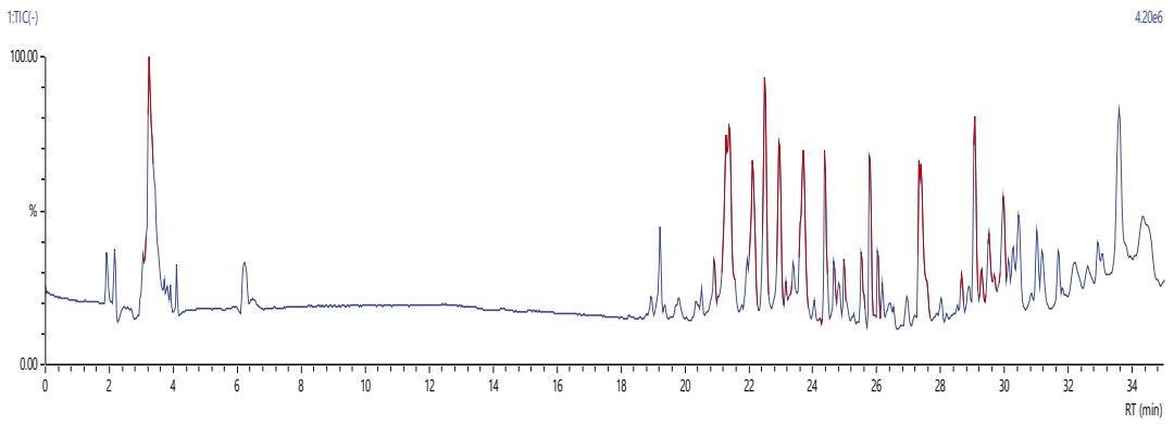
Şekil 4.22. P. major jacq. bitkisinin yaprak etanol ekstralarının negatif iyon LCMS kromotogramı
