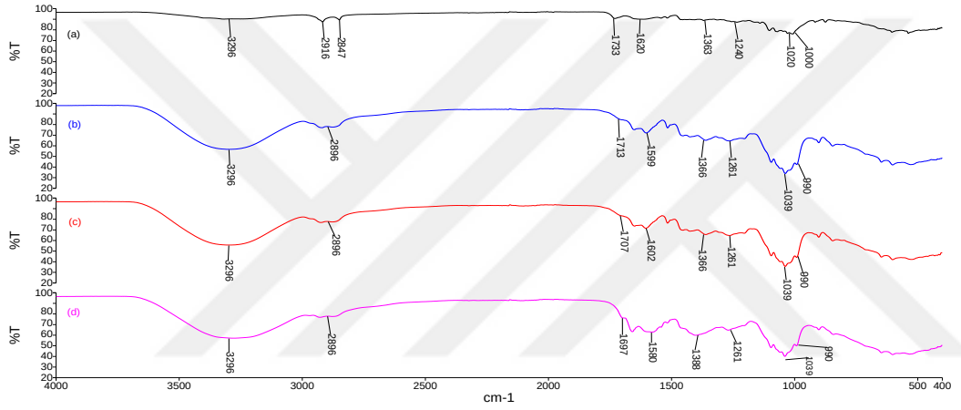
Şekil 4.14. P. major jacq. yaprak (a) ve yaprak ekstraktlarının (aseton (b), etanol (c), ve metanol (d)) FTIR spektrumu.
