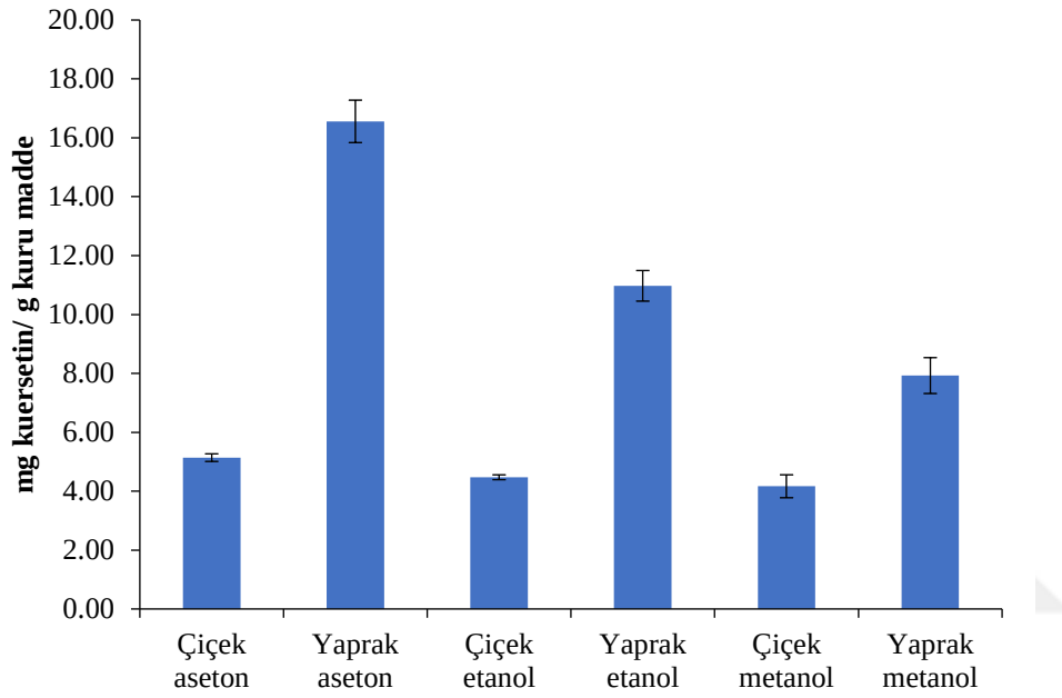
Şekil 4.5. P. major jacq. bitkisinin çiçek-yaprak aseton, etanol ve metanol ekstratlarının toplam flavonoid madde miktarları
