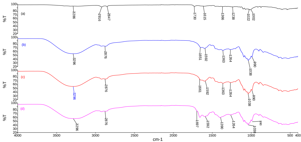
Şekil 4.15. P. major jacq. çiçek (a) ve çiçek ekstraktlarının aseton (b), etanol (c), ve metanol (d) FTIR spektrumu.
