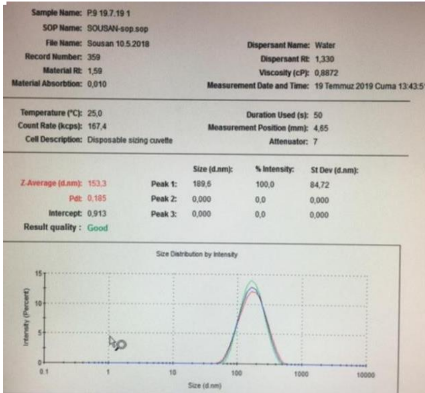
Şekil 4-17: P.9 PSC yüklü mikroemülsiyonun partikül büyüklüğü ve PDI dağılımı grafiği
