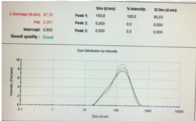
Şekil 4-16: P.8 PSC yüklü mikroemülsiyonun partikül büyüklüğü ve PDI dağılımı grafiği
