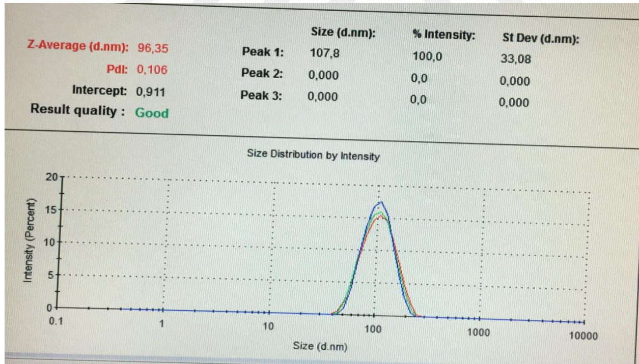
Şekil 4-14: P.1 PSC yüklü mikroemülsiyonun partikül büyüklüğü ve PDI dağılımı grafiği
