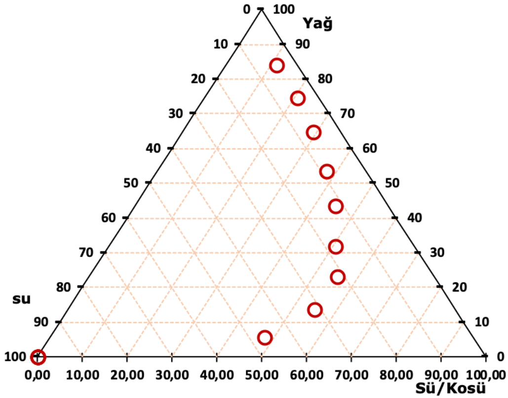
Şekil 4-10: Oleik asit, Tween 20 ve Transcutol P (1:1) içeren mikroemülsiyona ait üçgen faz diyagramı
