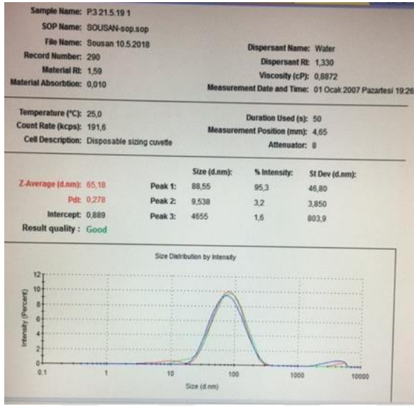
Şekil 4-15: P.3 PSC yüklü mikroemülsiyonun partikül büyüklüğü ve PDI dağılımı grafiği
