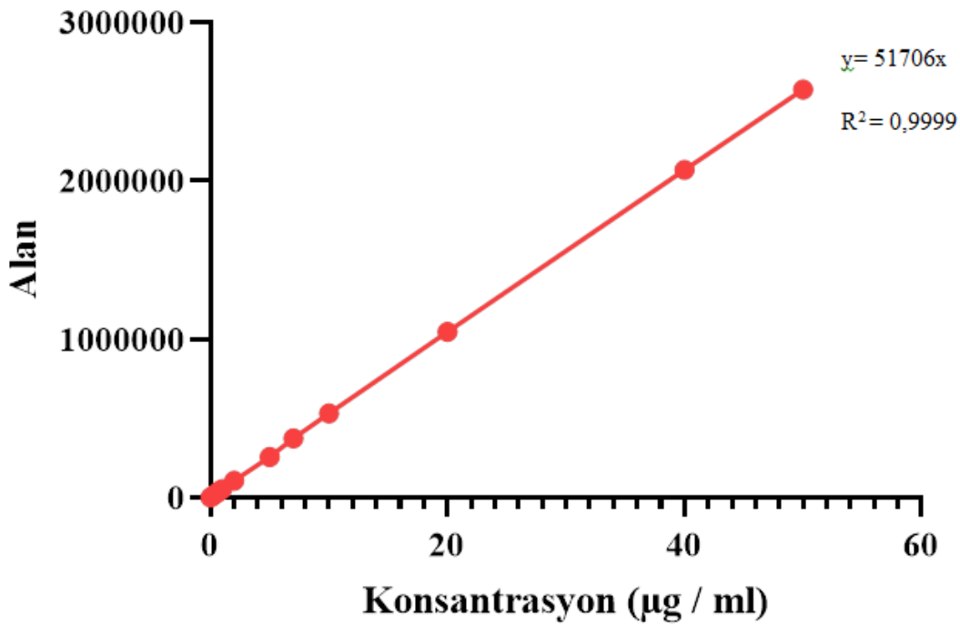
Şekil 4-4: PSC'nin kalibrasyon doğrusu ve denklemi
