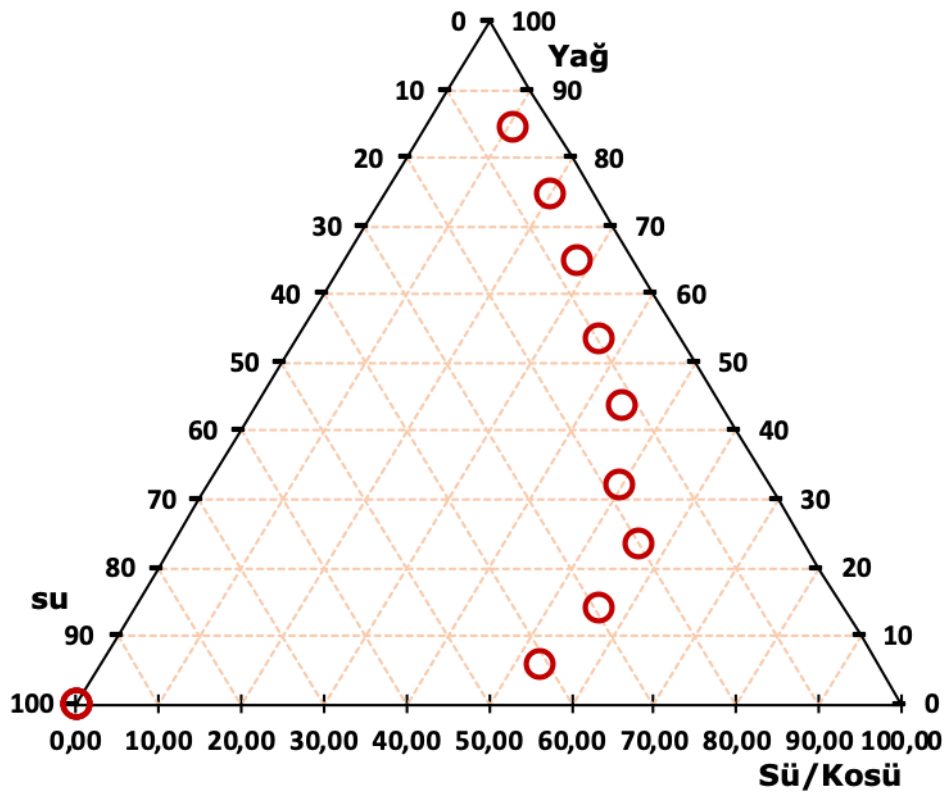
Şekil 4-9: Yağ fazı Oleik asit, Labrasol ve Transcutol P oranı 1:1 olan mikroemülsiyonlara ait üçgen faz diyagramı
