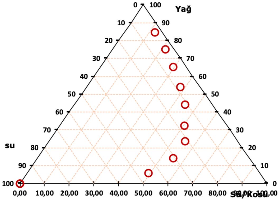
Şekil 4-11: Oleik asit yağ fazı olarak, Labrasol-Cremophor El:Transcutol P oranı 1:1 olan mikroemülsiyonlara ait üçgen faz diyagramı
