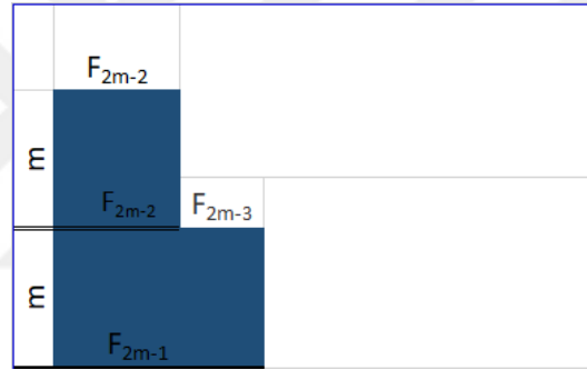
Şekil 4.5. 1 \odot P_m ve 1 \oplus P_m kümeleri tarafından oluşturulan dikdörtgenlerin boyutları.
