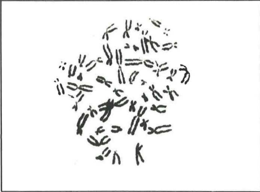
Şekil 21. Kromatid kırık.
