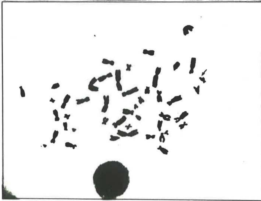
Şekil 35. Delesyon.
