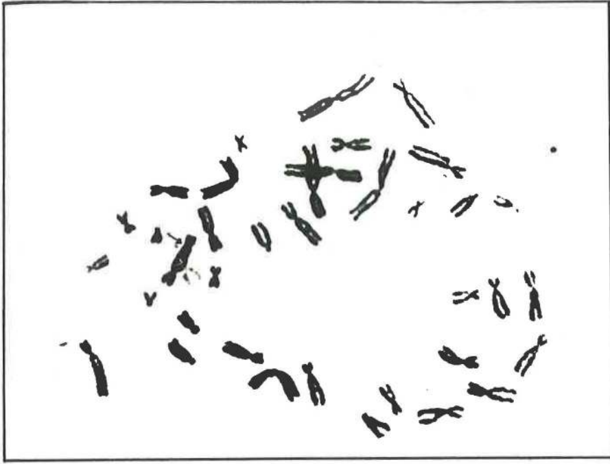
Şekil 34. Disentrik kromozom.
