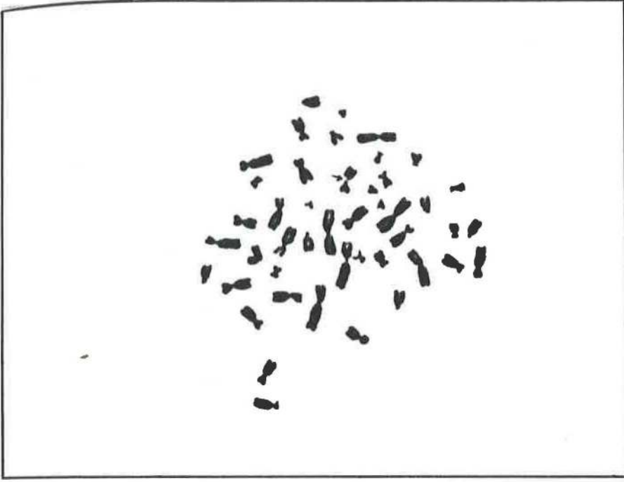
Şekil 36. İzokromatid kırık.
