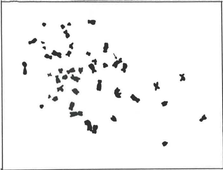
Şekil 19. Kromatid kırık.
