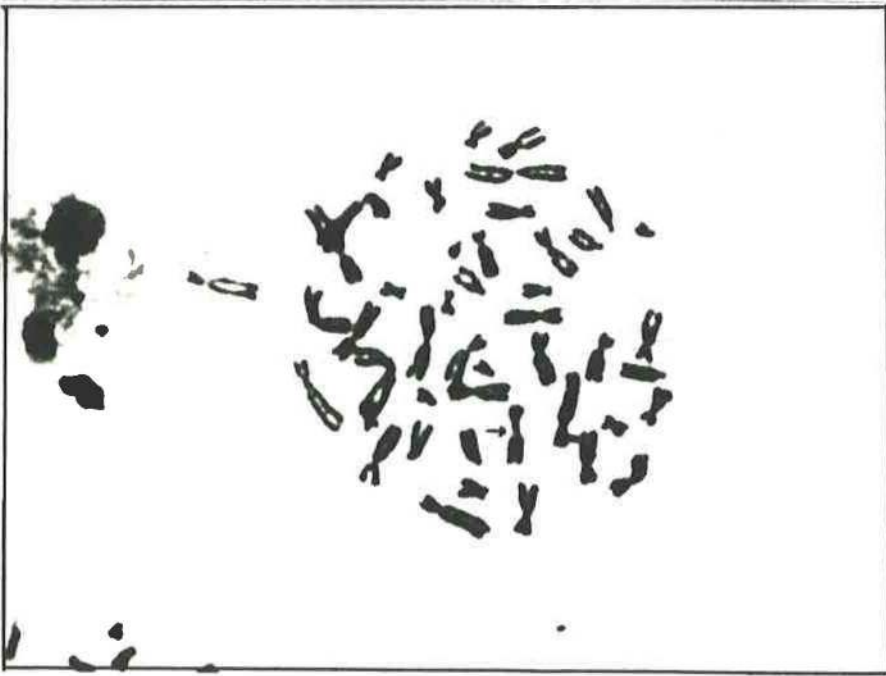
Şekil 37. İzokromatid gap.
