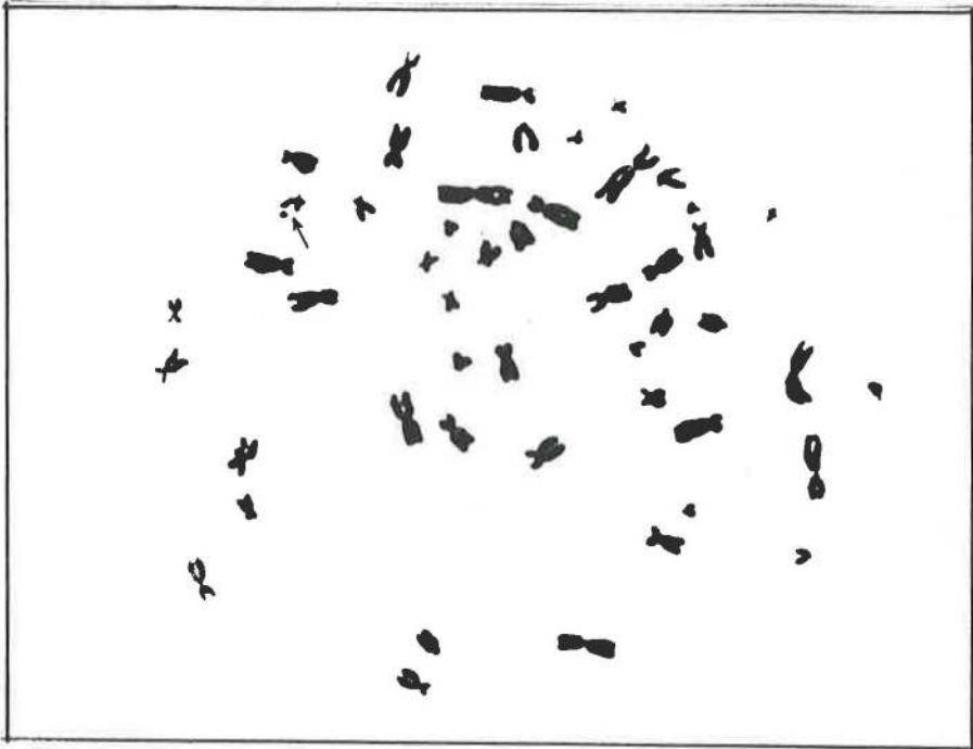
Şekil 15. Kromatid kırık.
