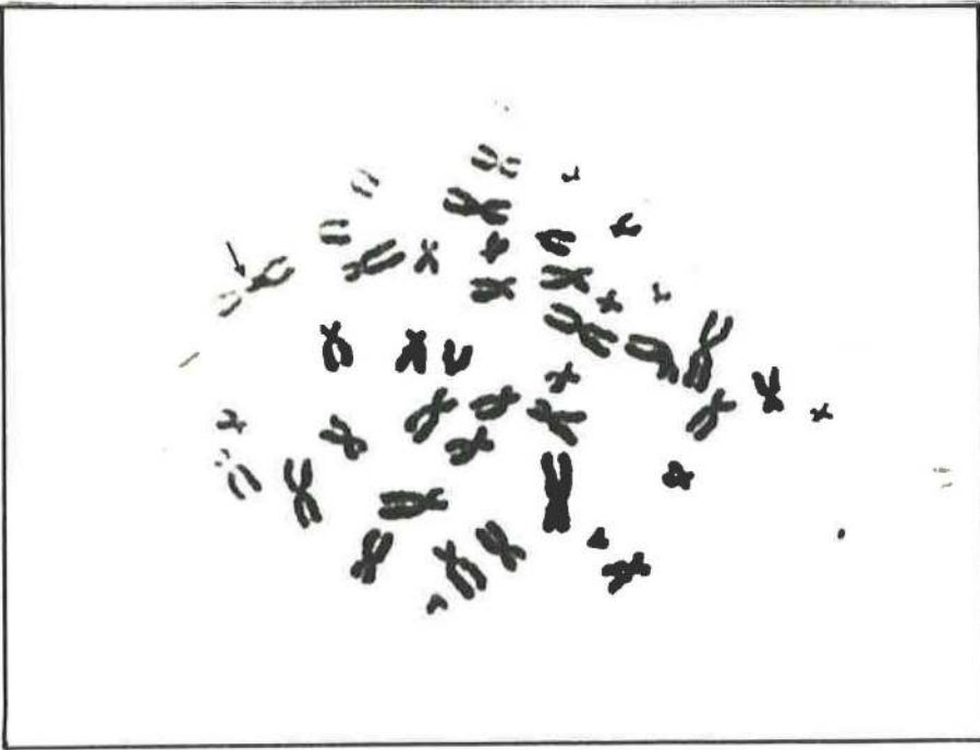
Şekil 33. Disentrik kromozom.
