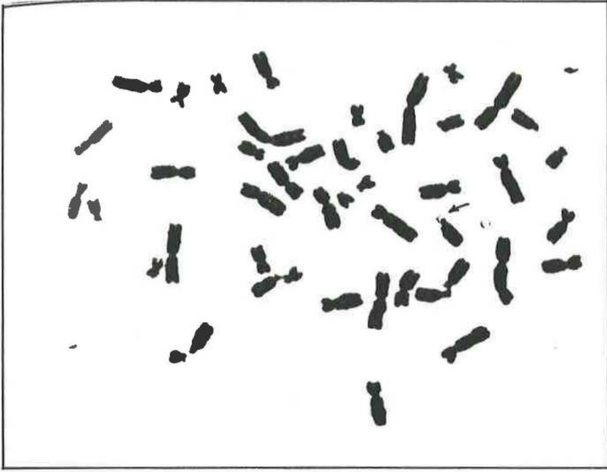
Şekil 32. İri satellit.
