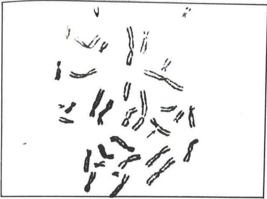
Şekil 18. Kromatid gap.
