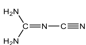
dicyandiamide (DDA)
