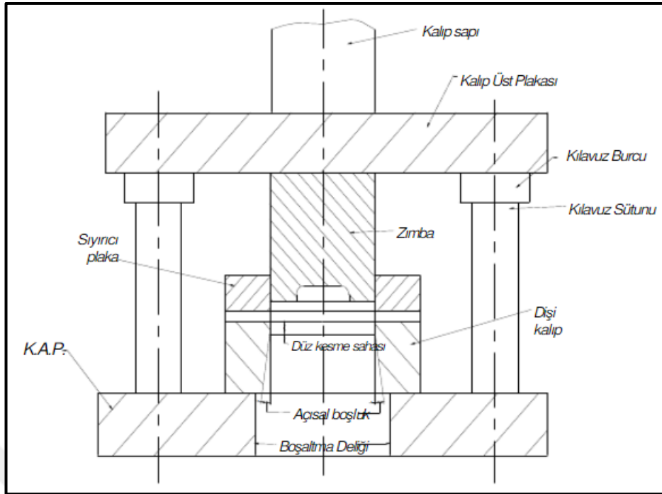
Şekil 4.1. Kesme kalıbı ve ana parçaları ( https://tr.scribd.com )
