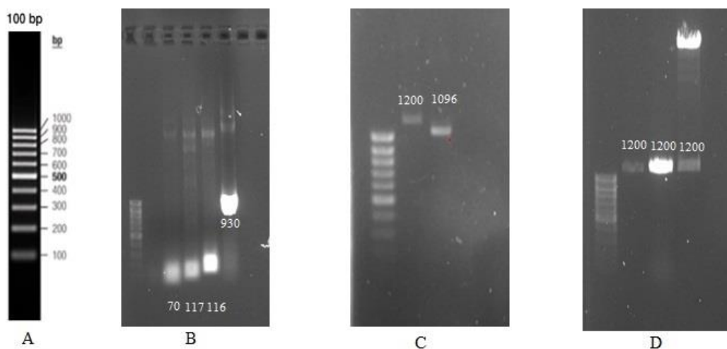
Figure 3.7. T. cuspidata GGPPS gene.
