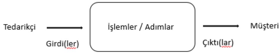
Şekil 1. Süreç Şeması
