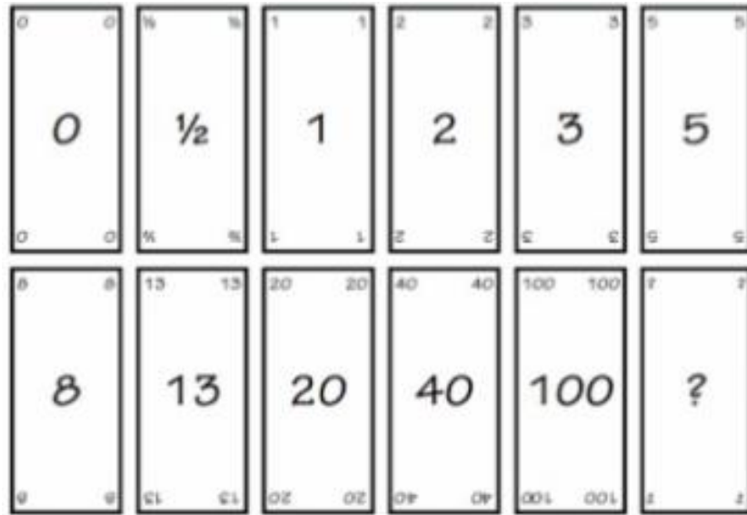
Şekil 25. Planlama Kartları
