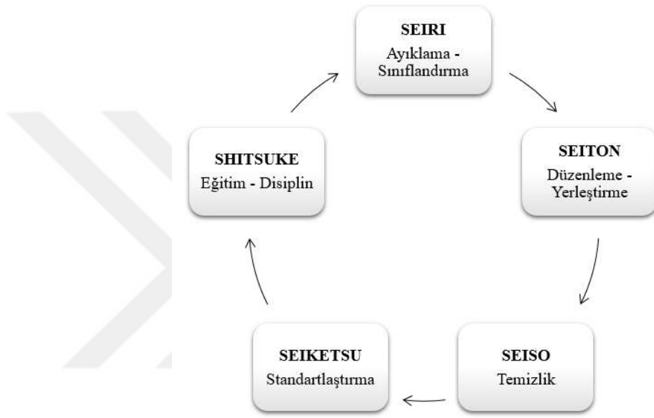
Şekil 33. 5S sistemi
