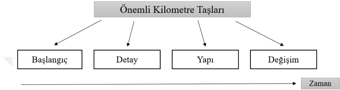
Şekil 20. RUP Fazları
