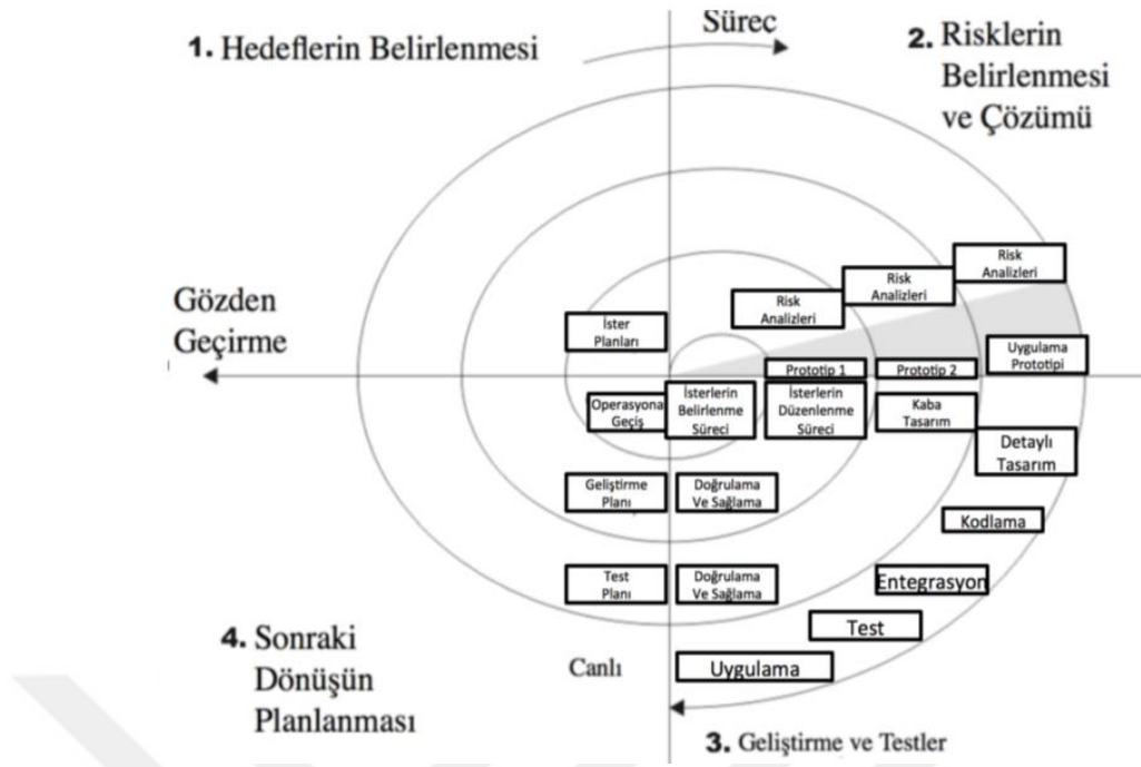
Şekil 18. Spiral Model
