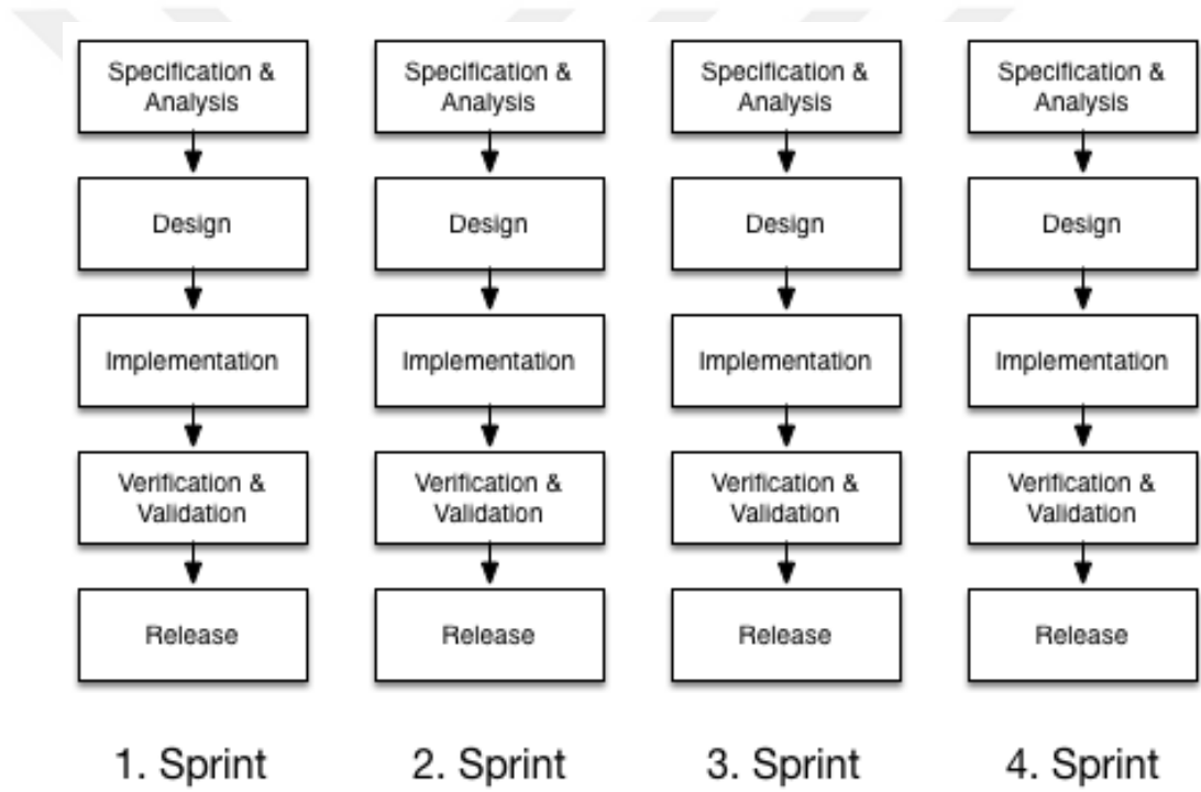
Şekil 24. SCRUM Sprintleri
