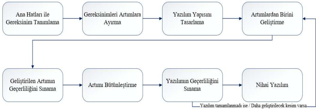
Şekil 16. Artımsal Model
