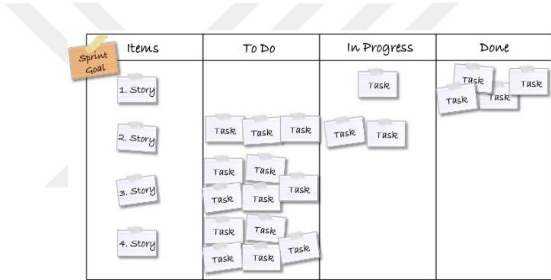
Şekil 26. SCRUM Tahtası
