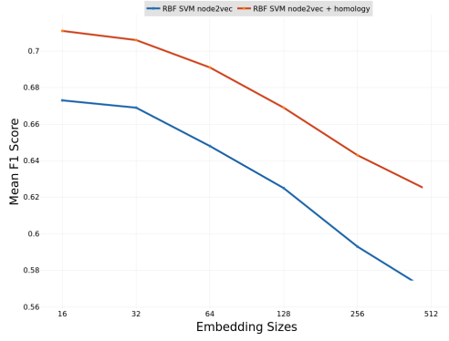
(b) F1 plot of RBF kernel
