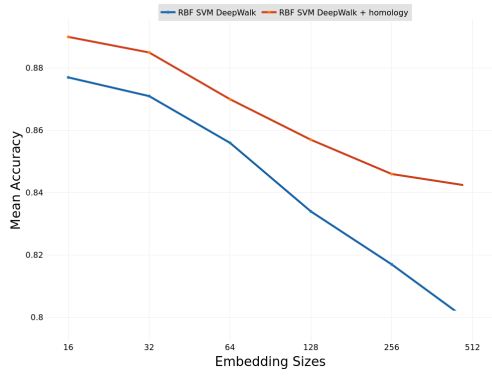
(b) RBF kernel
