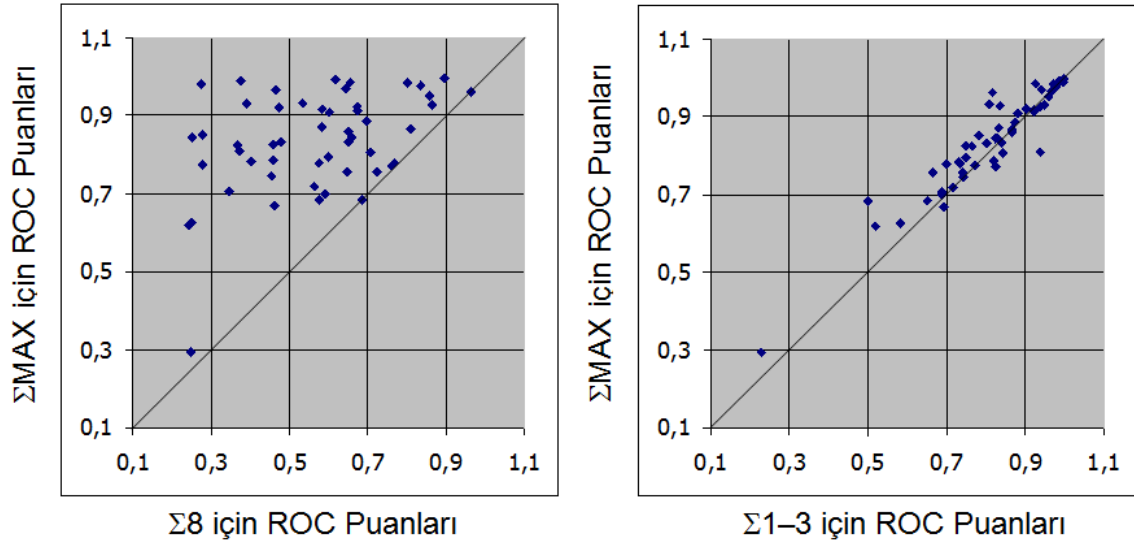
Şekil 6.26 – ΣMAX’a karşı Σ8(a), Σ1-3(b)
