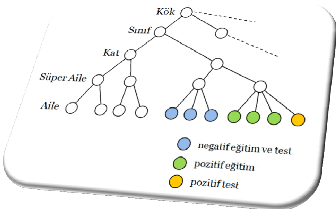
Şekil 5.4.2.1 – Uzak Homoloji Tespitinin SCOP Veritabanı Hiyerarşisi Üzerindeki Bir Simülasyonu
