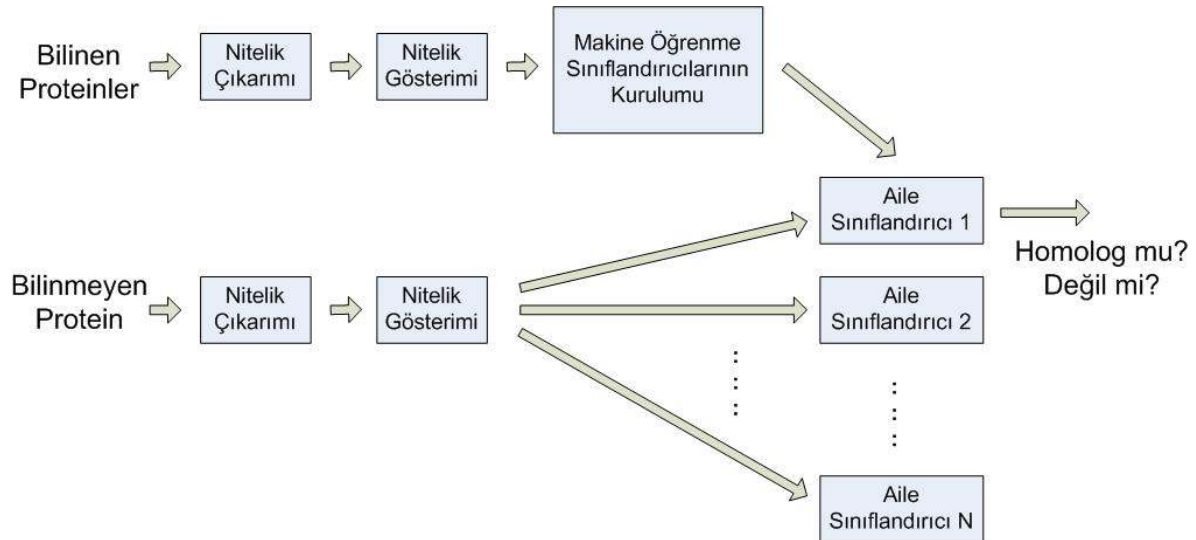
Şekil 5.3.1 – Fark Gözeten Homoloji Tespiti Modeli
