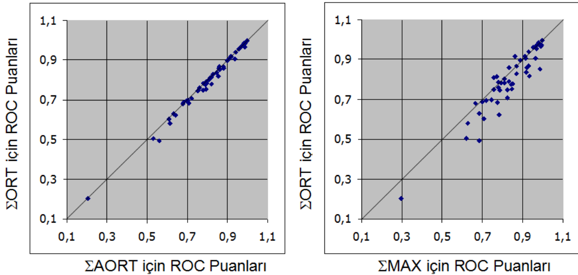
Şekil 6.27 – ΣORT’a karşı ΣAORT(a), ΣMAX(b)
