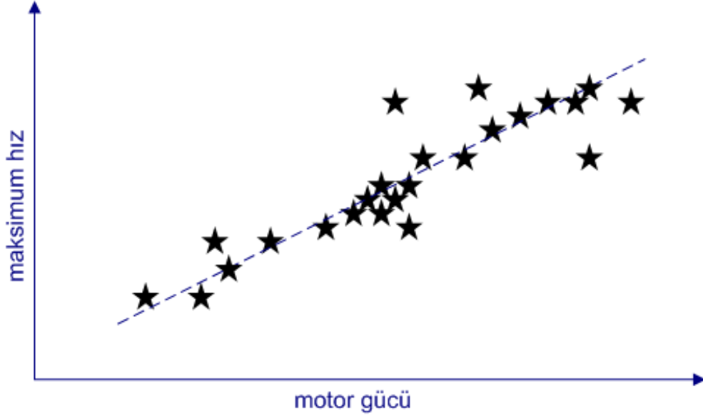
Şekil 3.1.2 – Regresyon
