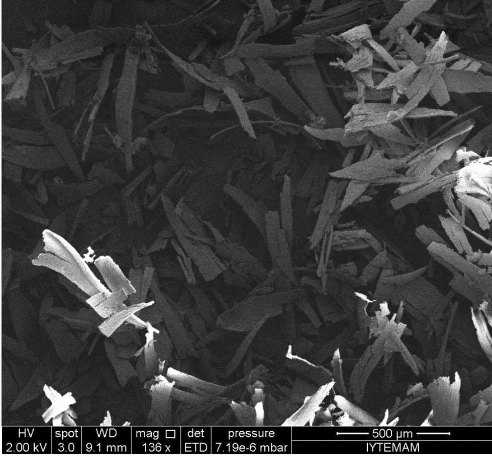
Şekil 3.10. H. cupressiforme 125 \mu\text{m} altı partiküllerin SEM ile genel görünümü (136x büyütme)
