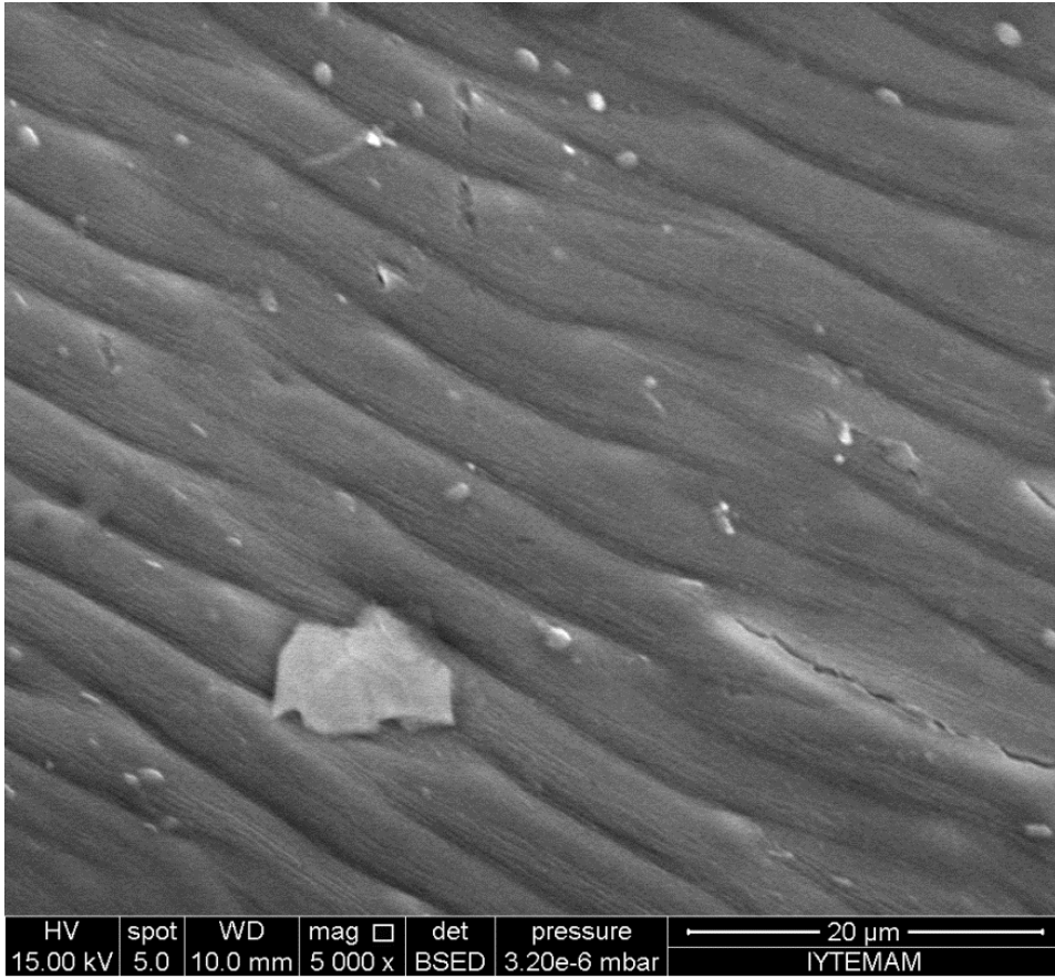
Şekil 3.13. H. cupressiforme 125 µm altı partiküllerin yüzey kıvrımlarının SEM görüntüsü (5000x büyütme)
