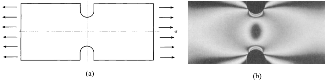
Şekil 3.1. Çekmeye zorlanan çentikli bir numune örneği (a) Meydana gelen gerilme (b) Fotoelastik Fotoğraf (Doz. Dr.-Ing. habil. K. Fethke, Universitat Rostock) [36]
