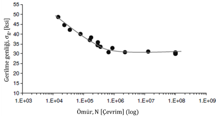
Şekil 1.8. Wöhler eğrisi [3]
