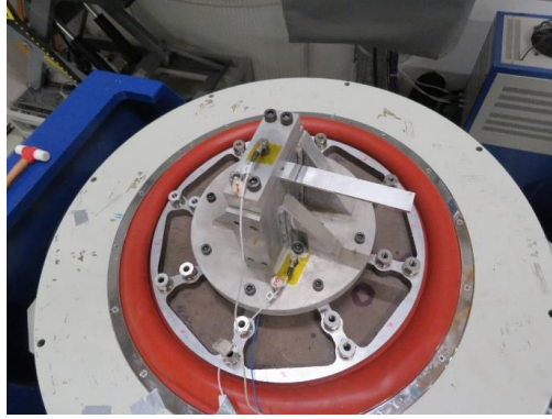
Şekil 3.27. Numunenin sarsıcı tabla testinin kurulumu [37]
