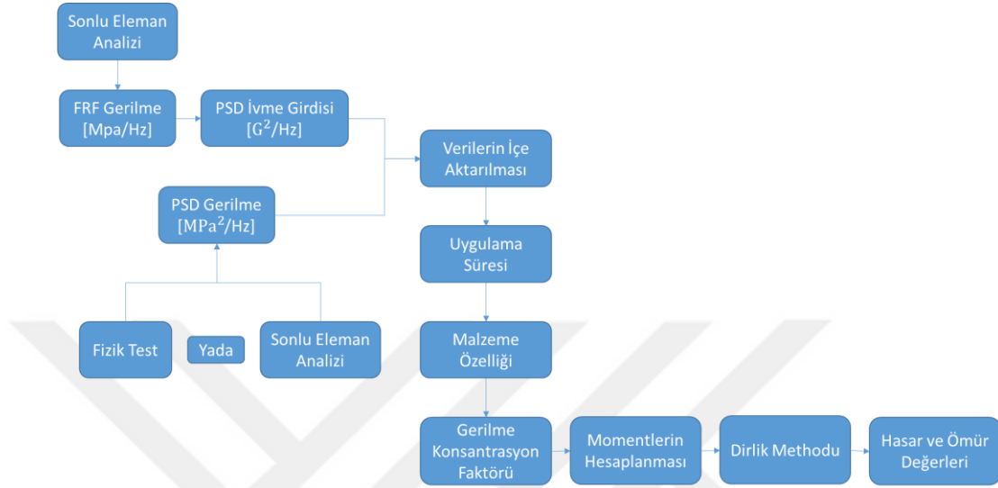
Şekil 3.26. Oluşturulan Python kodu ile hasar hesaplama iş akışı
