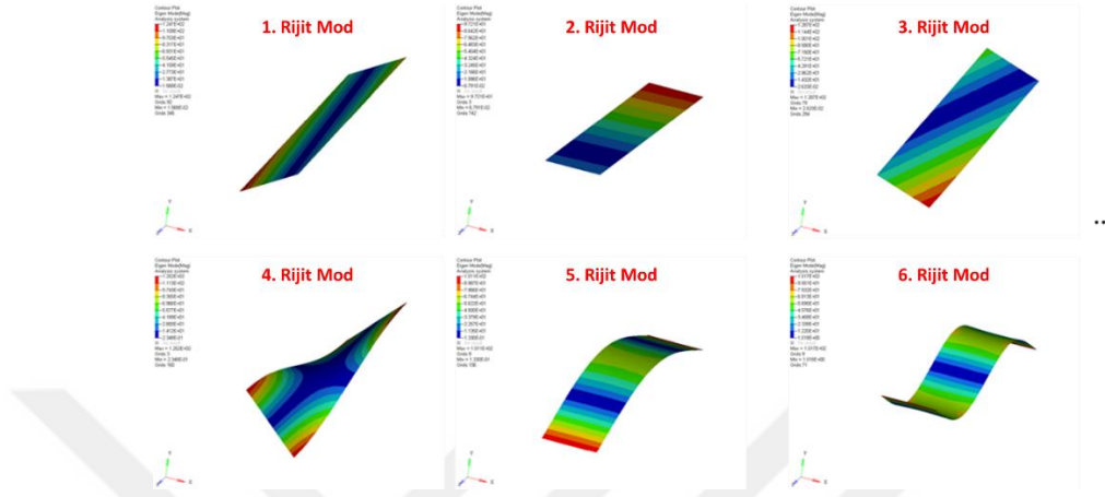
Şekil 2.8. Plakanın kısıtsız modal analizi sonucu - Rijit modları (HyperMesh - OptiStruct çözücüsü)
