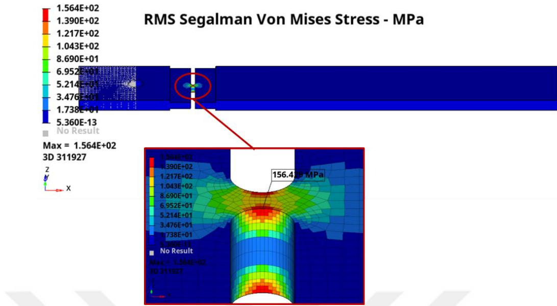
Şekil 3.9. Alüminyum numunenin RMS segalman von mises gerilmesi [MPa]
