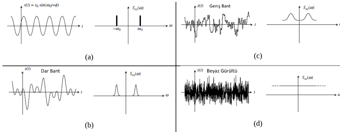
Şekil 2.16. Rastgele sinyal türleri [28]
