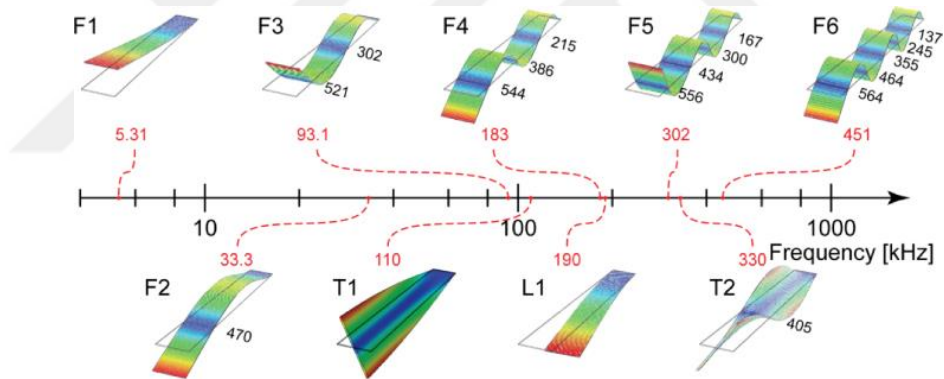
Şekil 2.9. Plakanın kısıtlı olarak gerçekleştirilen modal analiz sonucu (HyperMesh-OptiStruct çözücüsü)
