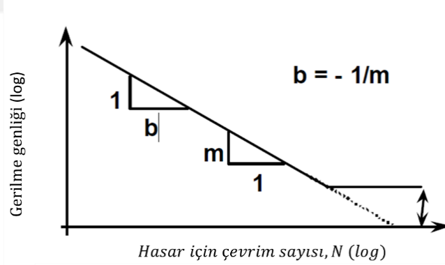
Şekil 2.20. SN Eğrisi [7]
