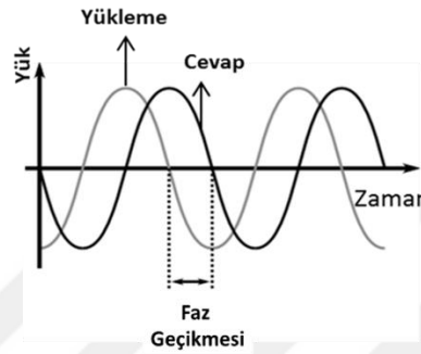
Şekil 2.11. Yükleme ile cevap arasındaki faz geçikmesi [23]
