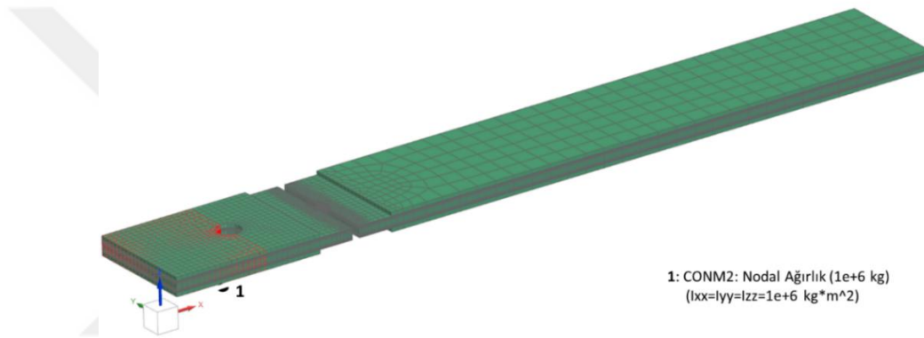
Şekil 3.17. Simcenter 3D yazılımında modal analiz tanımlamaları (Large Mass Yöntemi)
