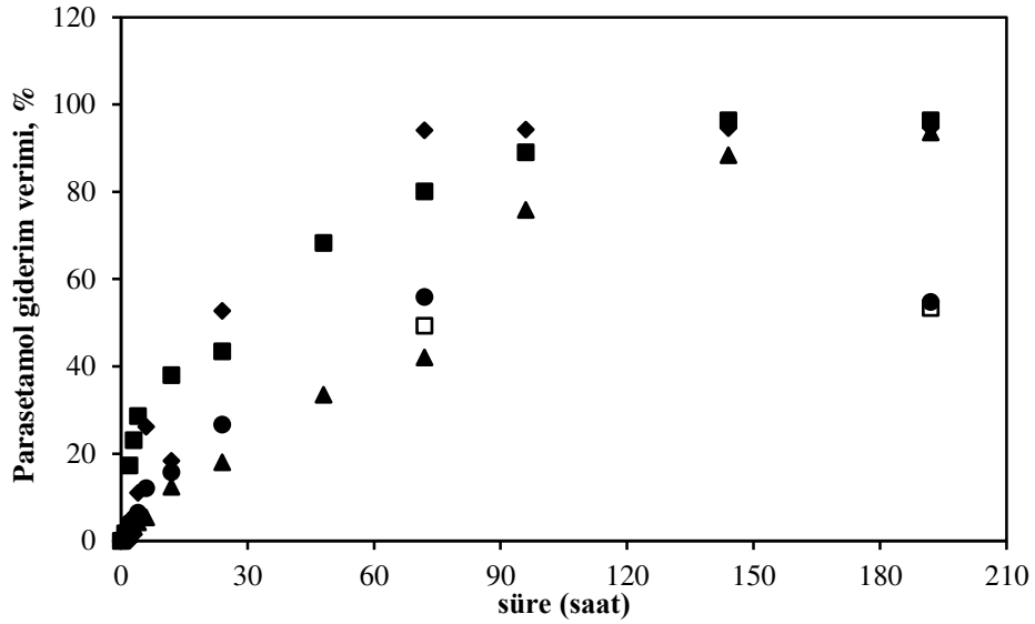
Şekil 6.19. Farklı etkiler altında parasetamol giderimi (parasetamol kons: 10 mg/L, BMO: 5 g/L, pH: 7, ♦: otoklav ile muamele, ■: NaN 3 ile muamele, ▲: işlemsiz, ●: P. putida , □: P. putida +Otoklav)
