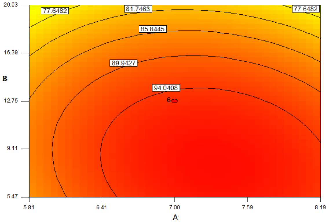
Şekil 6.18. Parasetamol giderim veriminde; pH (A) ve parasetamol konsantrasyonu (B) ve biyojenik mangan oksit miktarının (C) etkisini gösteren üç boyutlu ve iki boyutlu tepki yüzey eğrileri
