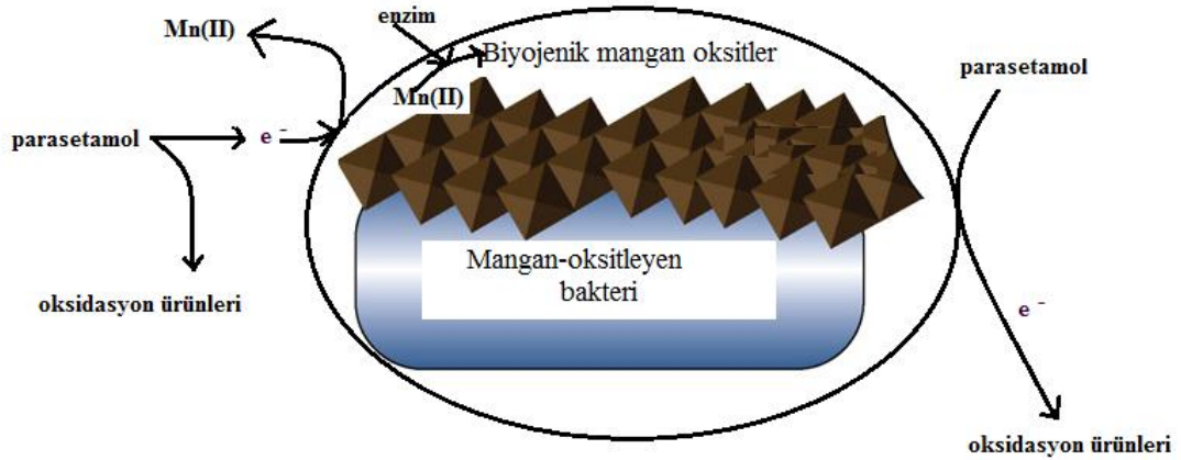
Şekil 6.20. Biyogenik mangan oksitlerle parasetamol gideriminin şematik gösterimi
