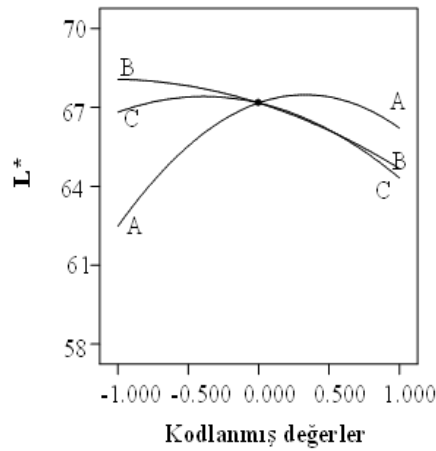
Şekil 4.17 L^* değeri için bağımsız işlem değişkenlerinin etkisini gösteren pertürbasyon grafiği (A: Şişirilme sıcaklığı, B: Şişirilme süresi, C: Vakum sıcaklığı)
