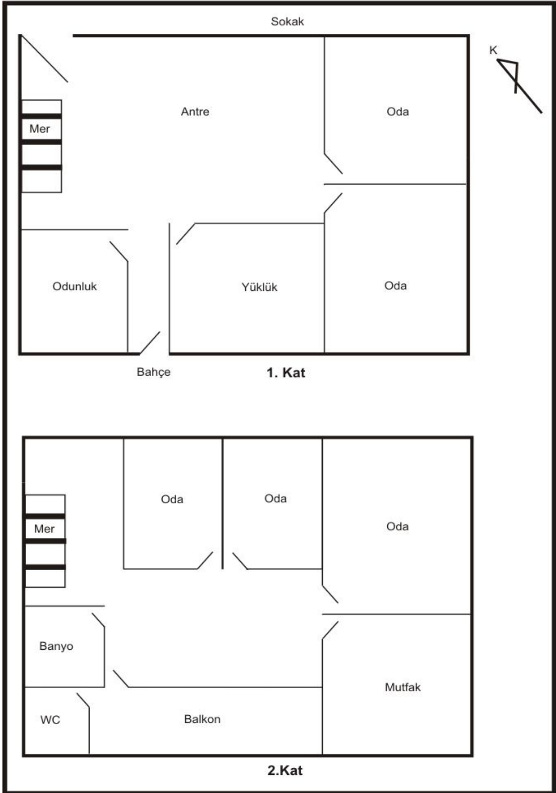
Şekil 4.14: Pütürge Kasabası'nda Geleneksel Konut Planı
