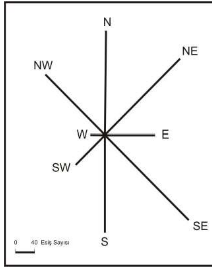
Şekil 2.2: Pütürge'nin Yıllık Ortalamalara Göre Rüzgar Güllü Diyagramı
