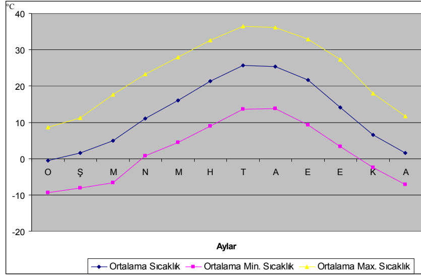
Şekil 2.1: Pütürge'nin Aylara Göre Ortalama Sıcaklık, Ortalama Minimum Sıcaklık, Ortalama Maksimum Sıcaklık ve Aylık Ortalama Yağış Grafiği
