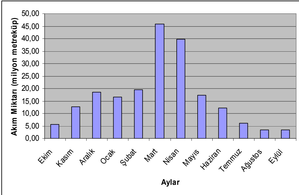
Şekil 2.7: Şiro Çayı'nın Taşıdığı Su Miktarının Aylara Göre Ortalama Dağılışı (2006-2009)
