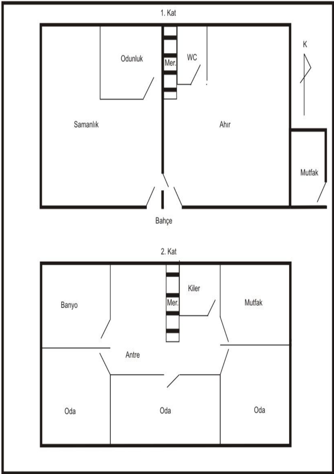
Şekil 4.9: Geleneksel Bir Köy Meskeninin Konut Planı (Aktarla Köyü)
