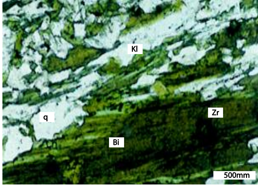
Şekil 5.5. Biyotitistlerdeki kapantı olarak görülen radyasyon hasarlı zirkon minerali. Biyotit (Bi), zirkon (Zr), kuvars (q), klorit (Kl) T.NX40 (Erdem, 1994).
