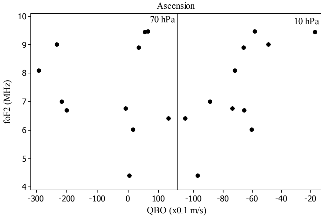
Ek Şekil A. 1. Ascension istasyonundan elde edilen foF2 kritik frekans verileri ile QBO nun serpilme diyagramı
