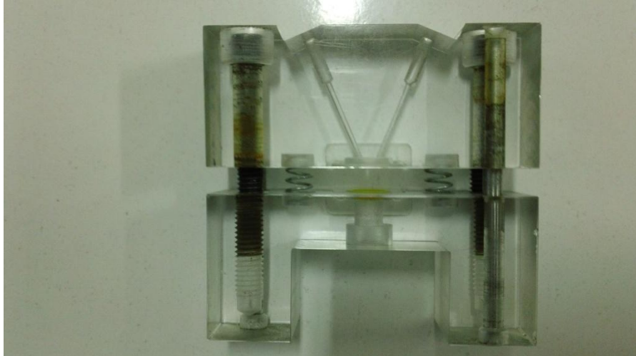
Ek-4 2 Akış hücresi
