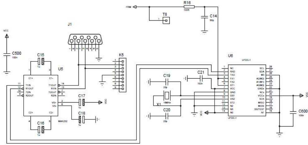
Şekil 3.13 Haberleşme devresi.
