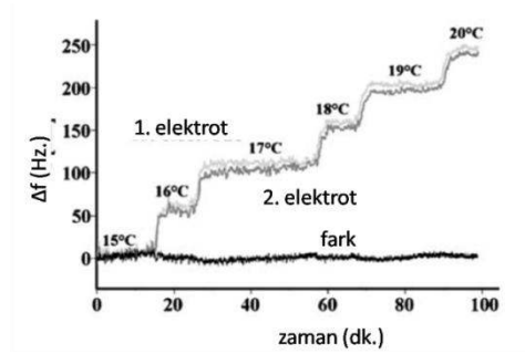
Çizelge 2.2 QCM’in 15-20 °C arasında frekans değişimleri [25]
