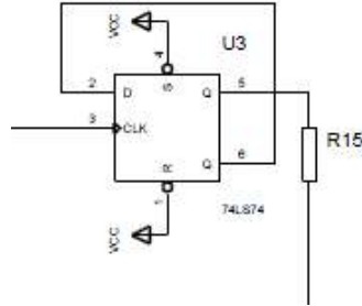
Şekil 3.12 Frekans bölücü devresi.
