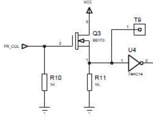
Şekil 3.11 12V / 5V dönüştürücü devresi.
