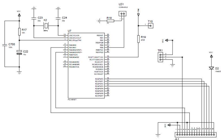
Şekil 3.9 Frekansmetre katı devre şeması.
