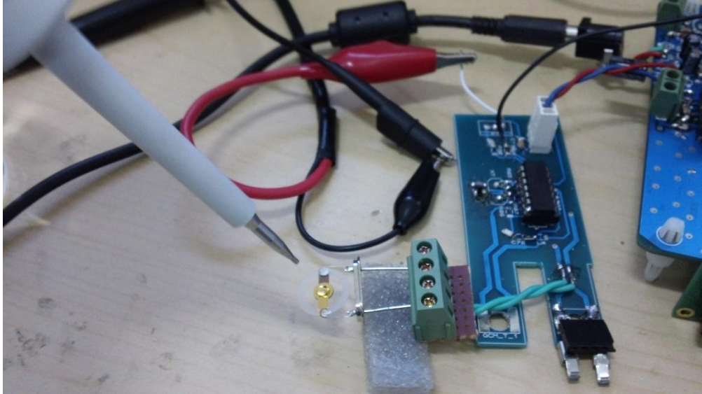
Şekil 3.4 TTL osilatör katının sıvı ortam için çalıştırılması.
