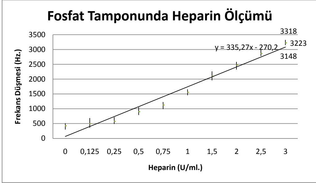
Şekil 3.15 Akış hücreinde fosfat tamponundan heparin ölçümü. Sensör cevabı y = 335,27x - 270,2 doğrusu ile belirtilmiştir.
