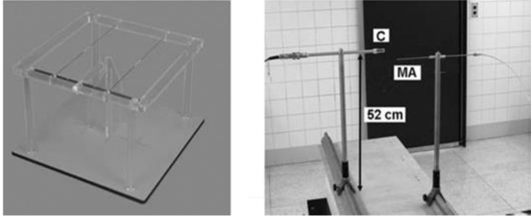
Fotoğraf 2.1. PDR ve HDR kaynakları için havadaki kalibrasyon örnekleri
