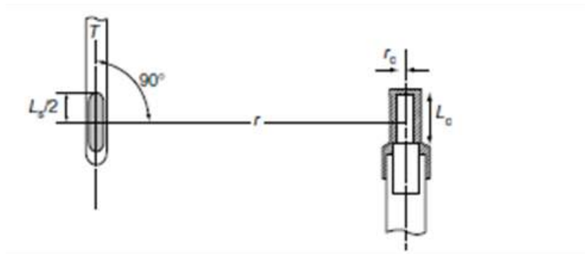
Şekil 2.1. Birikim kapaklı iyonlaşma odası kalibrasyon düzeneğinin geometrisi. (Kaynak, uygun silindirik bir bina (T) içerisine yerleştirilir. L_s , kapalı kaynağın aktif çekirdeğinin uzunluğudur ve r serbest uzaydaki hava kerma oranının ölçümü için kullanılan radikal uzaklıktır. L_c iç uzaklık iken, r_c ise bu şemada kullanılan iyonlaşma odasının tübüler kütlesinin dahili yarıçapıdır.)
