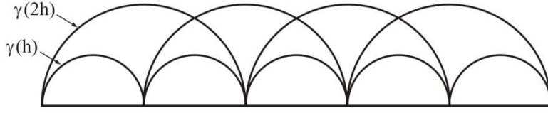
Şekil 8.1. Belirli bir uzaklık aralığındaki numuneleri kullanarak yapılan variogram hesaplamasının gösterimi
