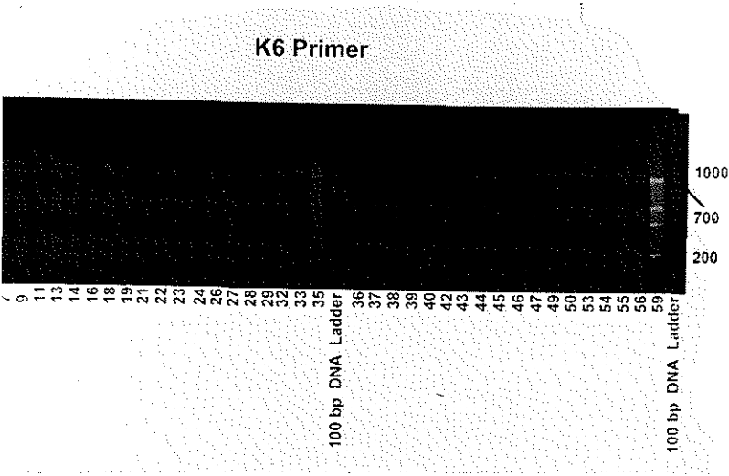
Şekil 4.5. Susam Populasyonlarında K6 Primeri ile Çoğaltılan RAPD Bant Profilleri.
