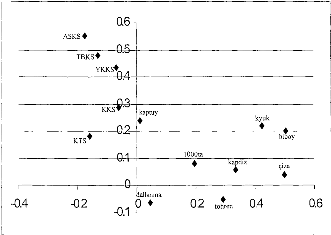
Şekil 4.1. Değişkenlerin İki Boyutlu Düzlemde Gösterilmesi
