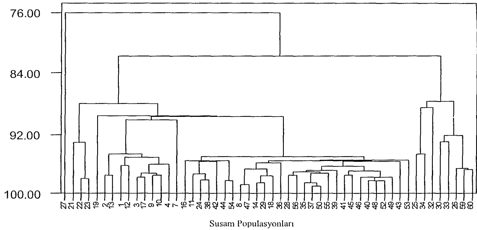
Şekil 4.2. Susam Populasyonlarının Morfolojik Özelliklerinin Öklit Uzaklığına dayanarak Yapılan Dendogramı (Numaralara ait bilgiler Çizelge 3.3'de verilmiştir).
