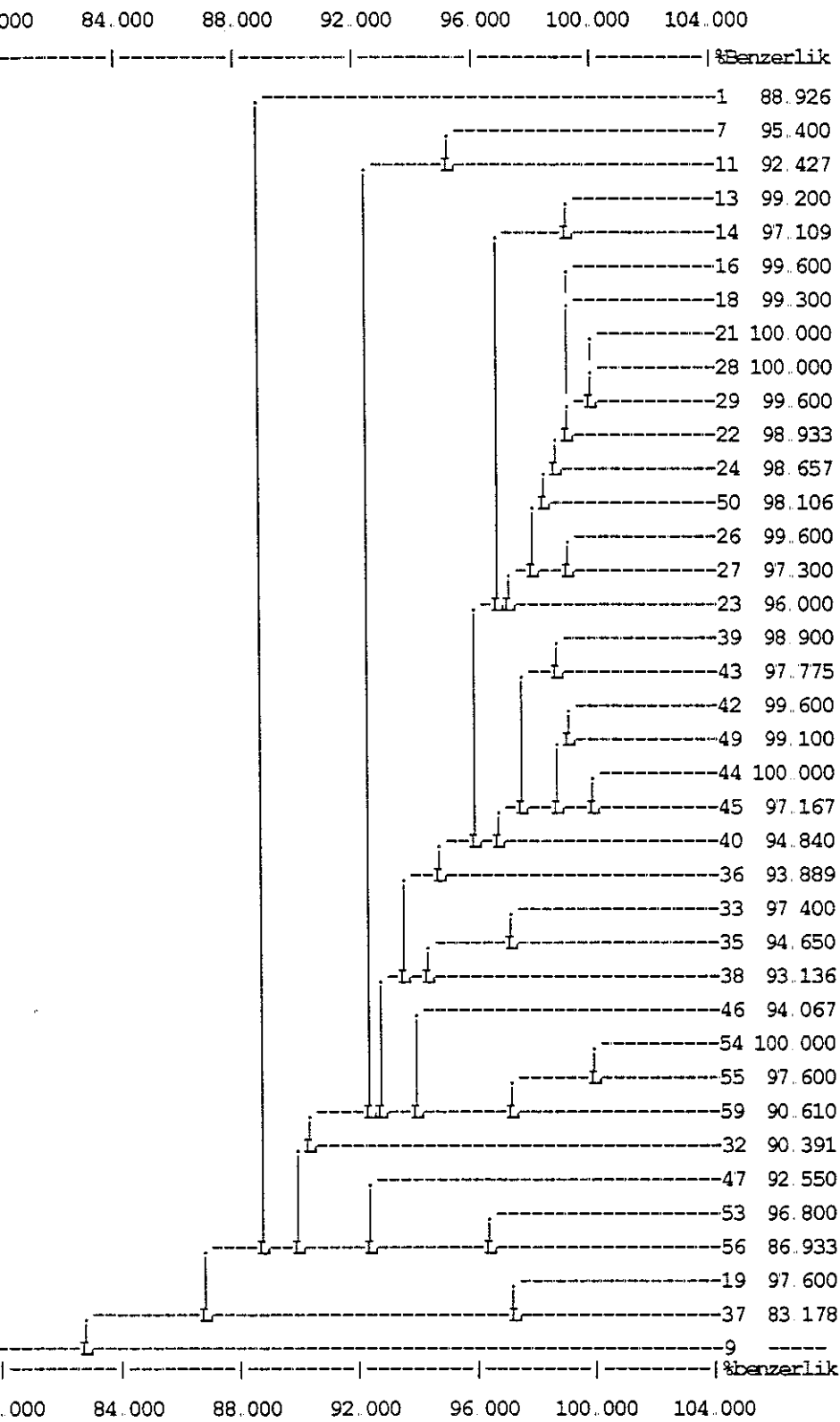
Şekil 4.7 RAPD Bant Profillerinin UPGMA ile Yapılan Dendrogramı
