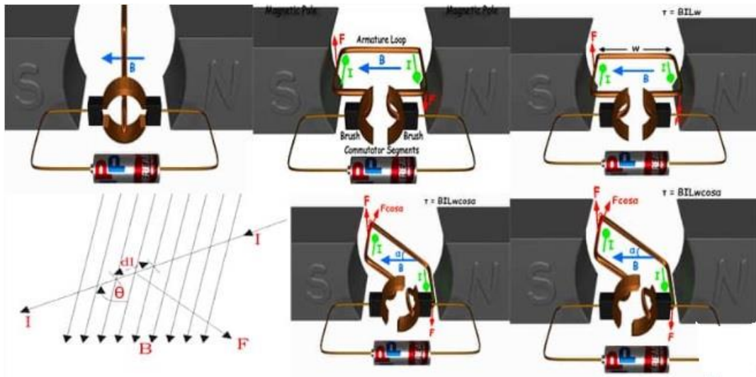
Şekil 2.16. DC Motor [30].
