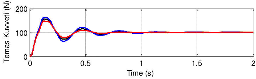
Şekil 3. 20. Farklı pantograf çerçeve sönümleme katsayısı ( c_{\text{ç}} ) değeri için temas kuvveti değişimi
