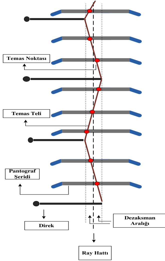
Şekil 5.3. Temas noktası değişimi
