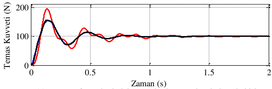
(a) Pantograf tepe kütesinin en yüksek ve en düşük değerleri için temas kuvvetlerinin karşılaştırılması
