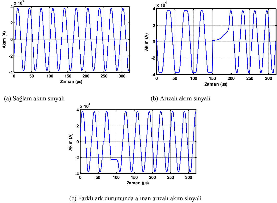
Şekil 6. 11. Model tabanlı oluşturulan sağlam ve arızalı durumlar için akım sinyalleri
