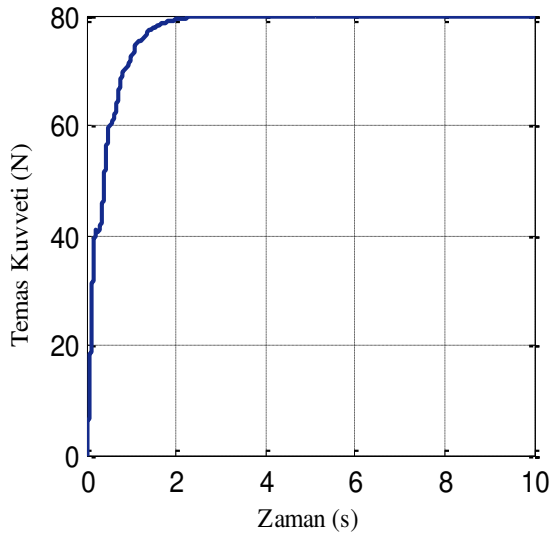
(a) 80 N'luk referans kuvveti için temas kuvveti değişimi
