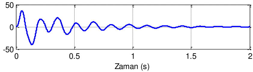
(b) Referans ve en yüksek tepe kütesi değerleri için temas kuvvetleri farkı
