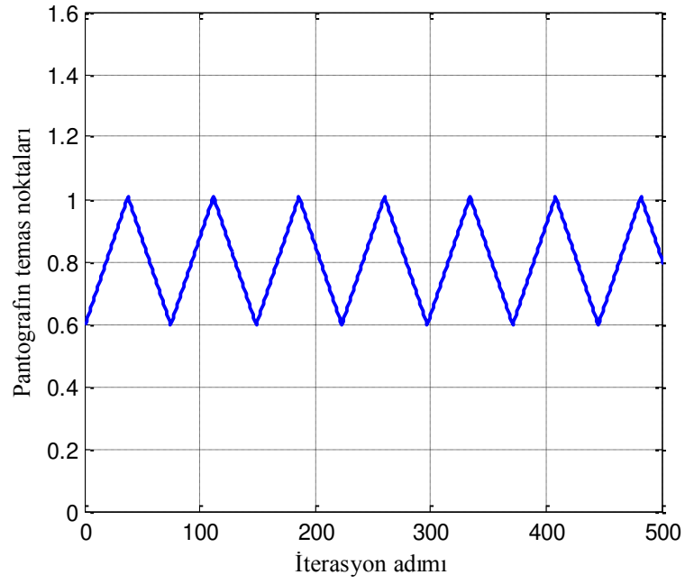
Şekil 5.6. 50 km/sa hız değeri için temas noktası değişimi
