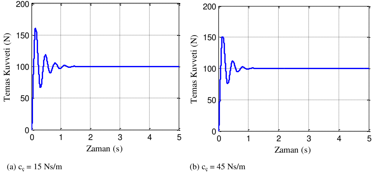
Şekil 3. 20. Farklı pantograf çerçeve sönümleme katsayısı ( c_{\text{ç}} ) değeri için temas kuvveti değişimi
