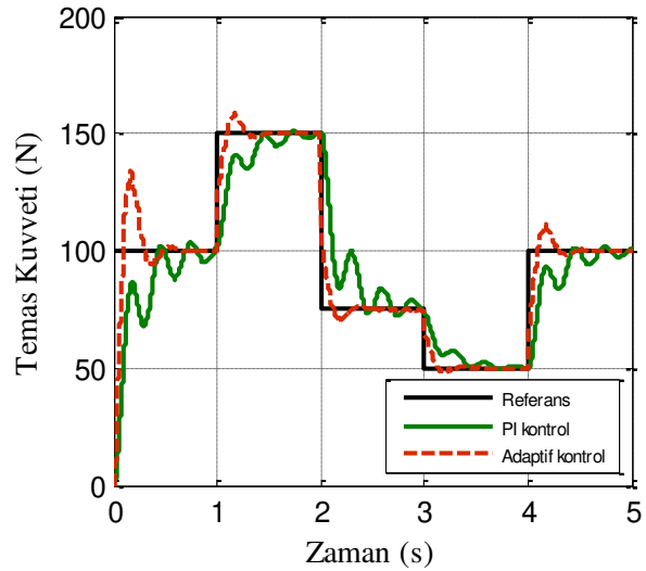
(b) Çoklu referans kuvvet değeri için temas kuvveti değişimi
