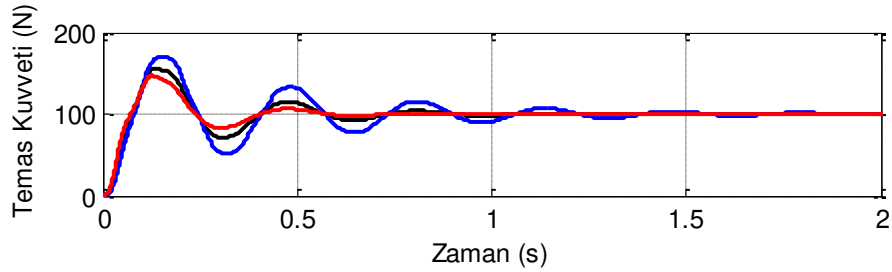
(a) Pantograf tepe sönümleme katsayısının en yüksek ve en düşük değerleri için temas kuvvetlerinin karşılaştırılması
