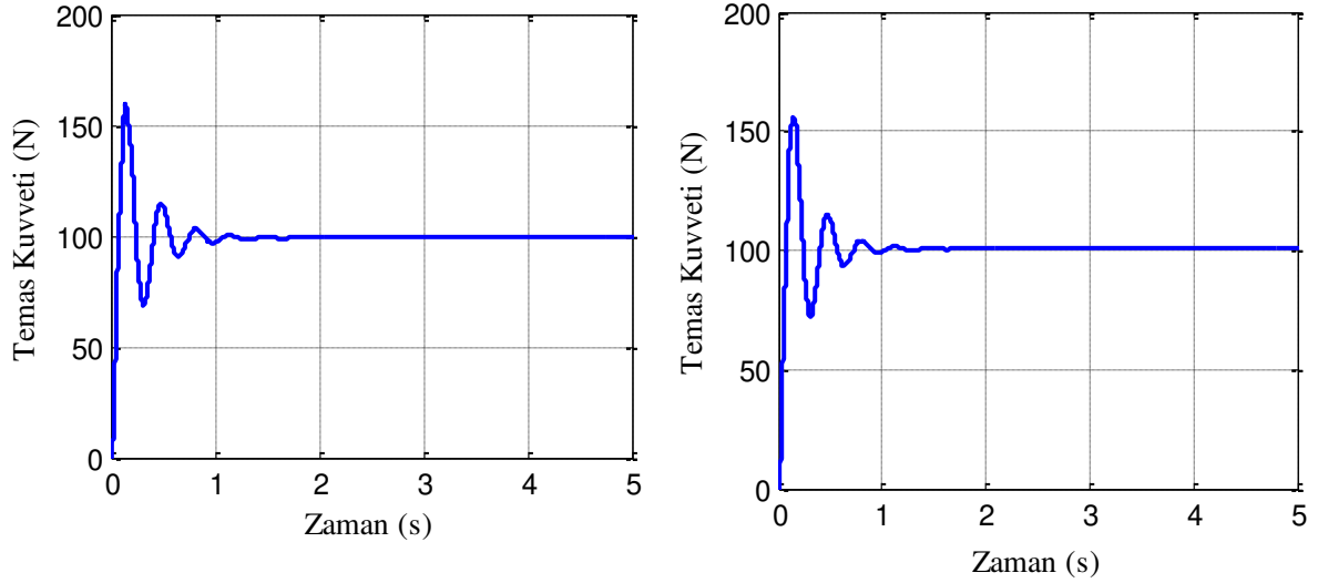
Şekil 3. 14. Farklı pantograf yay sabiti ( k_{pan} ) değeri için temas kuvveti değişimi
