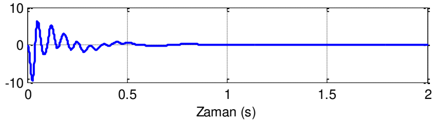
(c) Referans ve en düşük tepe kütesi değerleri için temas kuvvetleri farkı
