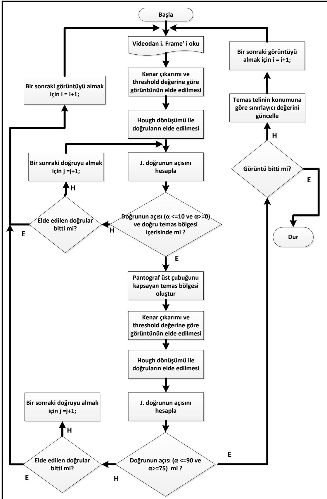
Şekil 5.15. Önerilen yöntemin akış şeması
