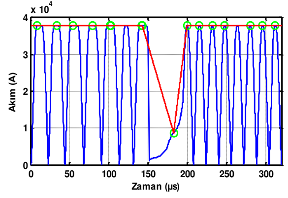
(b) Arızalı akım sinyali
