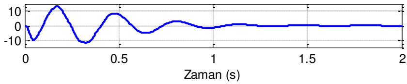
(b) Referans ve en yüksek pantograf tepe sönümleme katsayısı değerleri için temas kuvvetleri farkı
