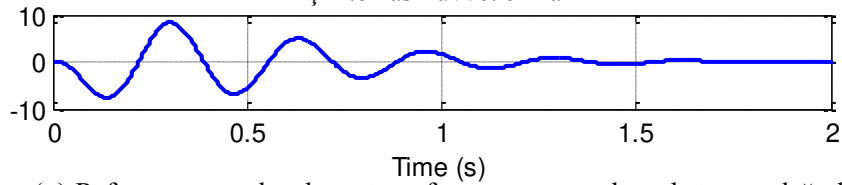
Şekil 3.21. Farklı pantograf çerçeve sönümleme katsayısı ( c_{\text{ç}} ) değeri için temas kuvvetlerinin karşılaştırılması
