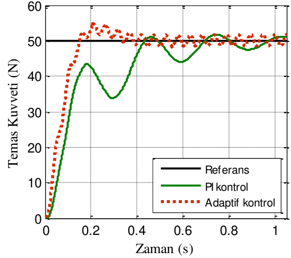
(b) 50 N'luk referans kuvveti için temas kuvveti değişimi
