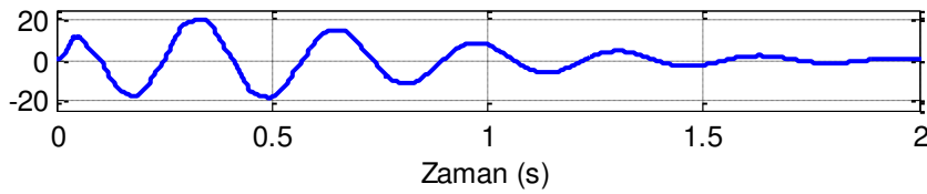
(c) Referans ve en düşük pantograf tepe sönümleme katsayısı değerleri için temas kuvvetleri farkı
