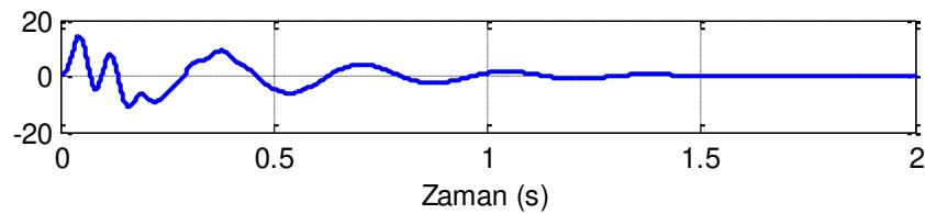
Şekil 3. 15. Farklı pantograf yay sabiti ( k_{pan} ) değeri için temas kuvvetlerinin karşılaştırılması
