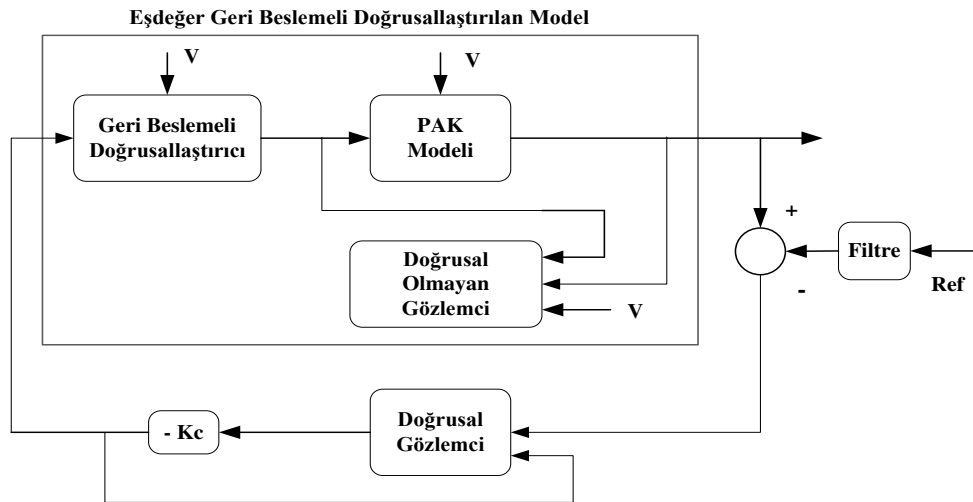
Şekil 1.2. Kontrol sisteminin blok diyagramı [11].
