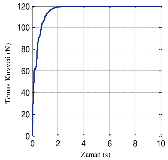
(b) 120 N'luk referans kuvveti için temas kuvveti değişimi
