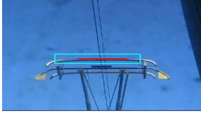
Şekil 4.23. Gerçek görüntü üzerinde sınırlayıcı alan ve pantograf üst çizgisi
