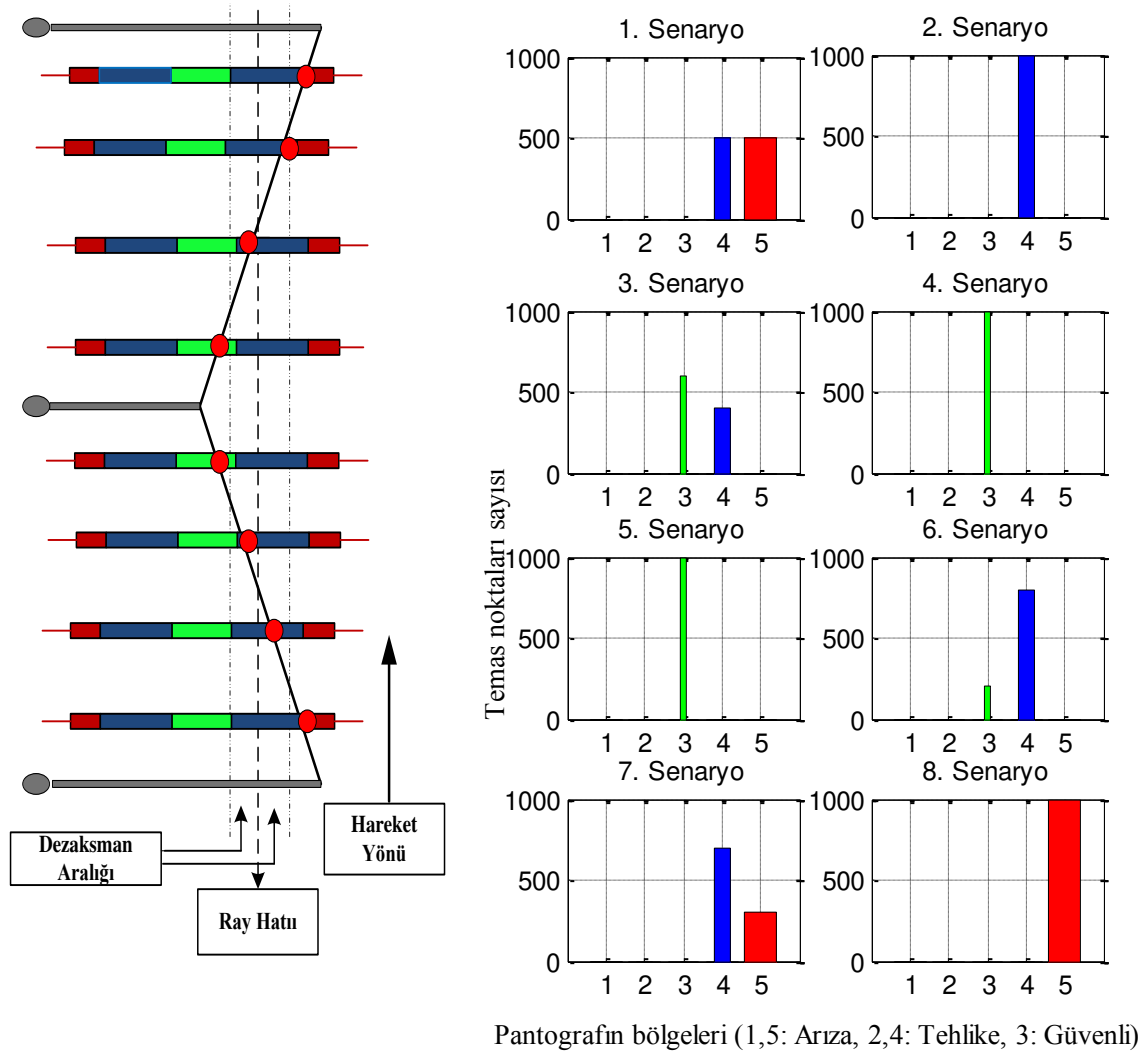
a) Temas noktası değişimi
