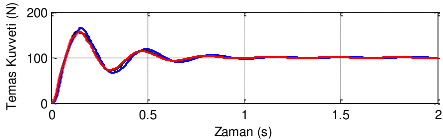
Şekil 3. 14. Farklı pantograf yay sabiti ( k_{pan} ) değeri için temas kuvveti değişimi
