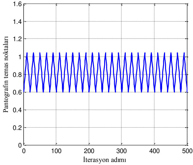
Şekil 5.7. 200 km/sa hız değeri için temas noktası değişimi
