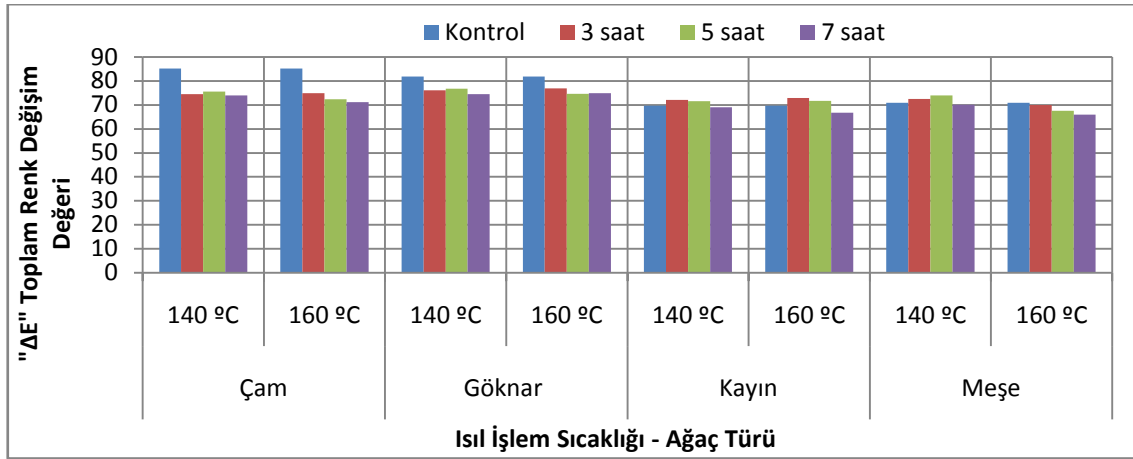
Şekil 3.58. Ağaç türü, ısıtım sıcaklığı ve ısıtım süresine ait karşılaştırma sonuçları.
