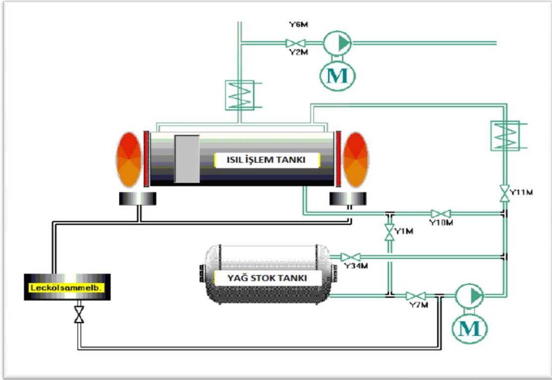
Şekil 1.13. Sıcak yağ uygulaması gerçekleştiren ısıtım fırının temel tasarım planı (Rapp ve Sailer 2000).
