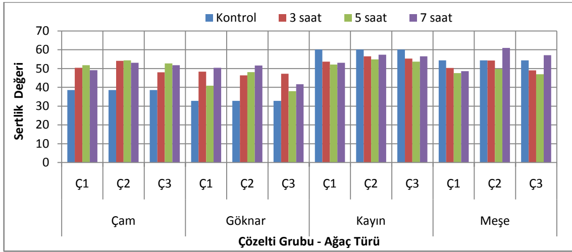
Şekil 3.87. Ağaç türü – Çözeltili grubu – Isıl işlem süresine ait karşılaştırma sonuçları.
