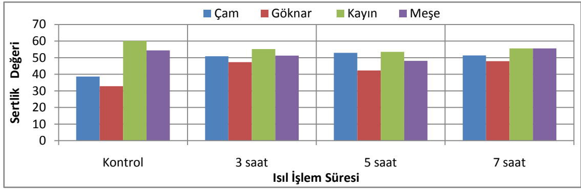
Şekil 3.83. Ağaç türü – Isıl işlem süresine ait karşılaştırma sonucu.
