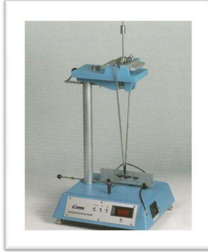
Şekil 1.23. Pandüllü sertlik ölçme cihazı (BYK Gardner).
