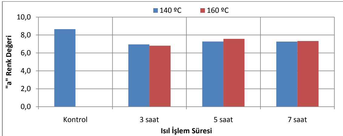
Şekil 3.10. Isıl işlem sıcaklığı – Isıl işlem süresine ait karşılaştırma sonuçları.
