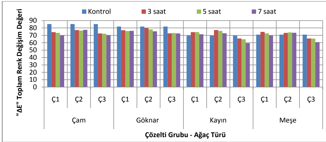
Şekil 3.57. Ağaç türü – Çözelti grubu – Isıl işlem süresine ait karşılaştırma sonuçları.
