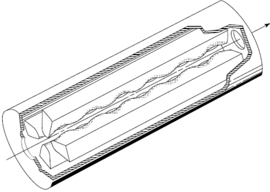
Şekil 2.6 RFQ yapısı [33]
