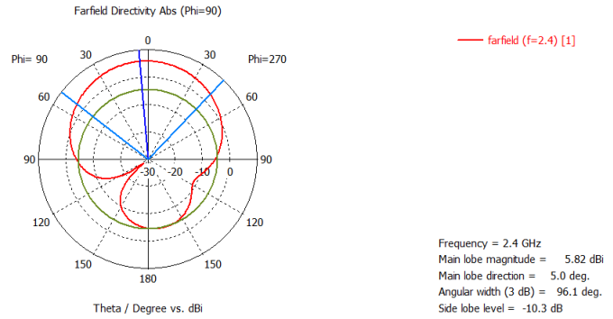
Şekil 7.16. Tasarlanan ikinci antenin tek boyutlu yönlülük grafiği
