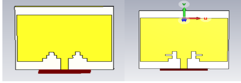
Şekil 4.2. Tasarlanan mikroşerit yama anten şekilleri
