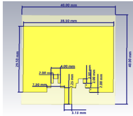
Şekil 7.47. Tasarlanan ve üretimi yapılan mikroşerit yama anten modeli (6. anten)
