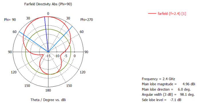
Şekil 7.25. Tasarlanan üçüncü antenin tek boyutlu yönlülük grafiği
