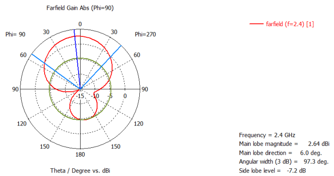
Şekil 7.32. Tasarlanan dördüncü antenin tek boyutlu kazanç grafiğı
