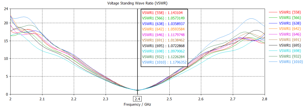
Şekil 7.31. Tasarlanan dördüncü antenin VSWR grafikleri
