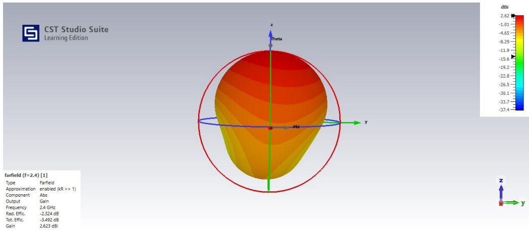
Şekil 7.46. Tasarlanan beşinci antenin üç boyutlu kazanç grafiği
