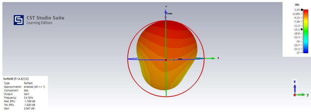
Şekil 7.10. Tasarlanan ilk antenin üç boyutlu kazanç grafiği
