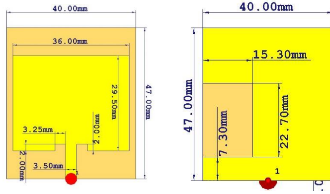
Şekil 7.66. Tasarlanan ve üretilen sekizinci çift bant (dual bant) antenin ön ve arka yüz modeli
