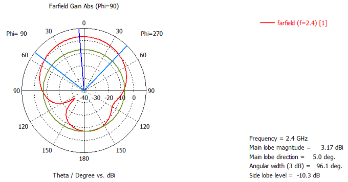
Şekil 7.14. Tasarlanan ikinci antenin tek boyutlu kazanç grafiği
