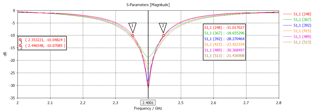
Şekil 7.49. Tasarlanan altıncı antenin S_{11} grafikleri
