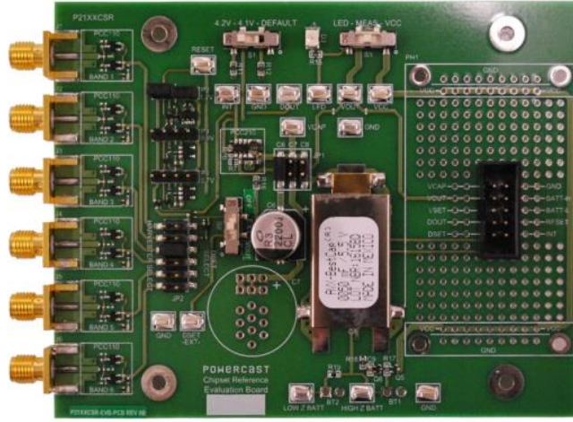
Şekil 7.1 P21XXCSR-EVB Enerji hasatlama modülü
