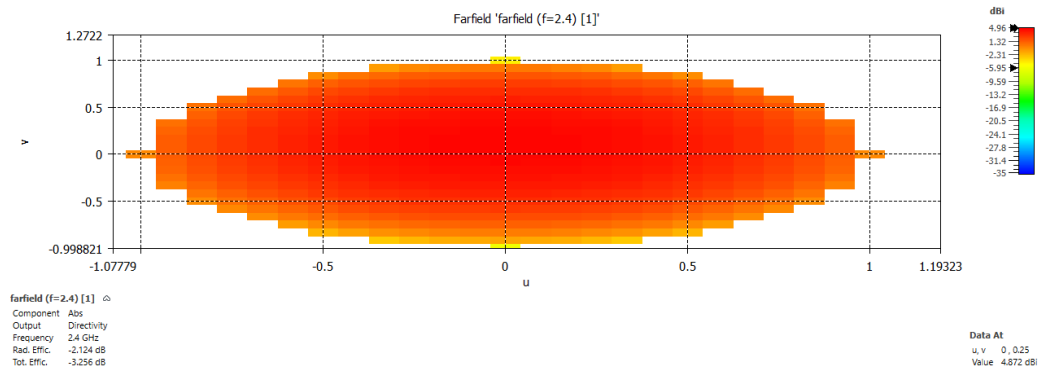
Şekil 7.26. Tasarlanan üçüncü antenin iki boyutlu yönlülük grafiği
