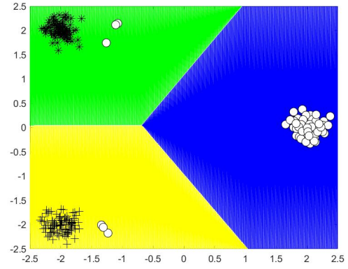
(b) CVaR CS-MSVM, 0.33 class 1 probability
