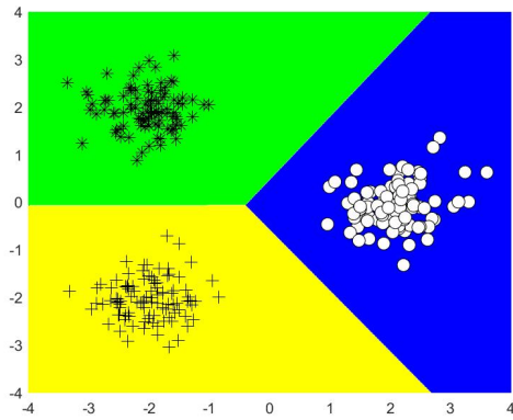
(a) CS-MSVM, 0.1 class 1 probability
