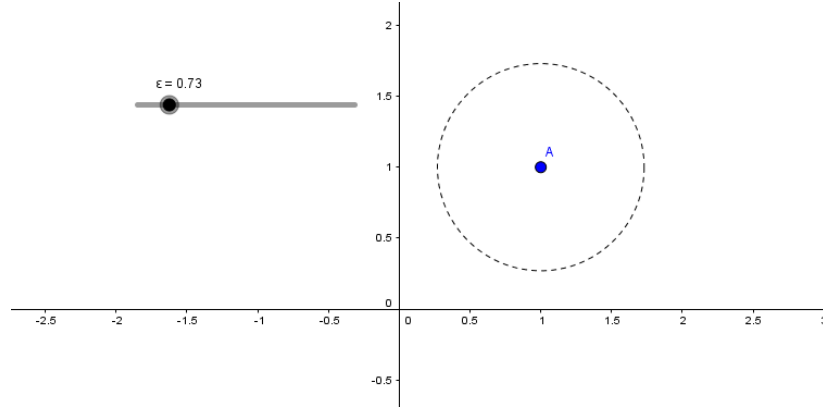
Şekil 2.3. \mathbb{R}^2 kümesi için açık yuvar gösterimi
