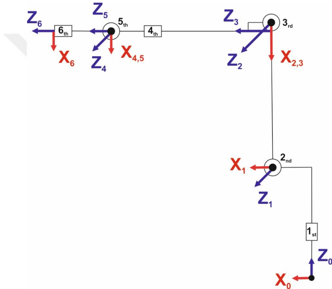
Figure 2-6: Kuka Kr240 R2900 DH frames
