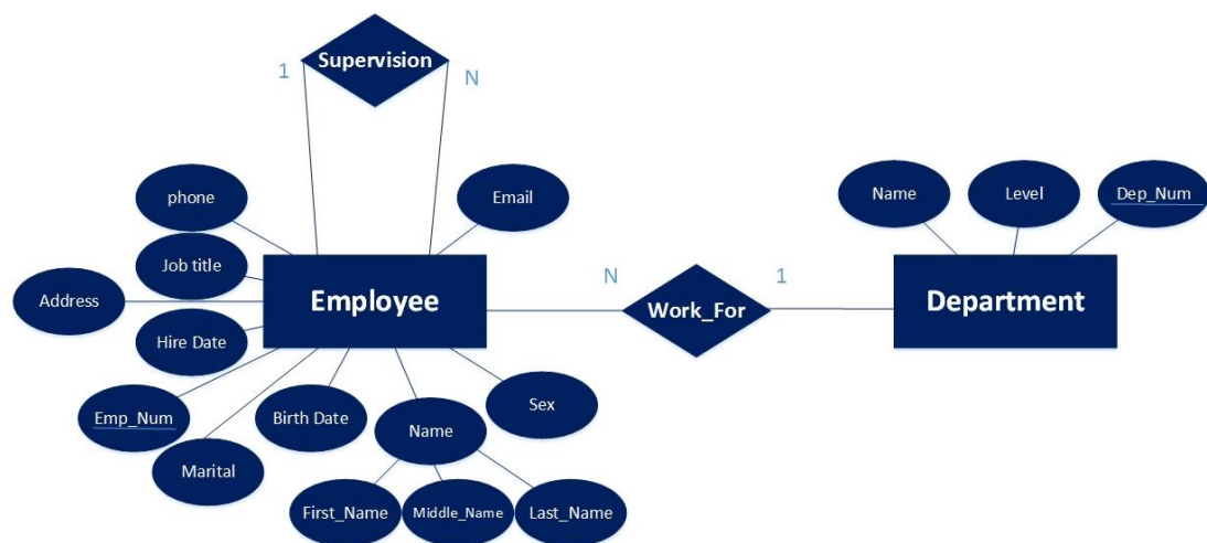
Figure 8 ER diagram
