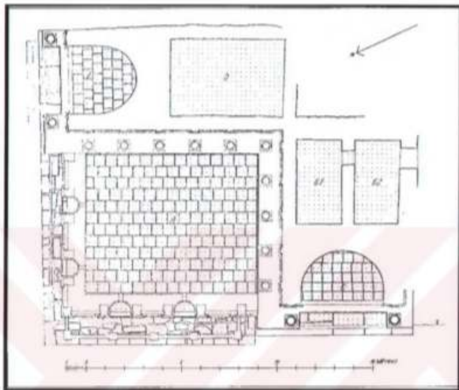
Resim 23: Nymphaion planı.(Laodiceia)
