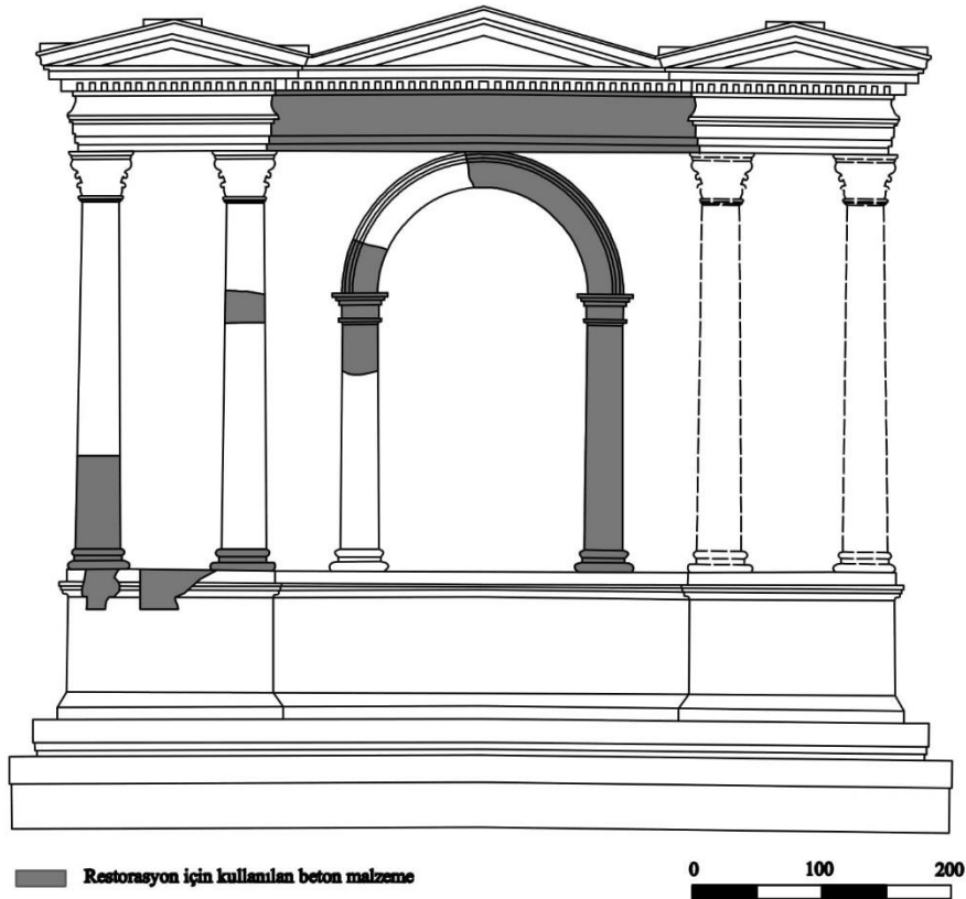
Görsel 63: Vespasianus Anıtı Cephe Çizimi ve Restorasyonda Beton Malzemenin Kullanıldığı Kısımlar
