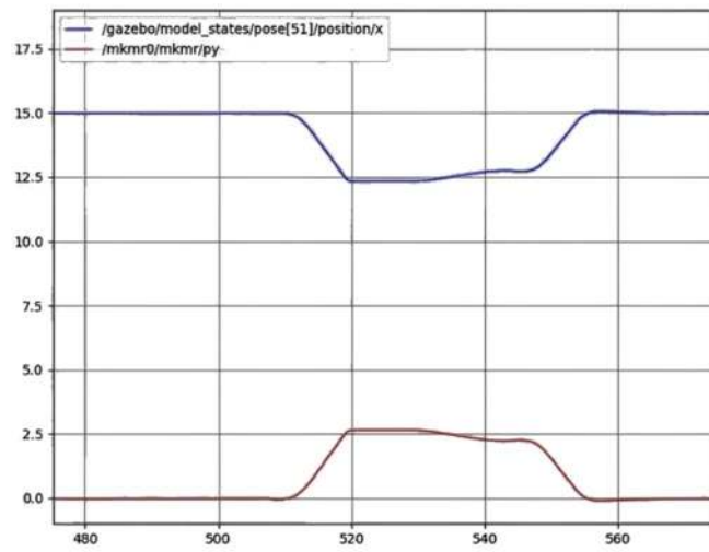
Şekil 5.19 : Simülasyon (x) ve navigasyon (y) eksenindeki değişim grafiği
