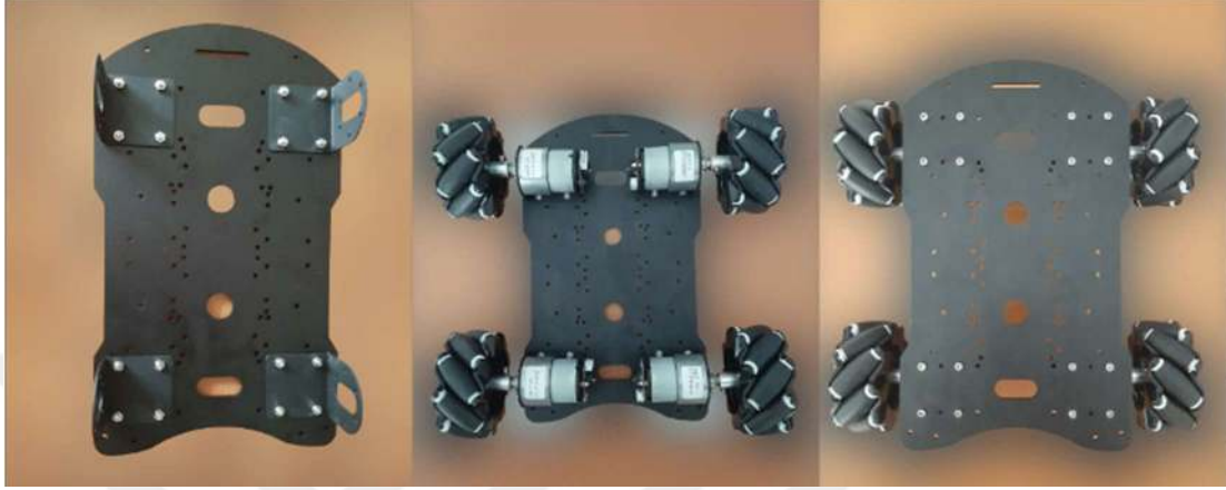
Şekil 2.6 : Montaj görüntüleri.
