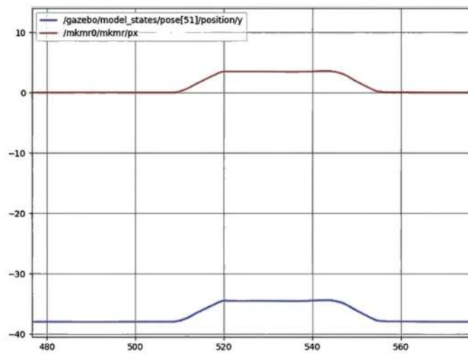
Şekil 5.20 : Simülasyon (y) ve navigasyon (x) eksenindeki değişim grafiği
