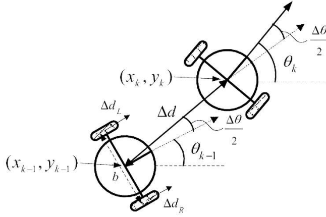
Şekil 2.8 : Odometri Verisi [27].
