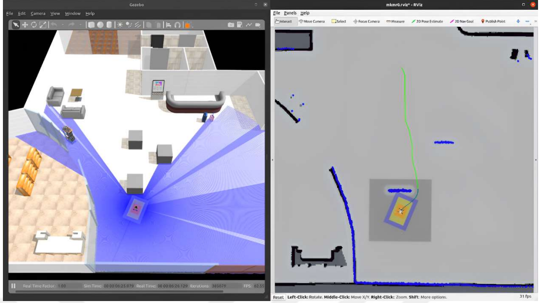
Şekil 4.11 : Navigasyon çalıştırılması.
