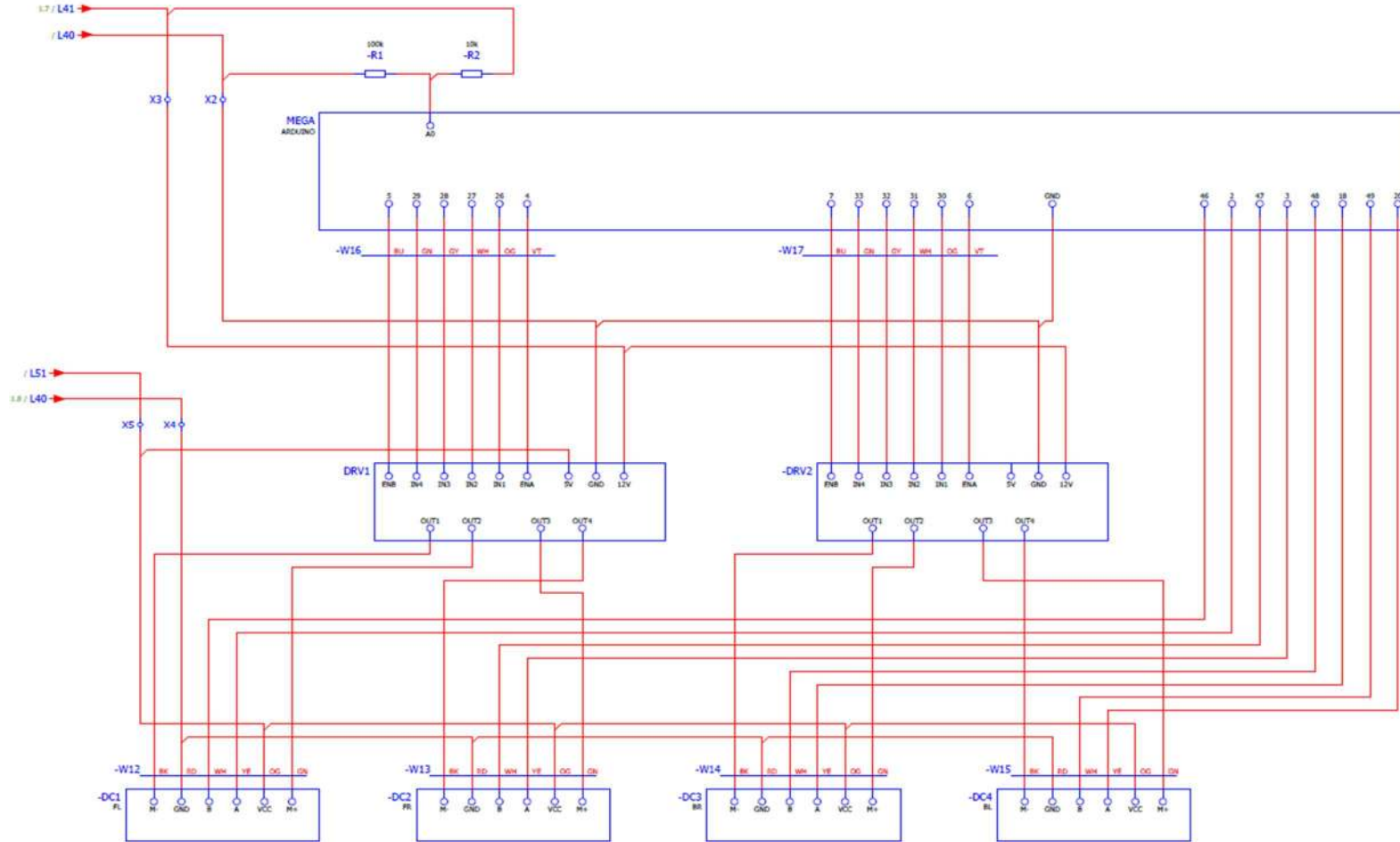
Şekil A.2 : Mikrodenetleyici ve motor sürücü elektrik şeması.
