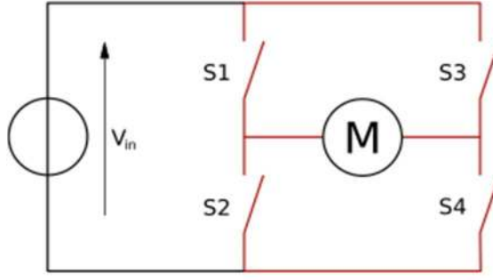
Şekil 2.9 : Motor sürücü H köprüsü [29].
