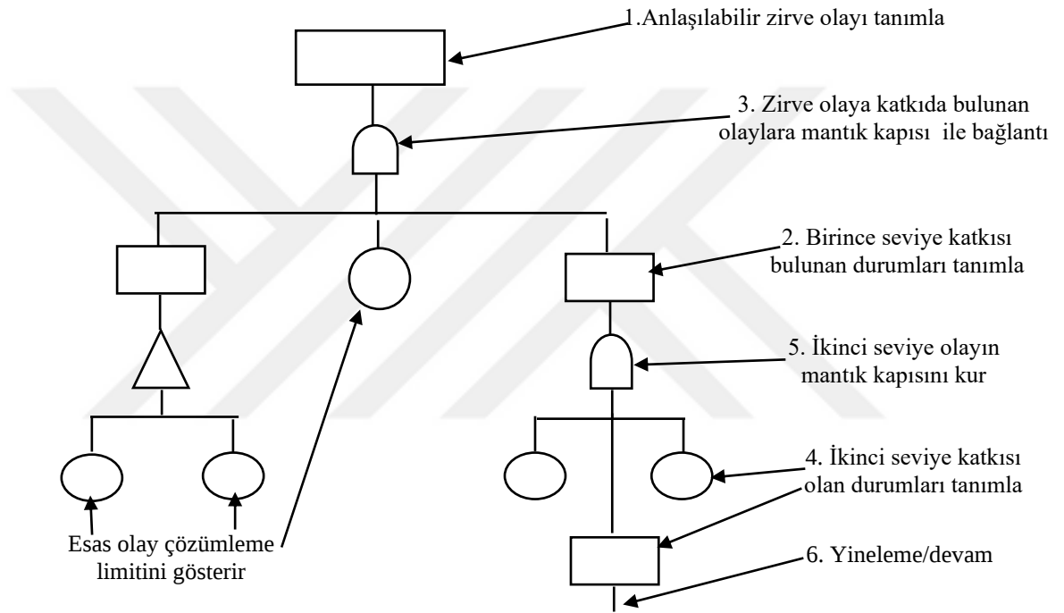
Şekil 1.2. Hata Ağacı Analiz Şeması (Koru, 2006)
