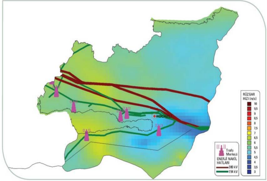
Şekil 3.22. Trafo merkezi ve enerji nakil hatları [62]
