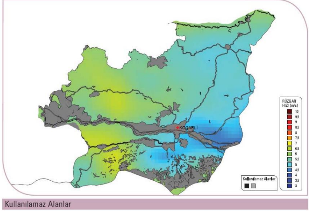
Şekil 3.21. Rüzgâr enerjisi santrali kullanılabilir alanlar [62]
