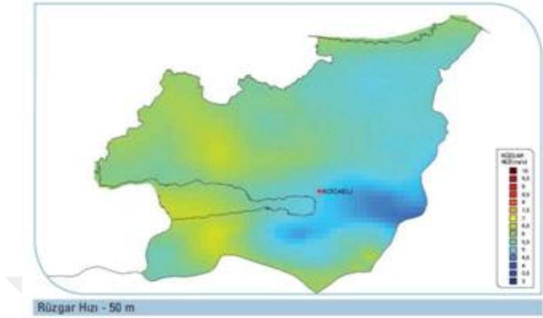
Şekil 3.19. Kocaeli ili rüzgâr hızı dağılımı 50 m [62]
