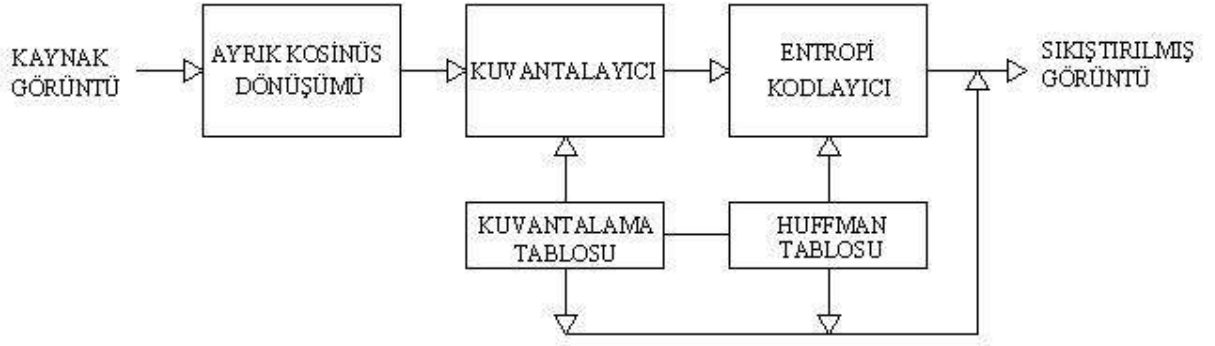
Şekil 3.2 JPEG kodlayıcı blok yapısı
