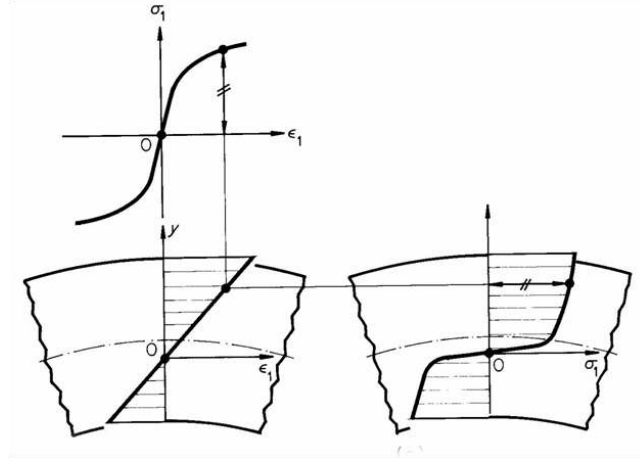
Şekil 2.22. Bükmedeki gerilme - gerinme dağılımı (Marciniak ve Duncan, 1992)
