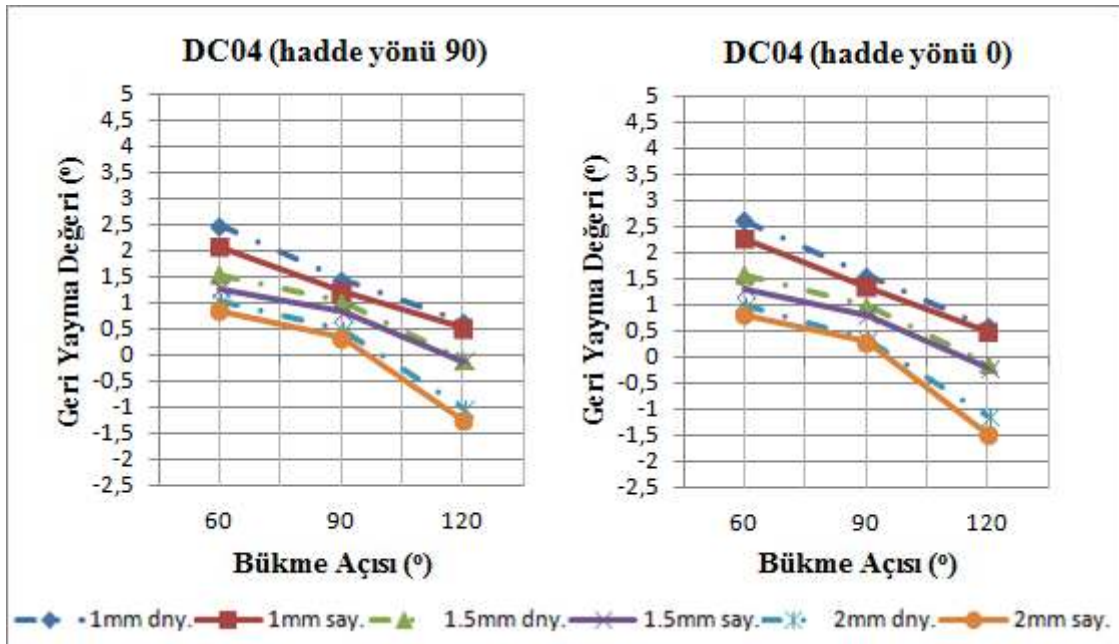
Şekil 4.4. DC04 sacının geri yaylanma grafiği
