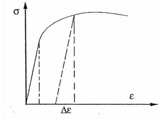
Şekil 2.27. Sünek bir metaldeki geri esnemenin akma diyagramı üzerinde gösterilişi (Arslan, 2007)
