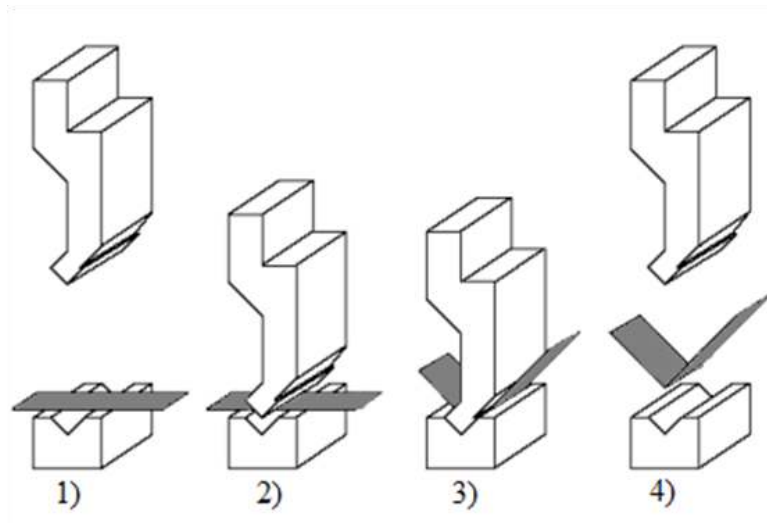
Şekil 2.14. V bükme işleminin safhaları (Kılıç, 2009)
