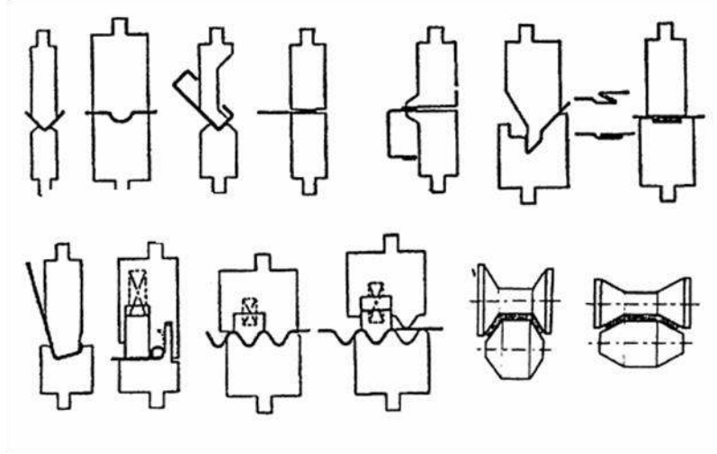
Şekil 2.13. Çeşitli sac bükme işlemleri (Tekiner, 2004)
