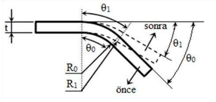
Şekil 2.28. Bükme işlemi sonrasında oluşan geri yaylanma (Garcia- Romeu vd., 2007)
