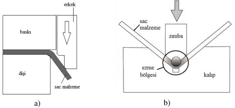
Şekil 2.17. a) Çift etkili bükme işlemi, b) Ezerek bükme işlemi (URL-1, 2013)
