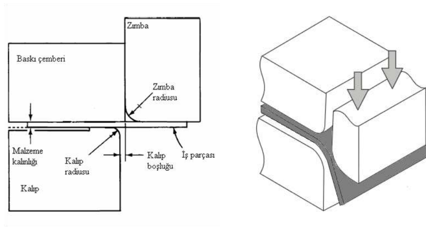
Şekil 2.16. Kenar bükme işlemi (Ling vd.,2005; URL-1, 2013)
