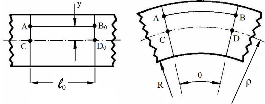
Şekil 2.25. AB yayının bükme sonrası oluşan deformasyonu (Kılıç, 2009)
