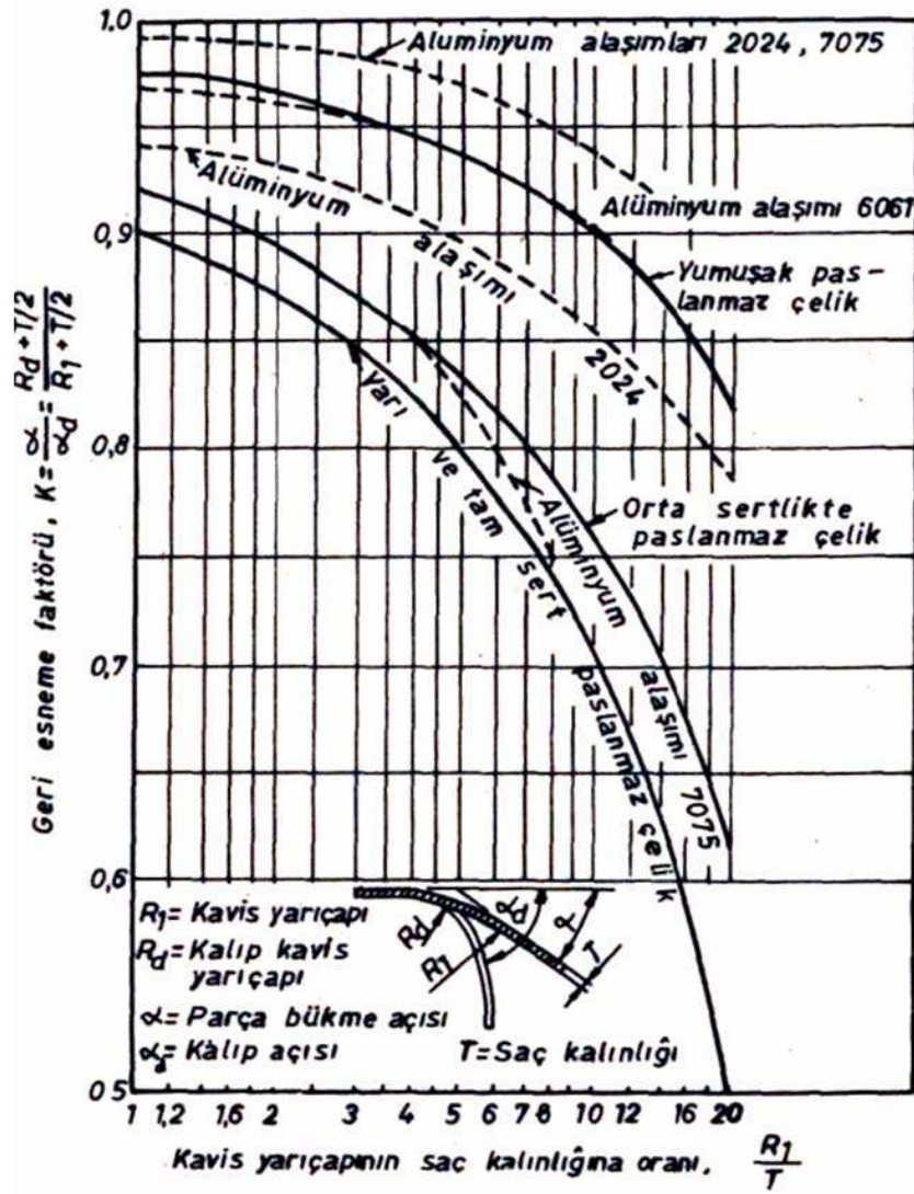
Şekil 2.29. R/t oranı ile geri yaylanma faktörü arasındaki bağıntı (URL-3, 2013)
