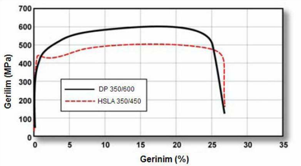
Şekil 2.4. DP ve HSLA çelik saclarının gerilim - gerinim grafikleri (AHSS Application Guidelines, 2005)
