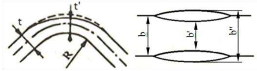
Şekil 2.23. Bükme işlemindeki sac kalınlığı ile parça eninin değişmesi (Çapan, 2003)
