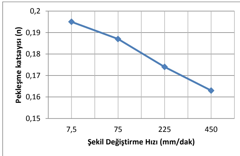
Şekil 5.8 DP780 şekil değiştirme hızı – pekleşme katsayısı değişim grafiği
