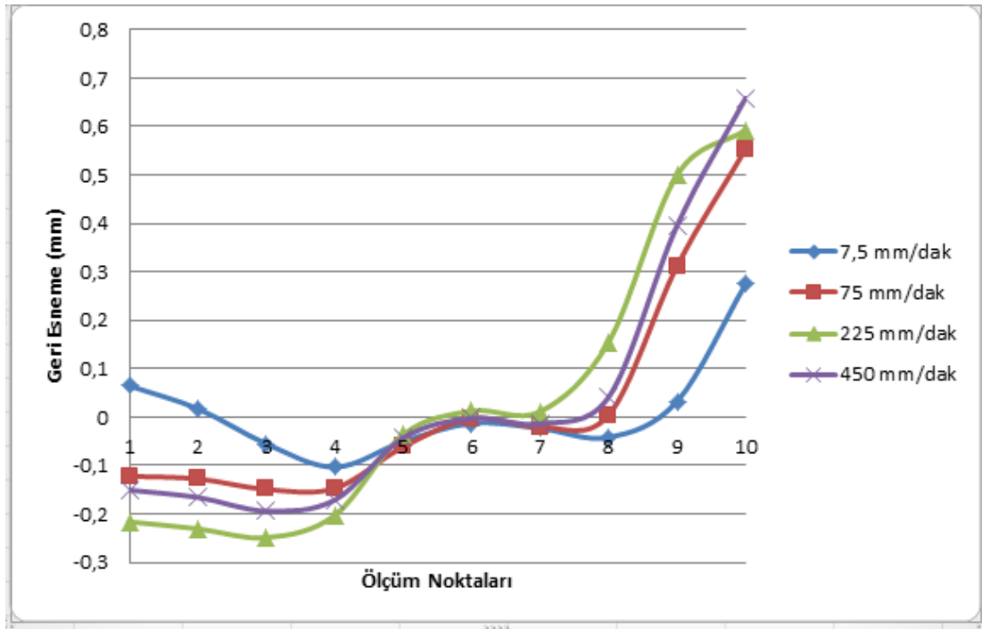
Şekil 5.22. DP780 şekil değıştirme hızı - geri esneme grafiğı
