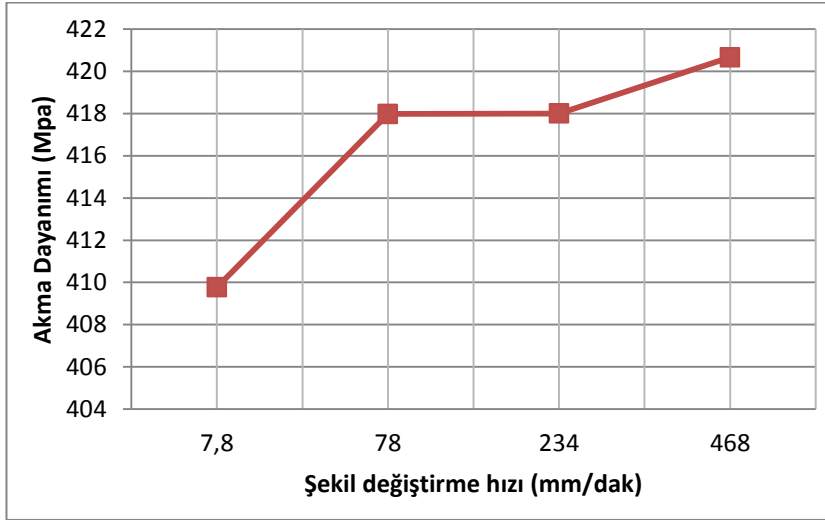
Şekil 5.3 DP600 şekil değiştirme hızı - akma dayanımı grafiği
