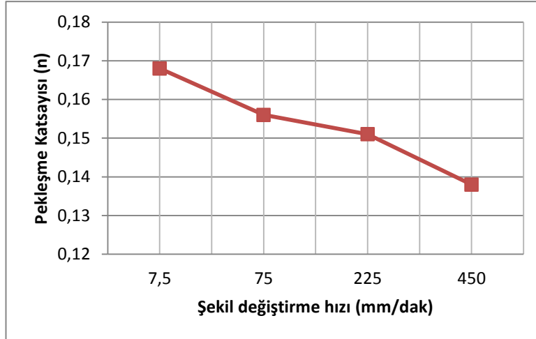
Şekil 5.7 DP600 şekil değiştirme hızı – pekleşme katsayısı değişim grafiği
