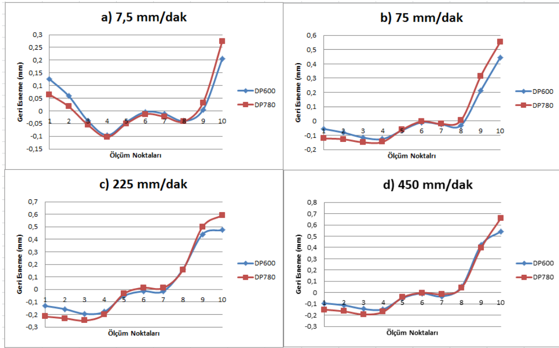
Şekil 5.20. Şekil değiştirme hızı – geri esneme grafikleri
