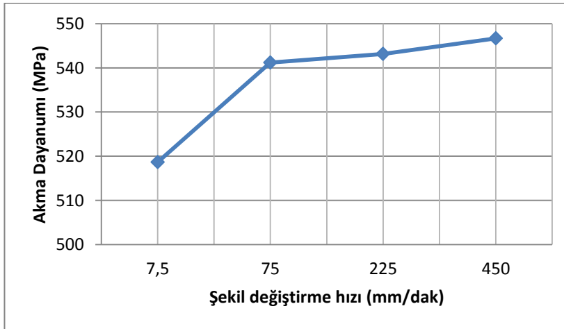
Şekil 5.4 DP780 şekil değiştirme hızı - akma dayanımı grafiği
