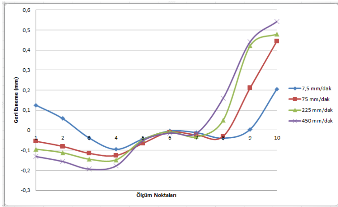
Şekil 5.21. DP600 şekil değiştirme hızı – geri esneme grafiği
