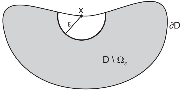
Şekil 5.4. x \in \partial D için D \setminus \Omega_\epsilon bölgesi
